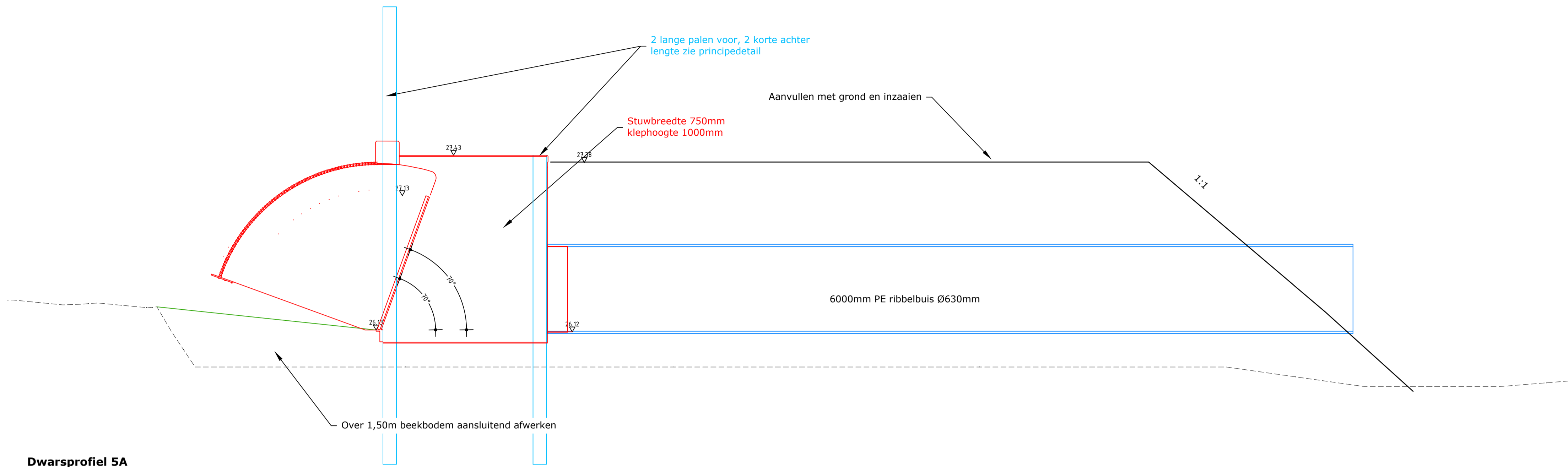
Dwarsprofiel 5A Schaal 1:20
