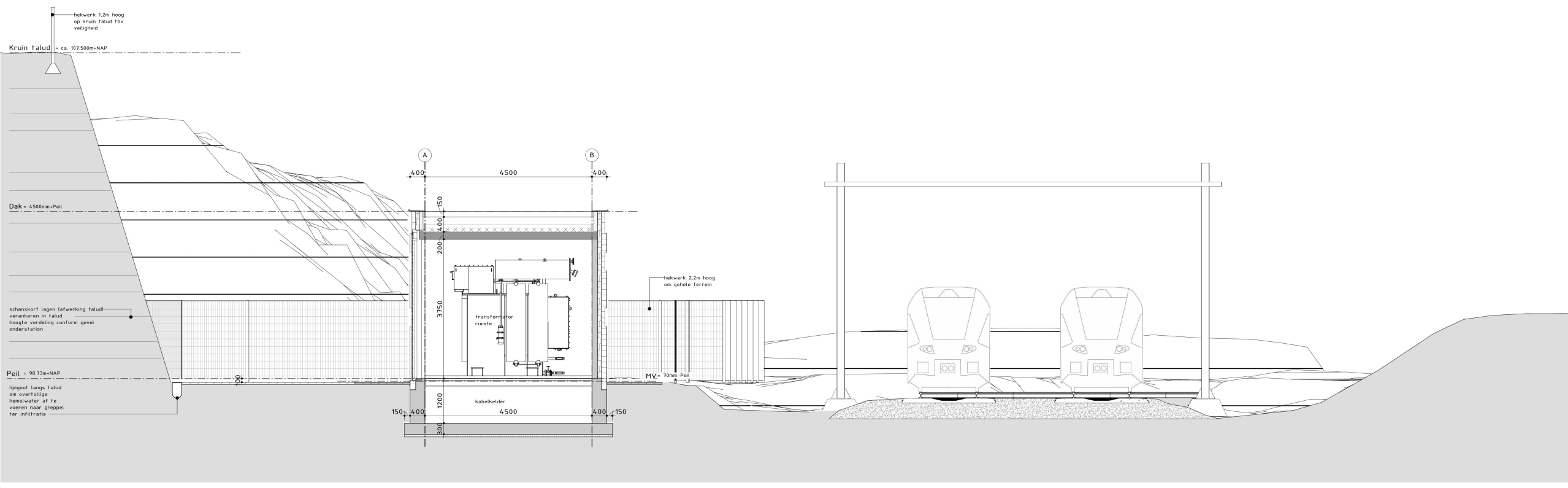
Dwarsprofiel Schaal 1:50
