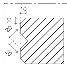
Detail koppelat-sparing
