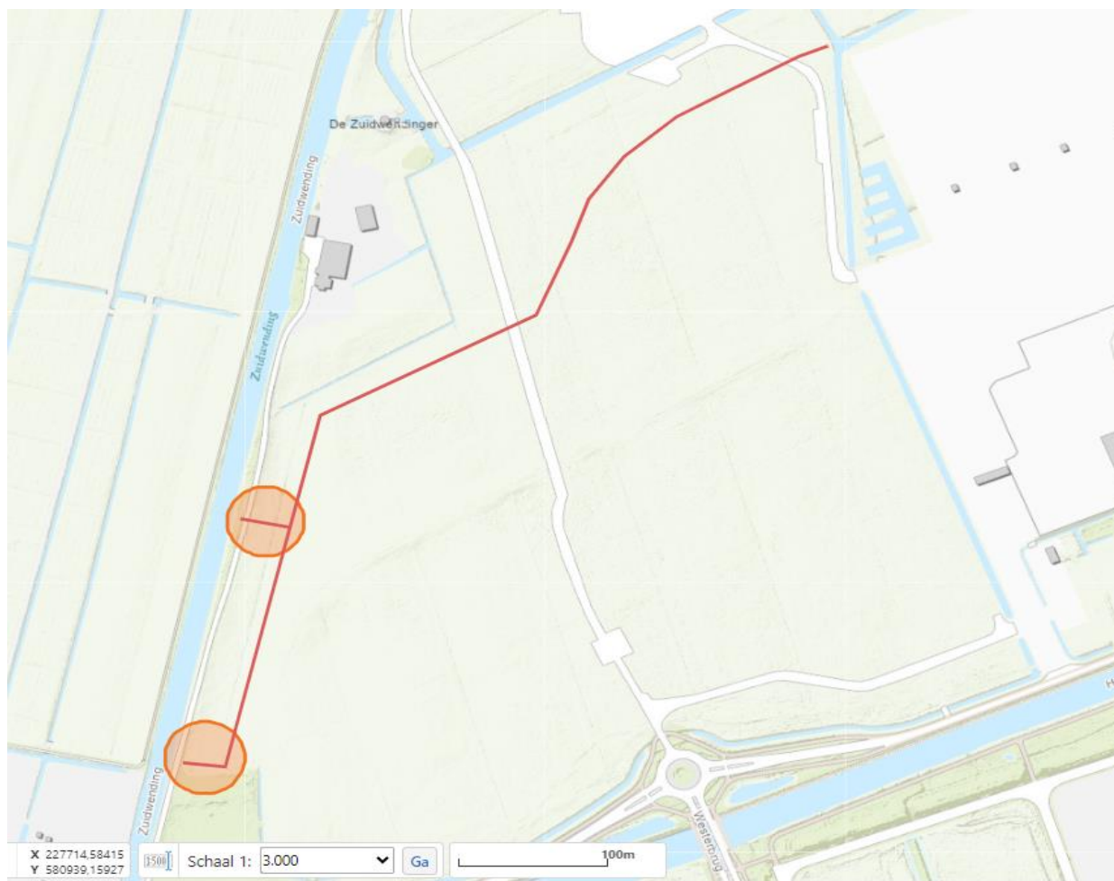
Figuur 1: De rode lijn geeft globaal de locatie weer van de aan te leggen leiding. De vergunningplicht ziet op de activiteit binnen de beperkingengebieden van de regionale waterkering, deze locaties zijn aangegeven met de oranje cirkels.
