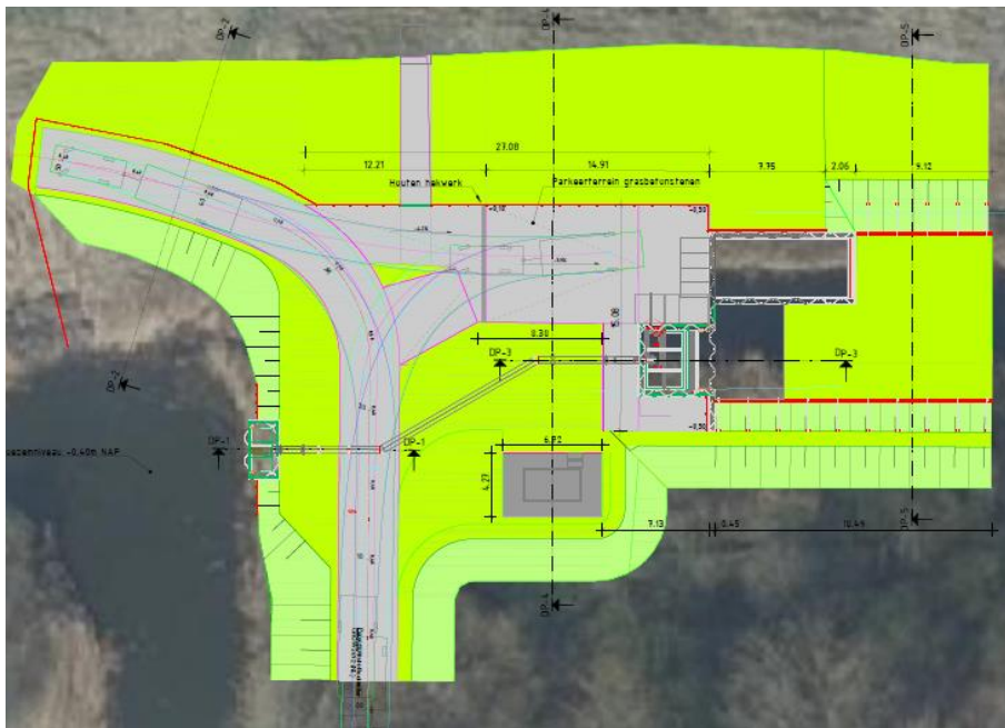
Figuur 2 bovenaanzicht gemaal met maatvoering
