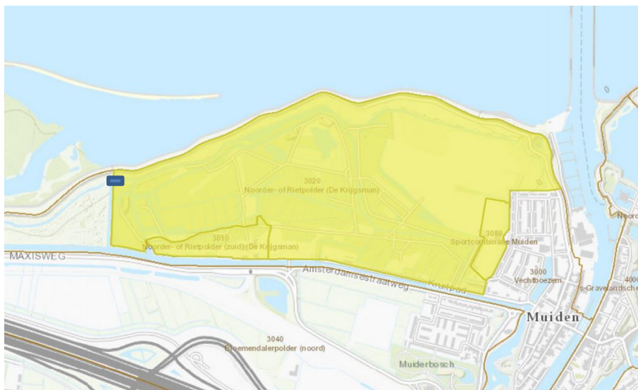
Figuur 1 Ligging Noorder- of Rietpolder met locatie van het te realiseren gemaal
