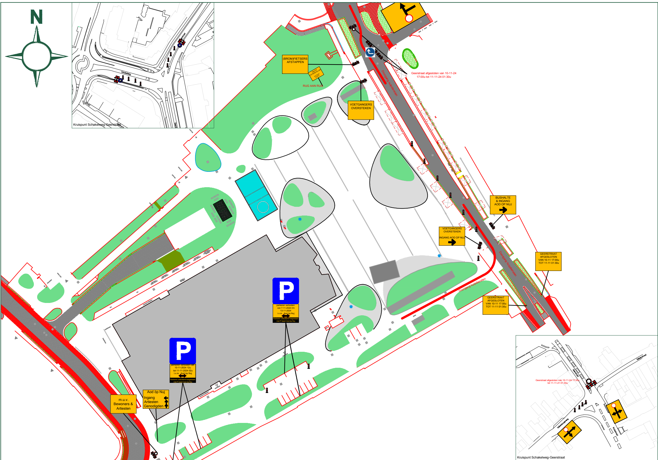
Kruispunt Schakelweg-Geerstraat
