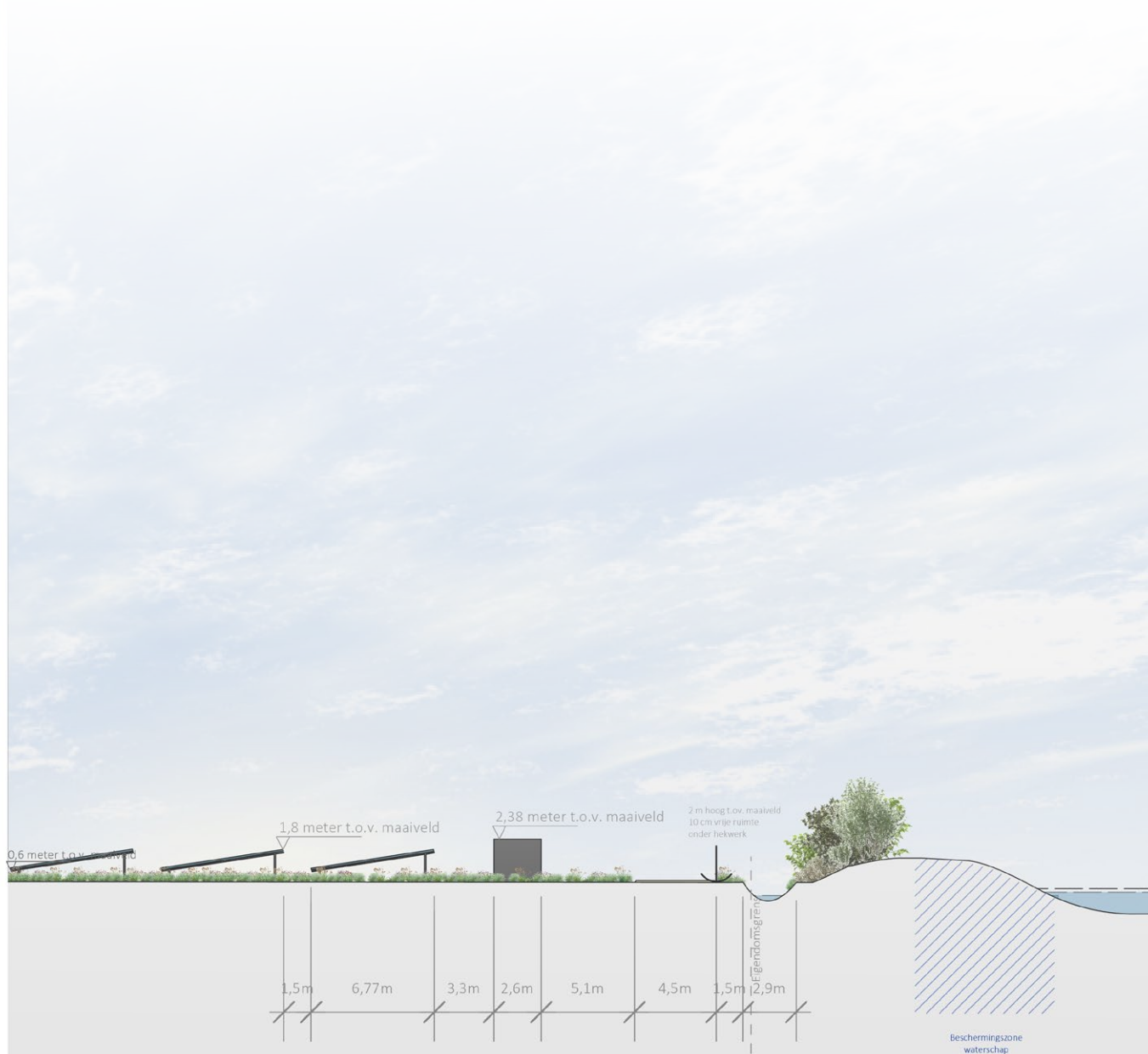
Afbeelding 14. Doorsnede E van de noordelijke grens van zonneveld Kanaaldijk-zuid met transformator
