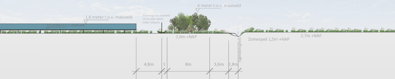
Afbeelding 10. Doorsnede C van de ecologische oever en de losse landschappelijke haag als oostelijke grens van zonneveld Kanaaldijk-Zuid.
