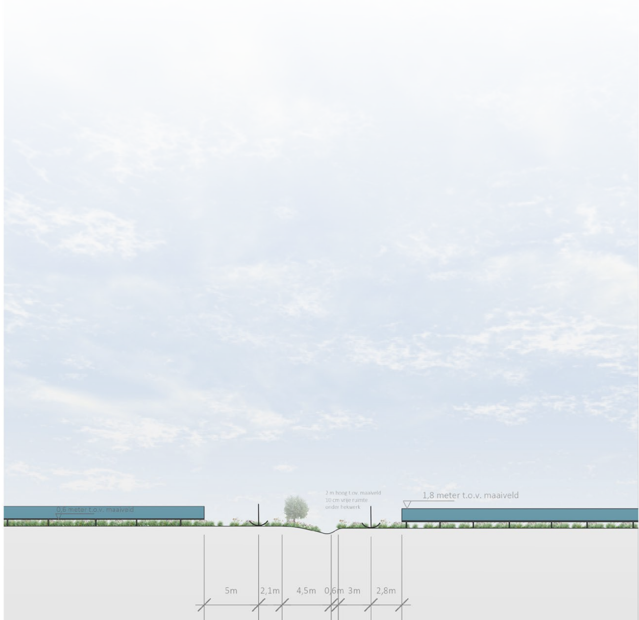
Afbeelding 17. Doorsnede G van de middelste watergang met ecologische oever van zonneveld Kanaaldijk-Zuid.
