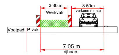
Dwarsdoorsnede B B
