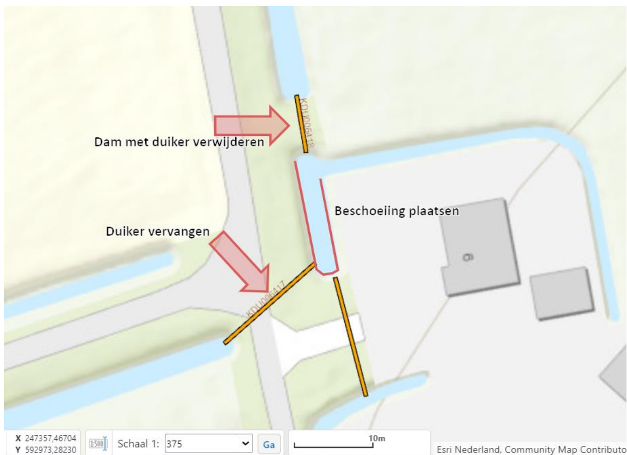
Figuur 1: Overzichtskartaal van de werkzaamheden. De rode lijn geeft de aan te leggen beschoeiing weer.
