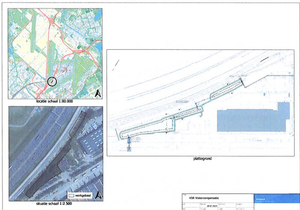
Figuur 2. Watercompensatie.
