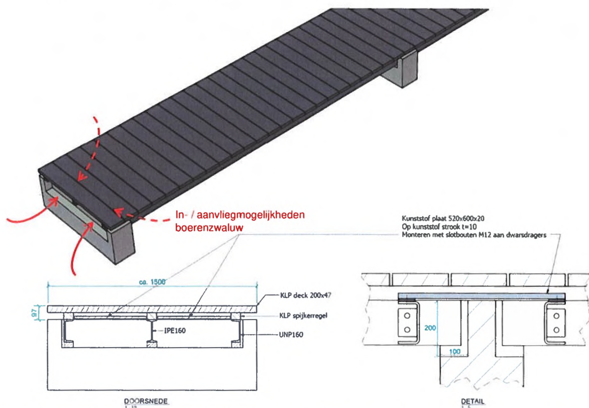
Figuur 1: Methode waarmee de jukken geschikt gemaakt worden voor de boerenwaluw om nesten te maken. Boven de uitsparingen waar de oude betondelen zaten wordt een kunststof afdak gemaakt, waardoor de boerenwaluwen zelf nesten tegen de uitsparingen kunnen maken. Dit wordt om en om gedaan, waardoor er bij 60 jukken steeds 4 theoretisch geschikte nestlocaties gerealiseerd worden. Zo worden er dus in totaal 240 permanente alternatieve nestlocaties gecreëerd.
