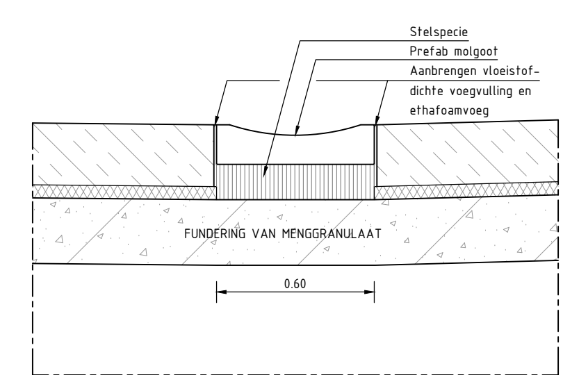
DETAIL D SCHAAL 1:20
