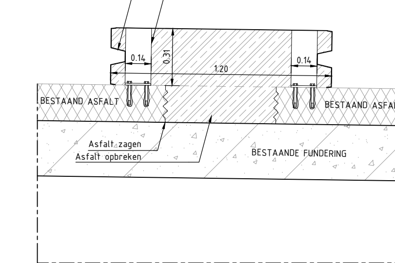
DETAIL F SCHAAL 1:20
