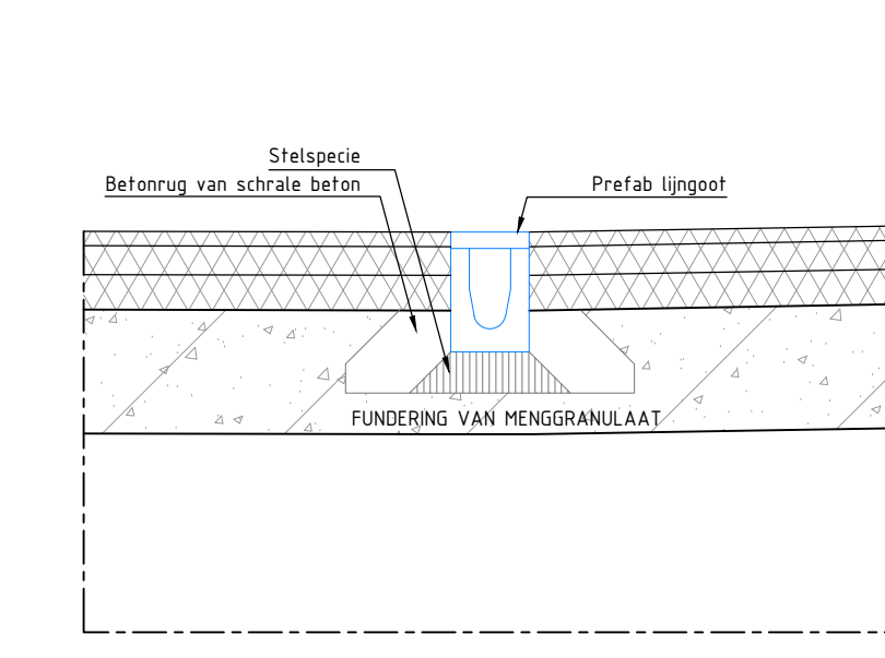
DETAIL C SCHAAL 1:20
