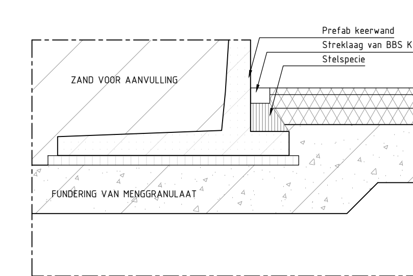
DETAIL E SCHAAL 1:20
