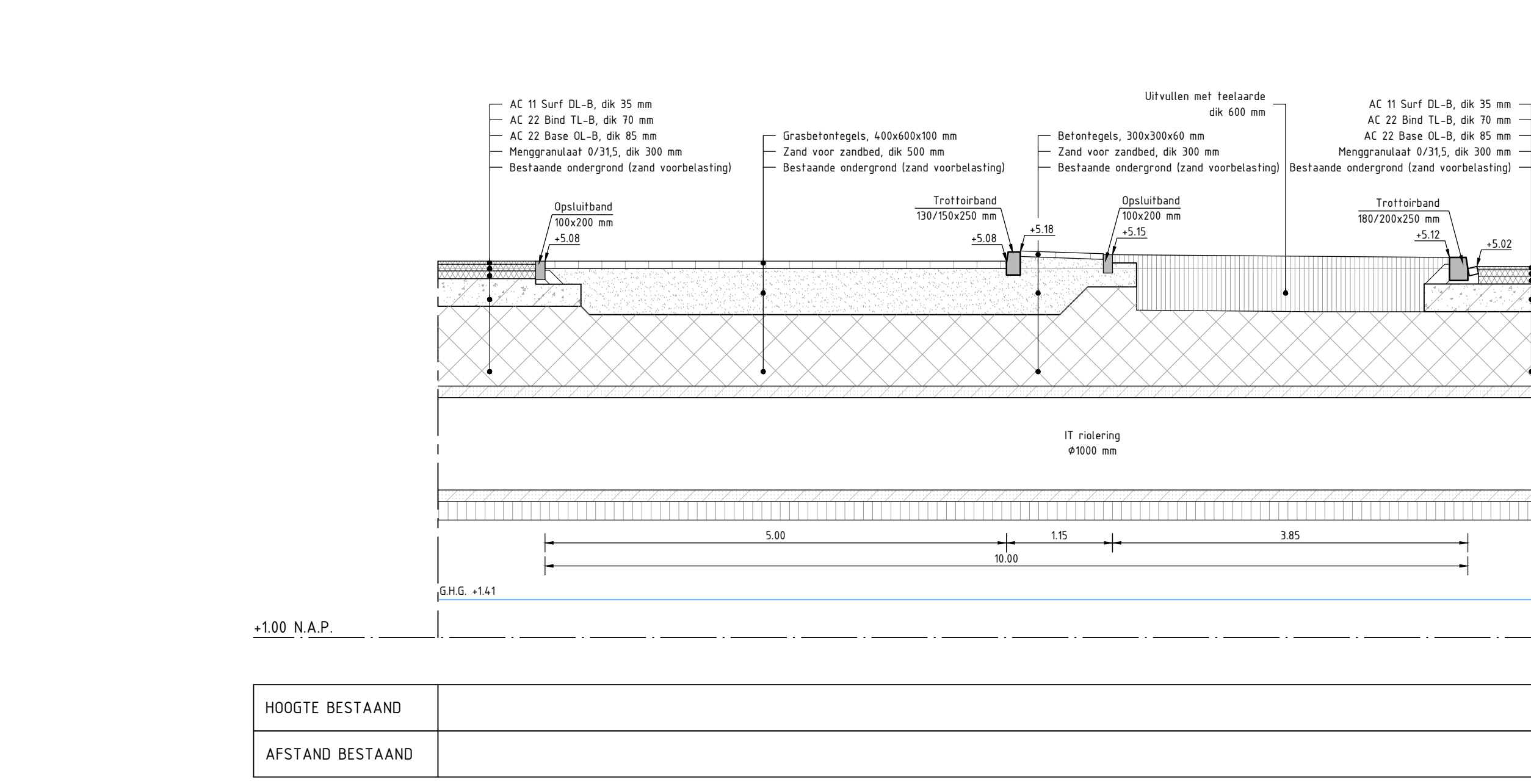
DOORSNEDE 12-12 SCHAAL 1:50
