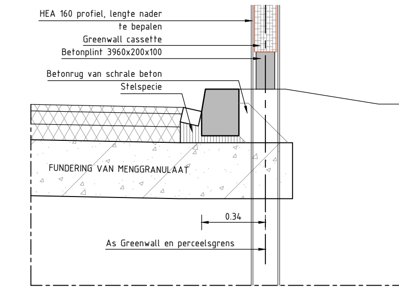
DETAIL B SCHAAL 1:20
