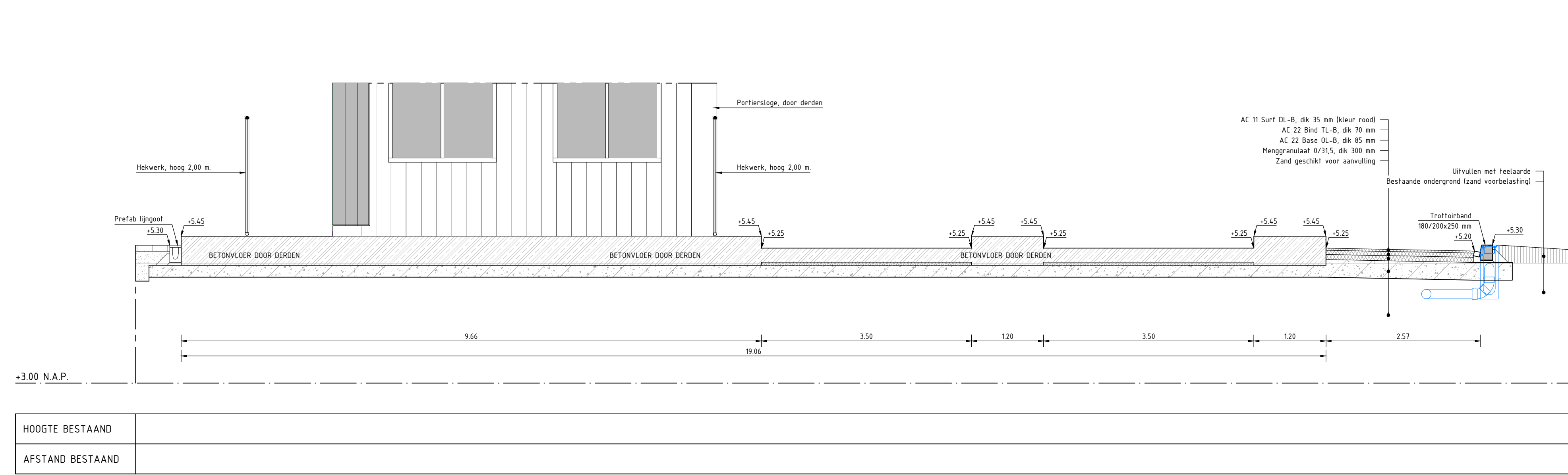
DOORSNEDE 14-14 SCHAAL 1:50
