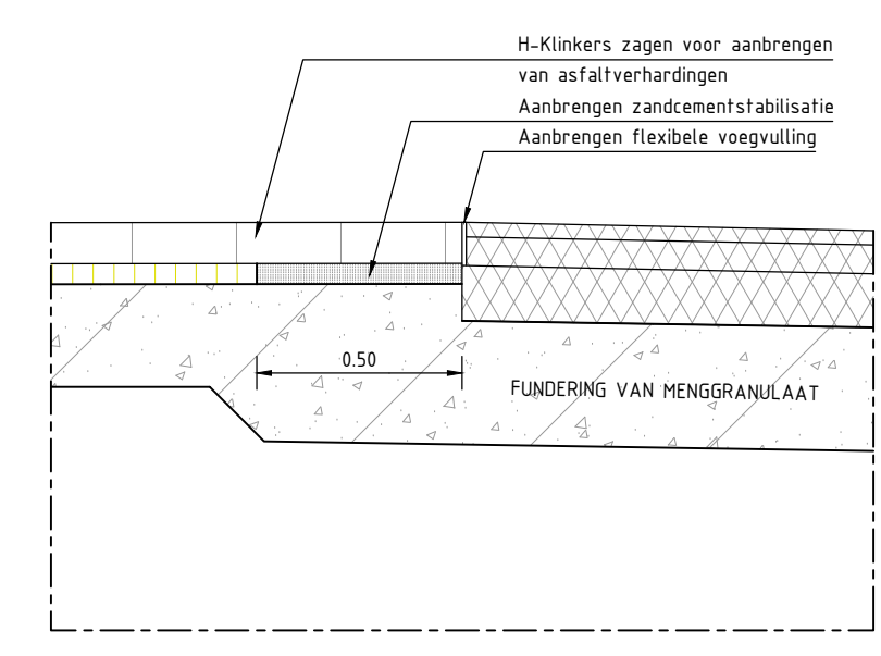
DETAIL A SCHAAL 1:20
