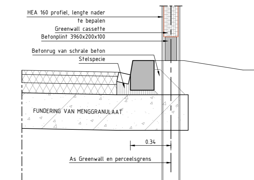
DETAIL B SCHAAL 1:20
