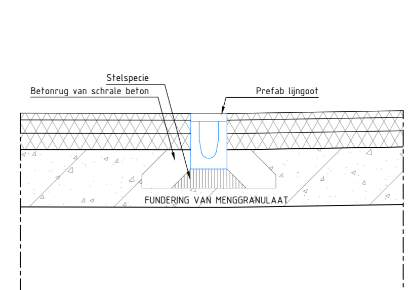
DETAIL C SCHAAL 1:20
