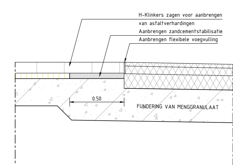
DETAIL A SCHAAL 1:20
