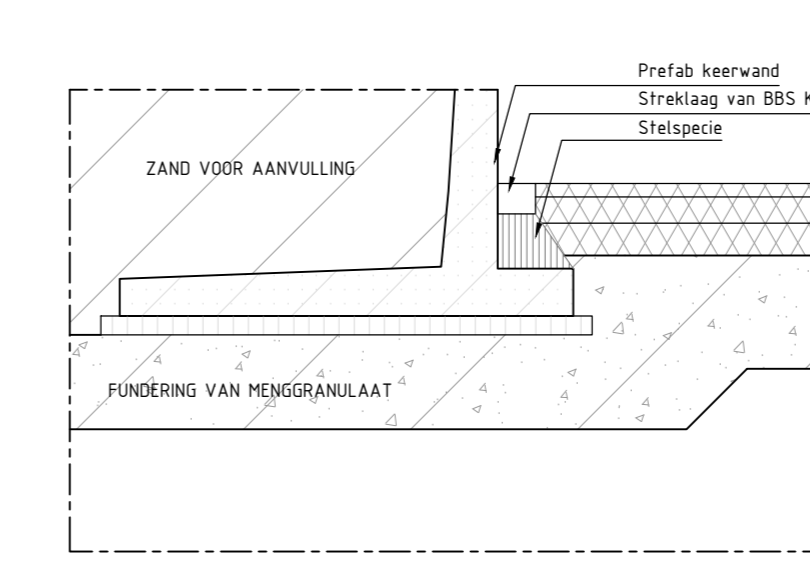
DETAIL E SCHAAL 1:20
