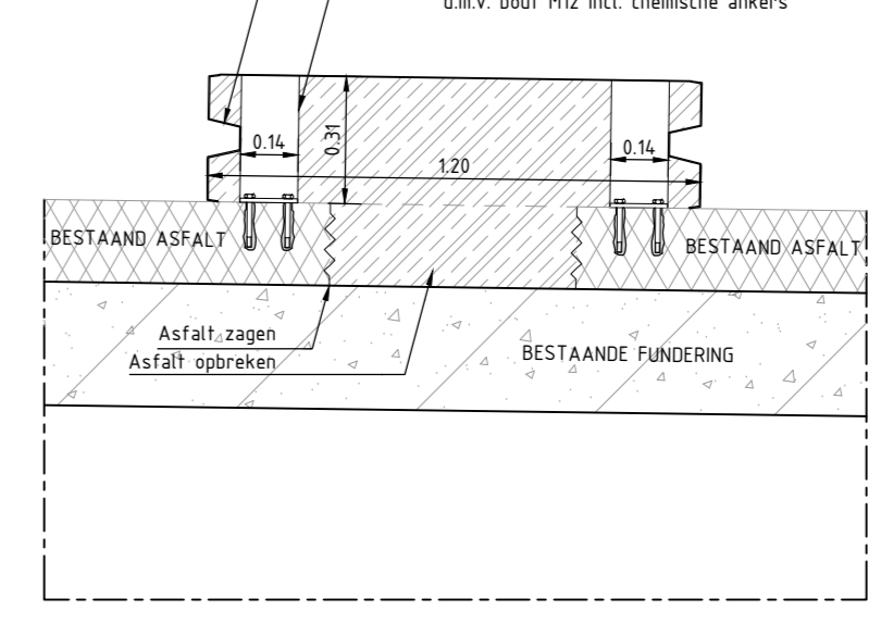
DETAIL F SCHAAL 1:20
