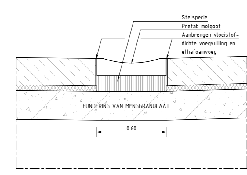
DETAIL D SCHAAL 1:20
