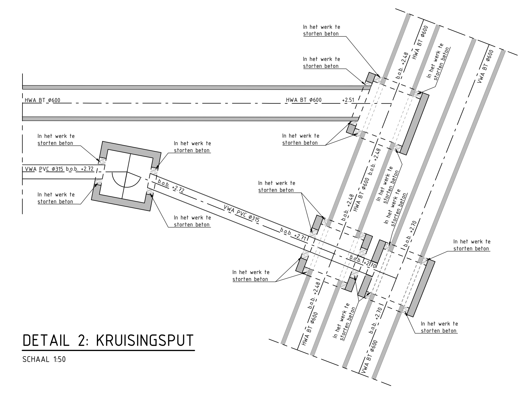
DETAIL 2: KRUISINGSPUT SCHAAL 150
