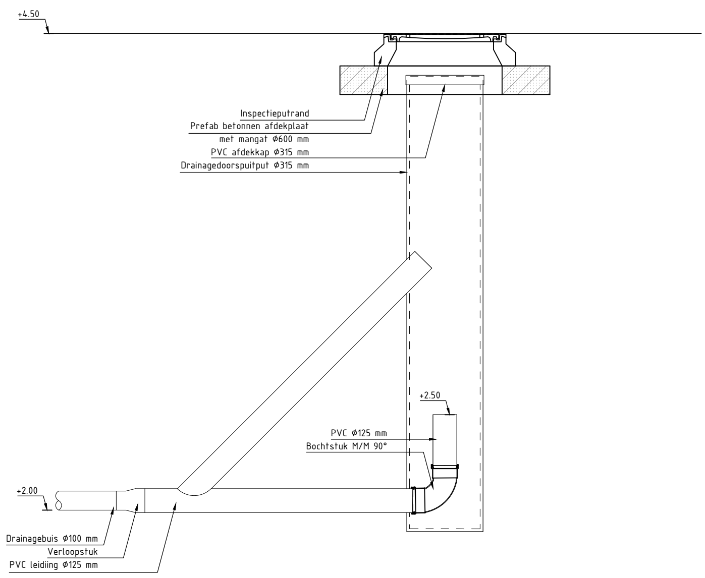
DETAIL DRAINAGEPUT MET INSTELNIVEAU SCHAAL 120
