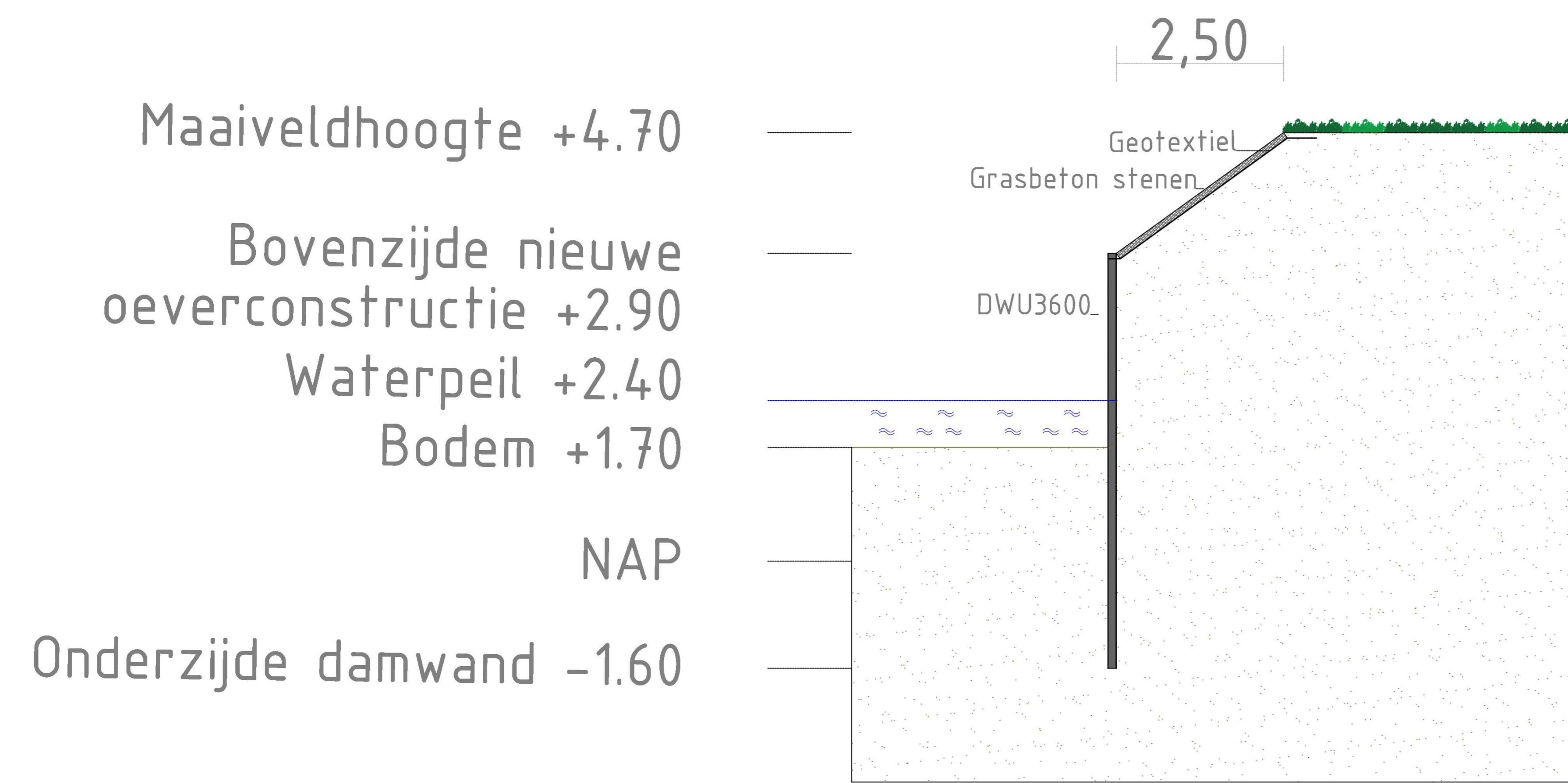
DOORSNEDE A - A schaal 1:50
