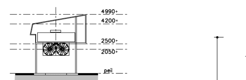
Doorsnede DD
