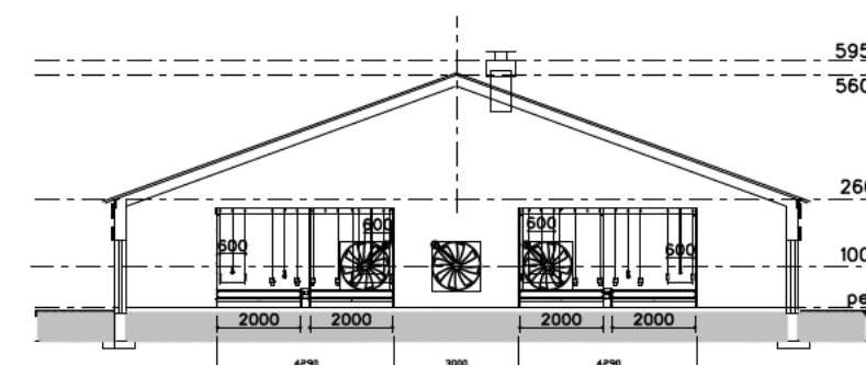
Doorsnede BB
