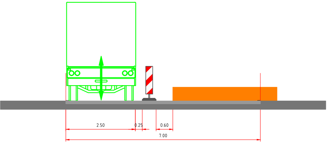
Doorsnede A-A
