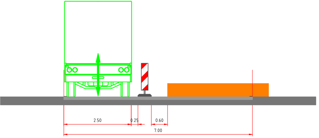
Doorsnede B-B
