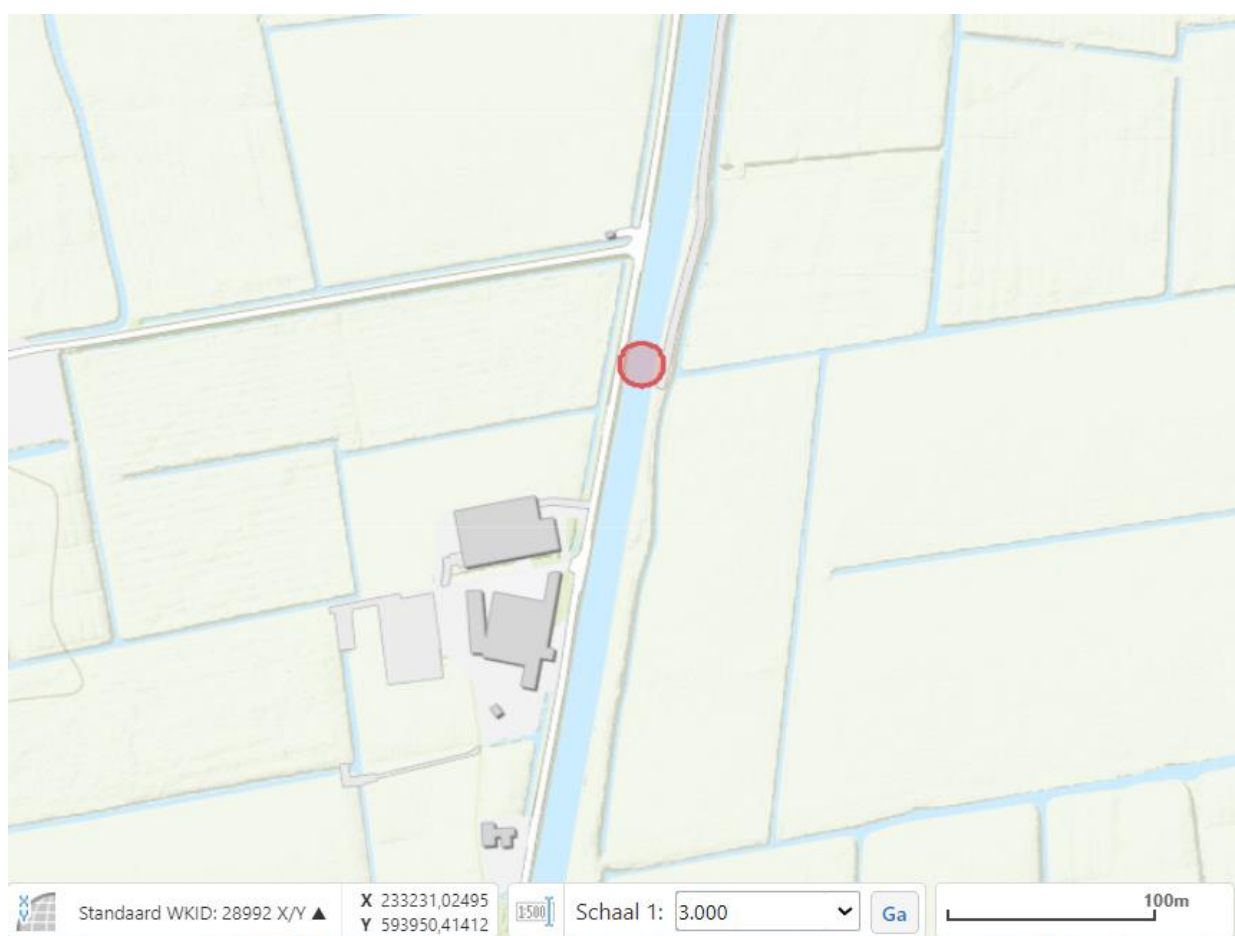
Figuur 1: De rode cirkel geeft globaal de locatie weer van de aan te leggen dam met duiker.
