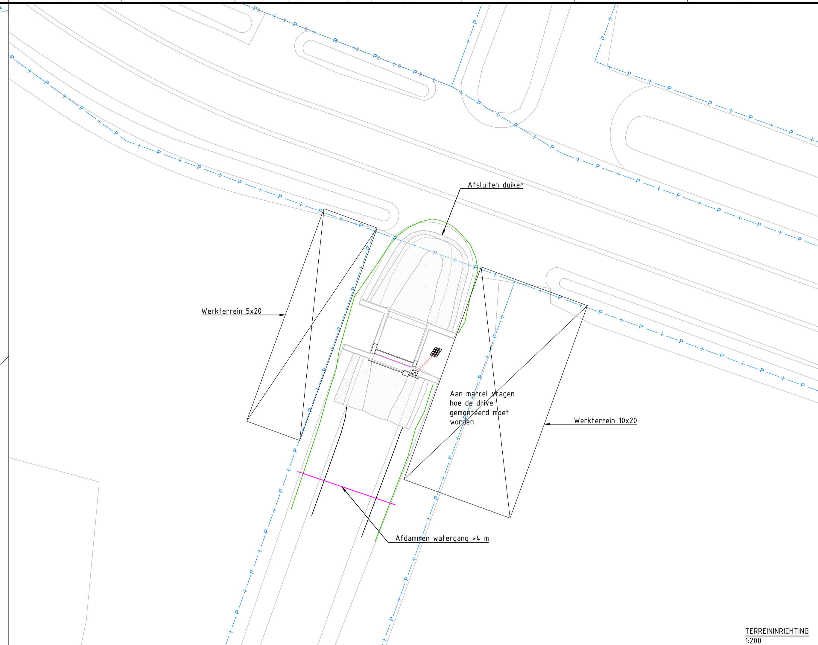
BOVENAANZICHT 1:200
