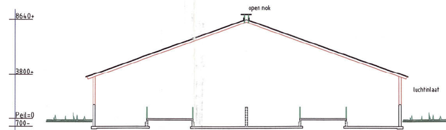
DOORSNEDE F-F, gebouw 8
