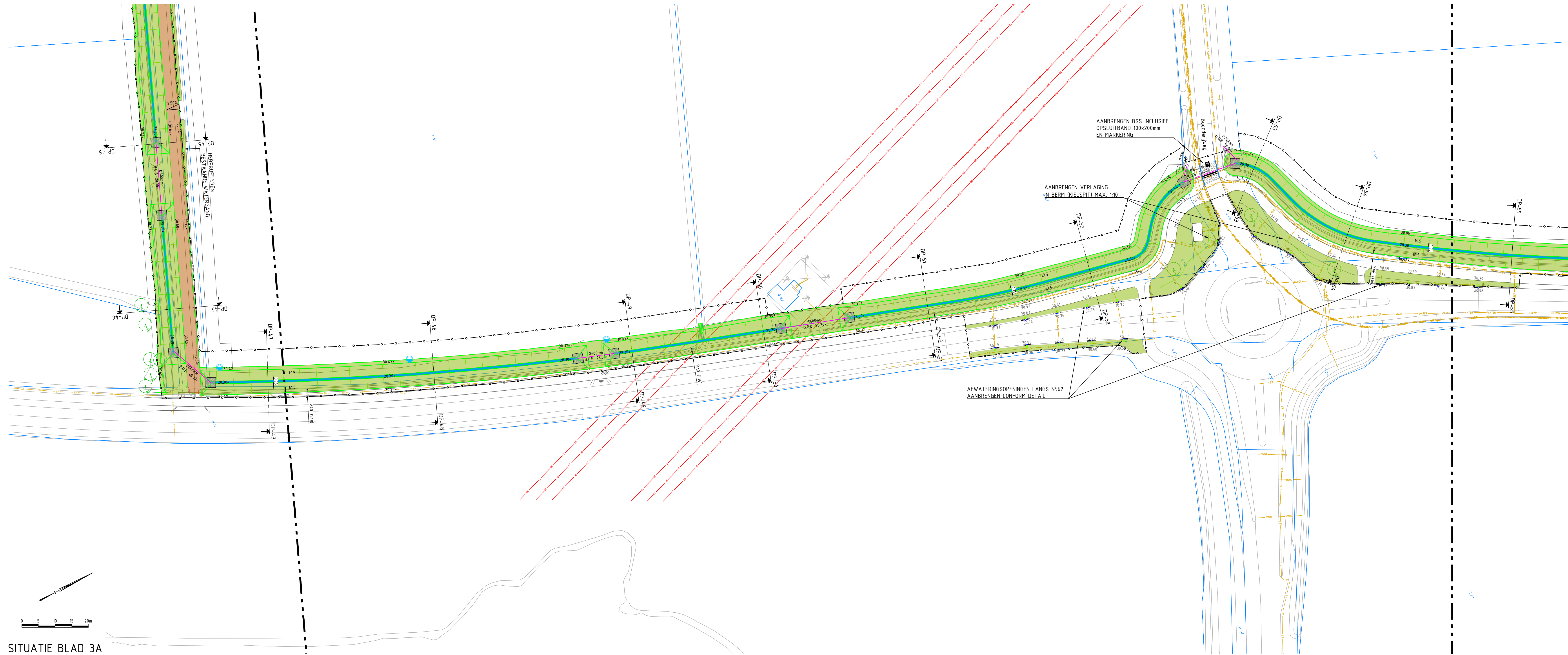
SITUATIE BLAD 3A SCHAAL 1:500
