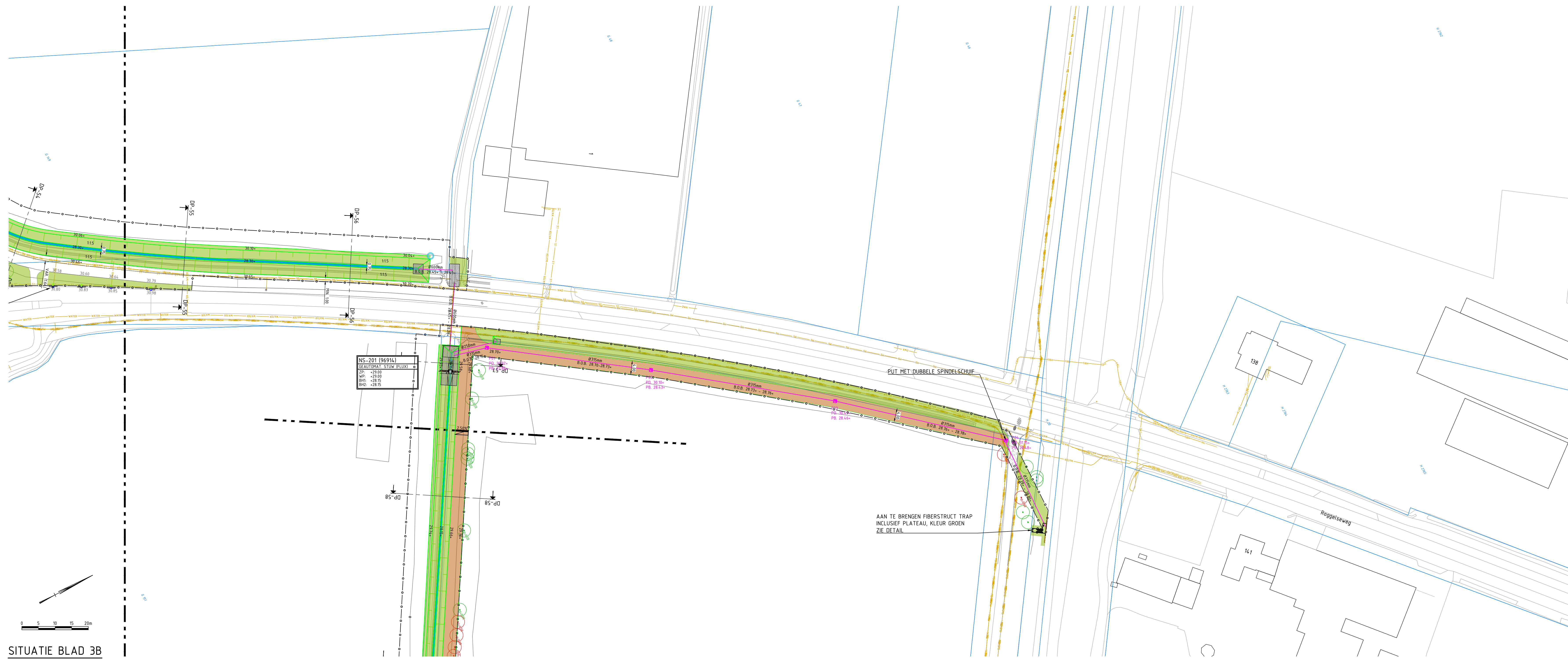
SITUATIE BLAD 3B SCHAAL 1:500
