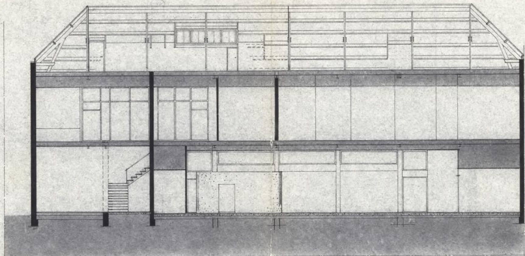
DOORSNEDE A-A
