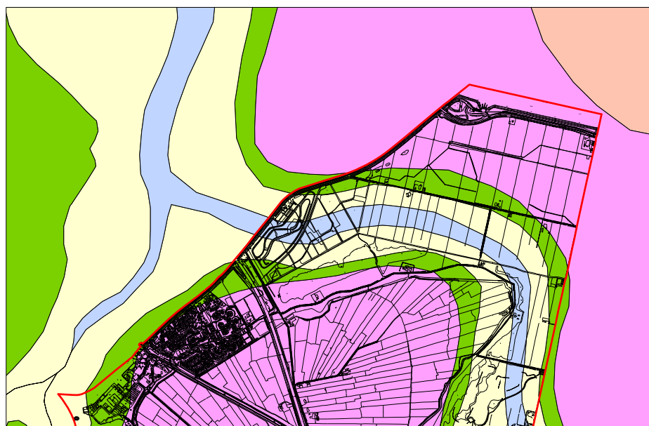
Geologie tijdvlak 1800 - 250 v. Chr.
