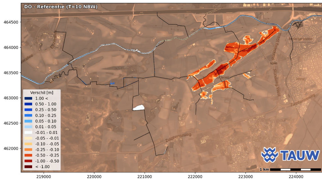
Figuur 5.35 Verskil in inundatiediepte in meters ten opzichte van de referentiesituatie (T=10+10 %-situatie)
