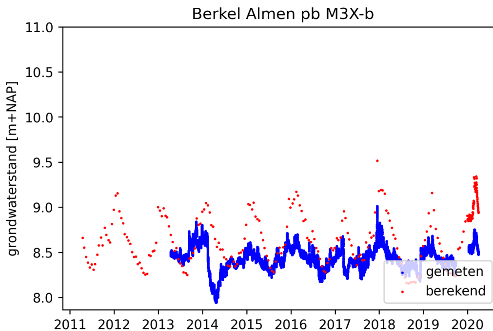
Figuur B2.3 Gemeten en berekende grondwaterstand ter hoogte van peilbuis 'Berkel Almen pb M3x-b'
