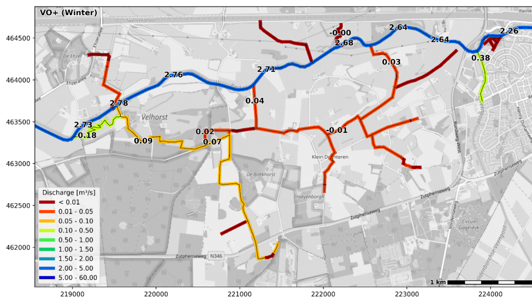
Figuur 4.9 Gemodelleerde debieten in de toekomstige situatie (gemiddelde wintersituatie)
