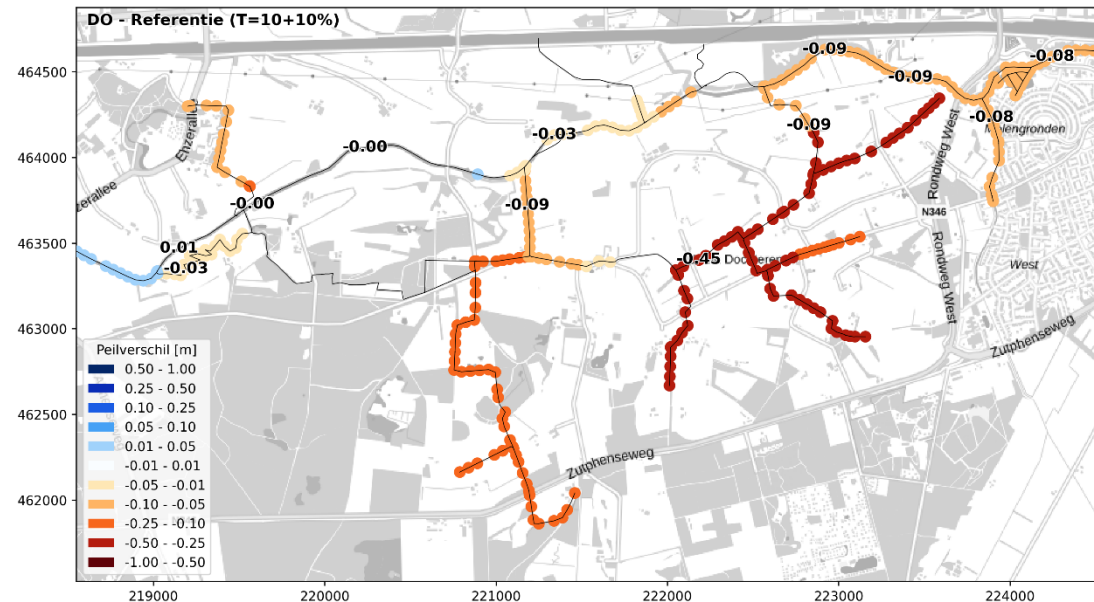
Figuur 5.25 Verschil in waterstanden (en tevens verschil in waterdiepte) ten opzichte van de referentiesituatie in meters (T=10+10 %-situatie)
