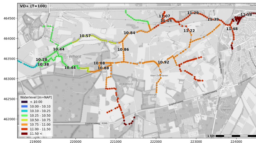
Figuur 4.17 Gemodelleerde waterstand in de toekomstige situatie in m + NAP (T=100-situatie)
