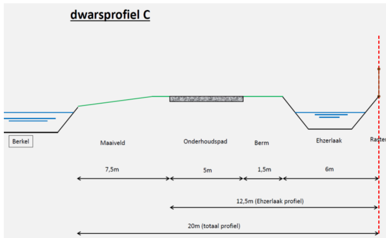
Figuur 5.10 Dwarsprofiel op locatie C, ten noorden van Velhorstbrug / Ehzerlaak
