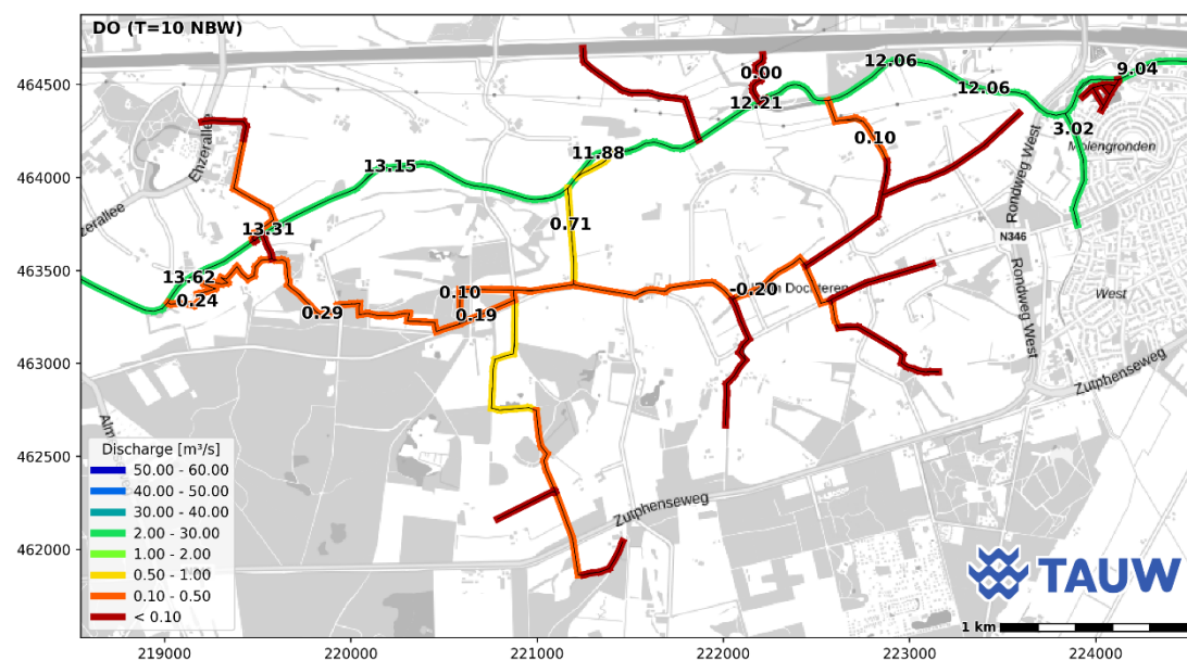
Figuur 5.16 Gemodelleerde debieten in de toekomstige situatie (T=10+10 % NBW-scenario)
