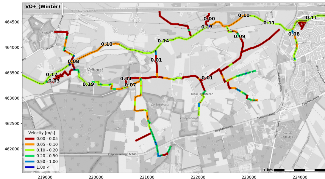
Figuur 4.26 Gemodelleerde stroomsnelheden in de toekomstige situatie (gemiddelde wintersituatie)
