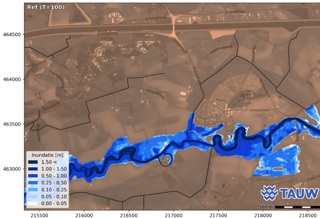
Figuur 5.38 Berekende inundatiediepte in meters ten opzichte van het maaiveld in de T=100-situatie (NB! betreft de referentiesituatie)
