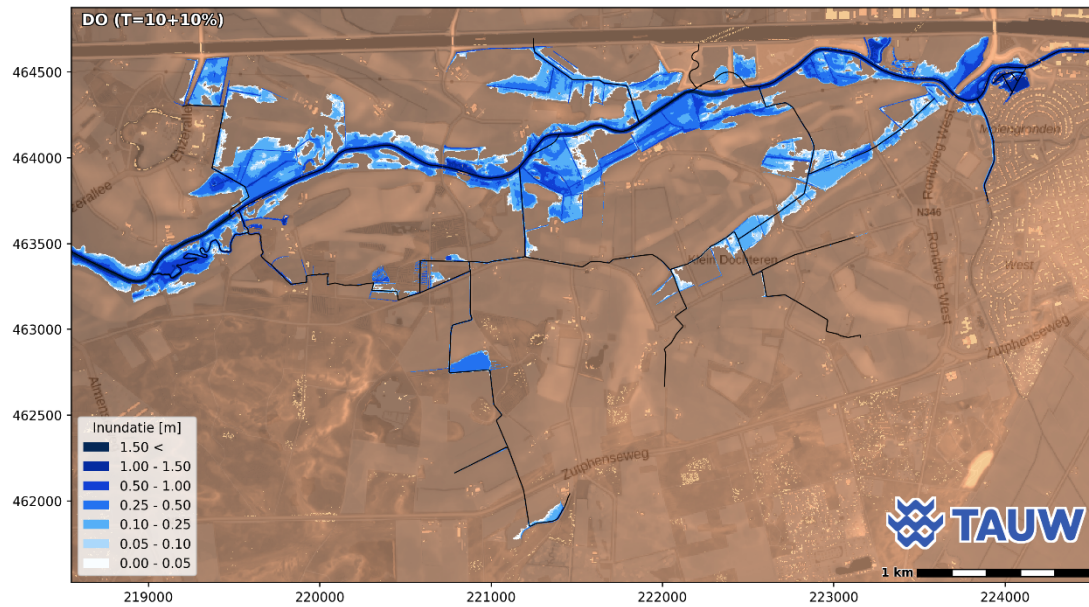
Figuur 5.32 Berekende inundatiediepte in meters ten opzichte van het maaiveld in de T=10+10 %-situatie
