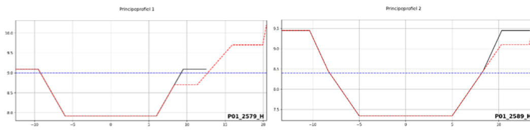
Figuur 4.3 Voorbeeld profielaanpassing modelvertalingen NVO's. Links: principeprofiel 1 (Plasberm), en rechts: principeprofiel 2 (bosoever) zoals deze in het SOBEK-model zijn geschematiseerd
