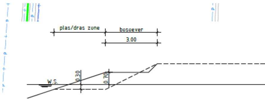
Figuur 4.4 Principe profiel natuurvriendelijke oever 'principe 2 Bosoever'
