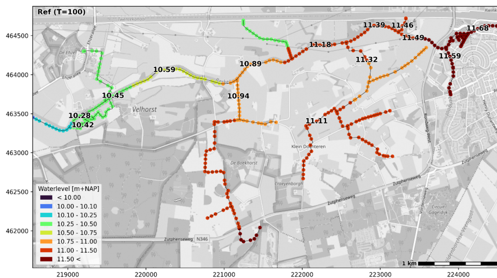
Figuur 3.10 Gemodelleerde waterstanden (m + NAP) in de huidige situatie (T=100-situatie)
