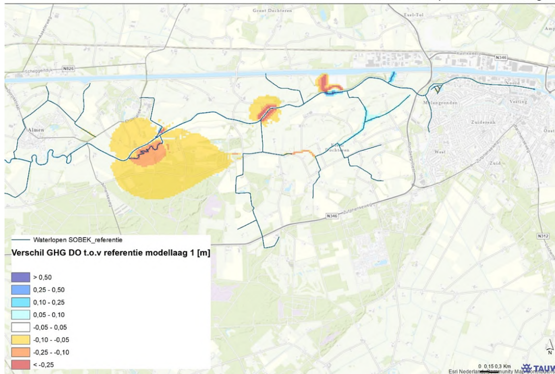
Figuur B3.17 Verschil GLG (DO minus referentie)
