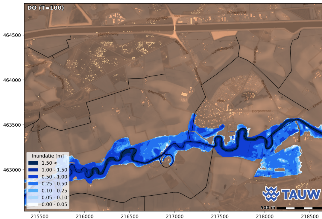
Figuur 5.39 Berekende inundatiediepte in meters ten opzichte van het maaiveld in de T=100-situatie (NB! betreft het DO)
