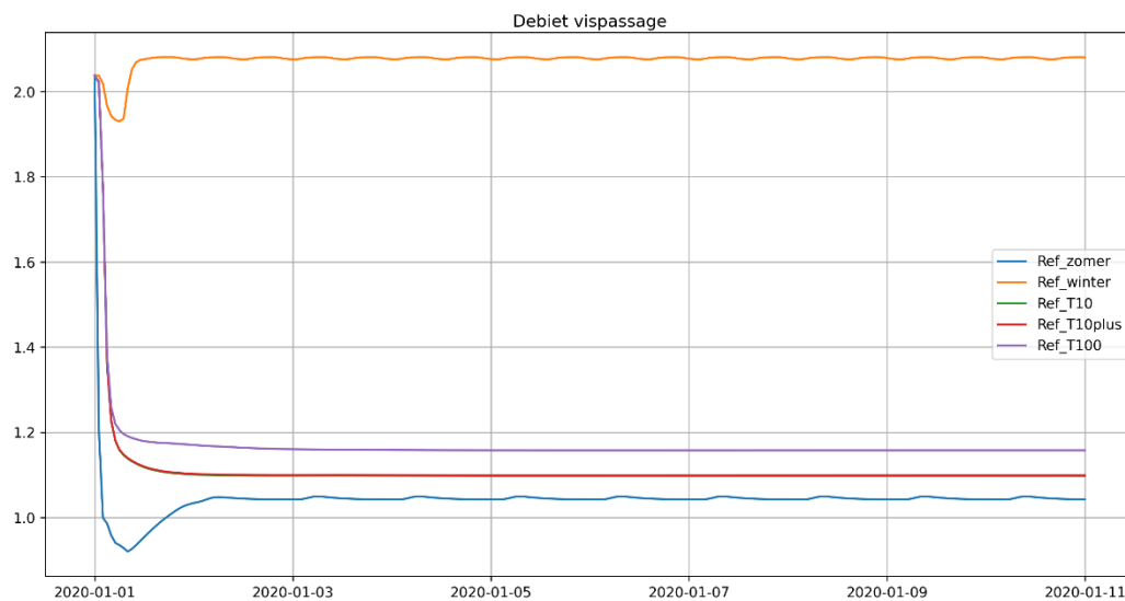
Figuur 2.4 Debieten door de vispassage in alle afvoerscenario's
