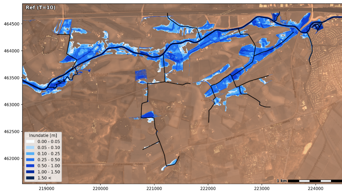
Figuur 3.14 Inundatiediepte in de T=10-situatie in meters ten opzichte van maaiveld. De kleurschaal is representatief voor de berekende inundatiediepte (zie legenda)
