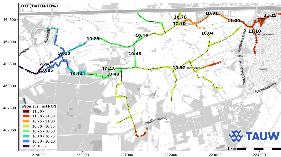
Figuur 5.20 Gemodelleerde waterstand in de toekomstige situatie in m + NAP (T=10+10 %-situatie)
