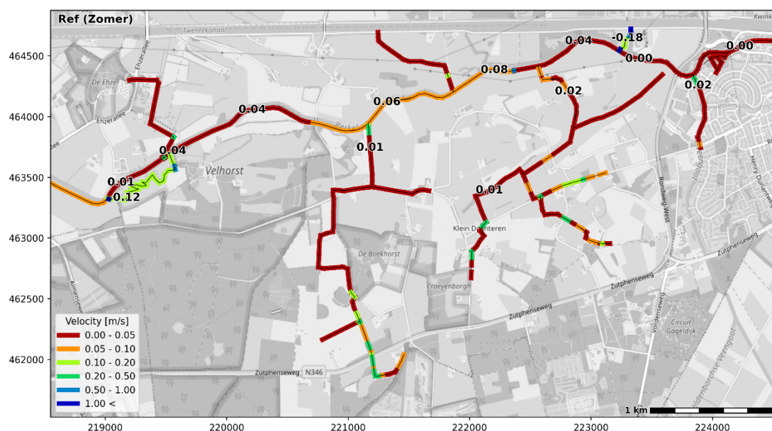
Figuur 3.12 Gemodelleerde stroomsnelheden in de huidige situatie in m/s (gemiddelde zomersituatie)
