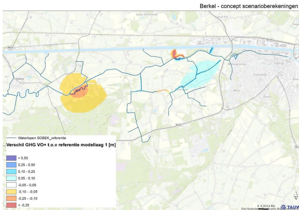
Figuur 4.35 Vershil GHG (VO++ minus referentie)
