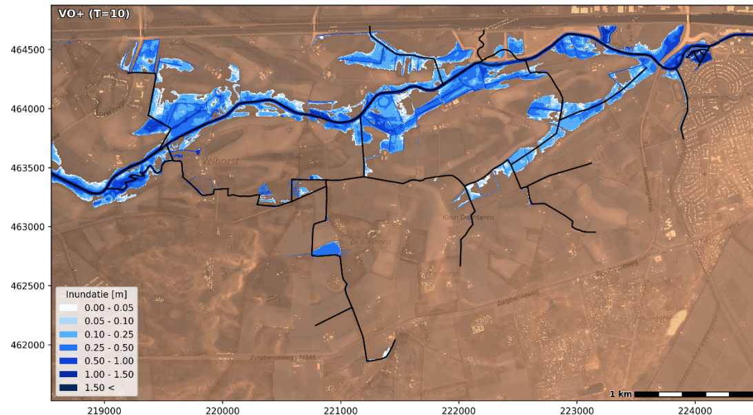
Figuur 4.27 Berekende inundatiediepte in meters ten opzichte van het maaiveld in de T=10-situatie
