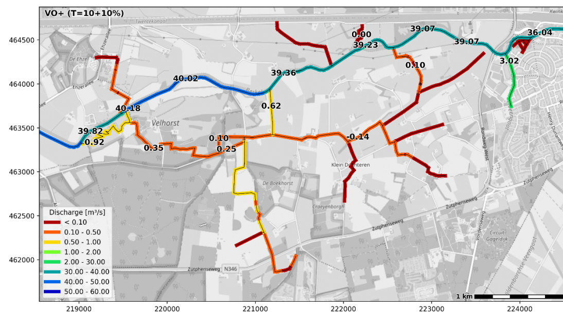
Figuur 4.11 Gemodelleerde debieten in de toekomstige situatie (T=10+10 %-situatie)
