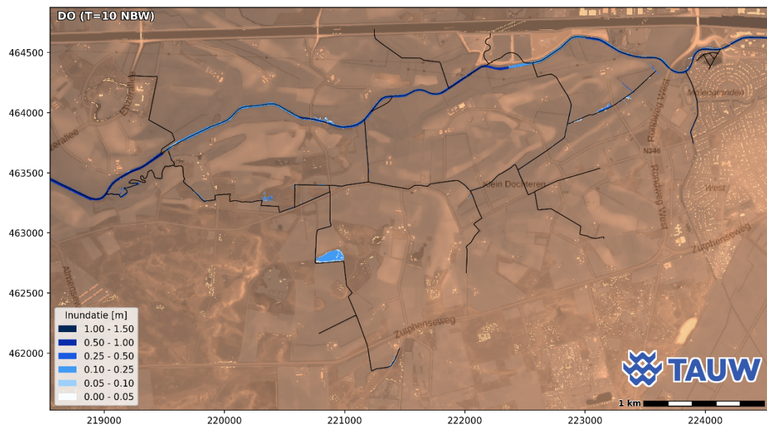
Figuur 5.34 Berekende inundatiediepte in meters ten opzichte van het maaiveld in de T=10+10 % NBW-situatie
