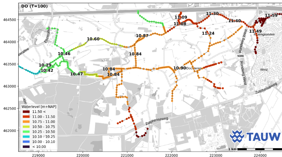
Figuur 5.22 Gemodelleerde waterstand in de toekomstige situatie in m + NAP (T=100-situatie)
