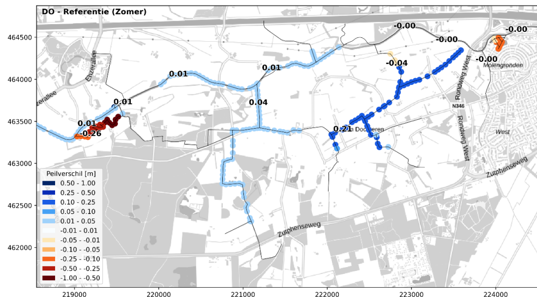
Figuur 5.23 Verskil in waterstanden (en tevens verskil in waterdiepte) ten opzichte van de referentiesituatie in meters (gemiddelde zomersituatie)
