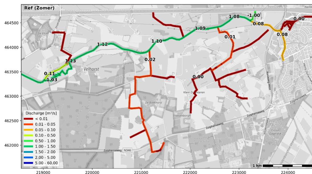
Figuur 3.1 Gemodelleerde debieten in de huidige situatie (gemiddelde zomersituatie)
