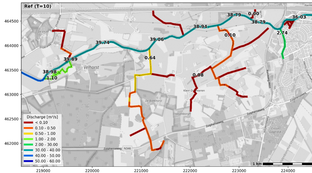
Figuur 3.3 Gemodelleerde debieten in de huidige situatie (T=10-situatie)
