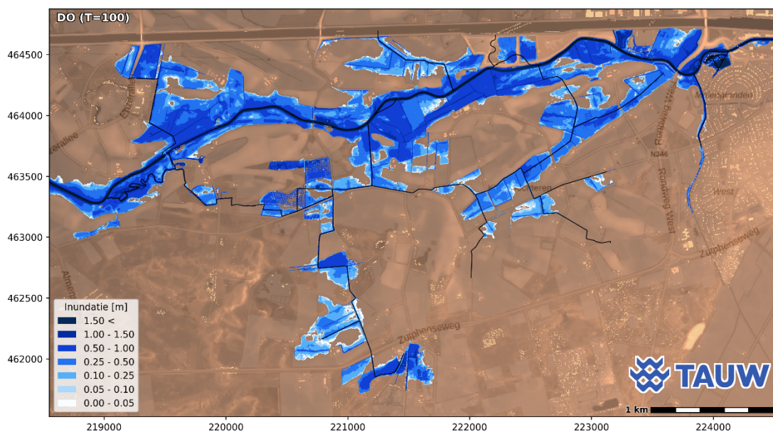
Figuur 5.36 Berekende inundatiediepte in meters ten opzichte van het maaiveld in de T=100-situatie
