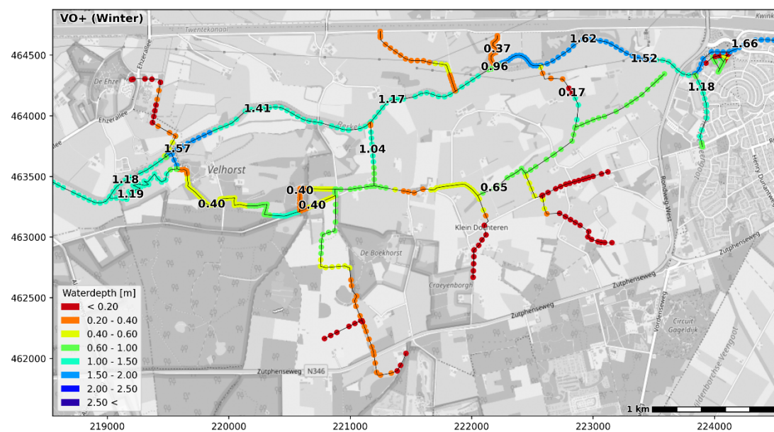
Figuur 4.24 Berekende waterdiepte in de toekomstige situatie (gemiddelde wintersituatie)
