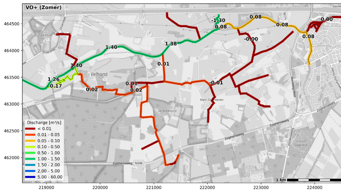
Figuur 4.8 Gemodelleerde debieten in de toekomstige situatie (gemiddelde zomersituatie)
