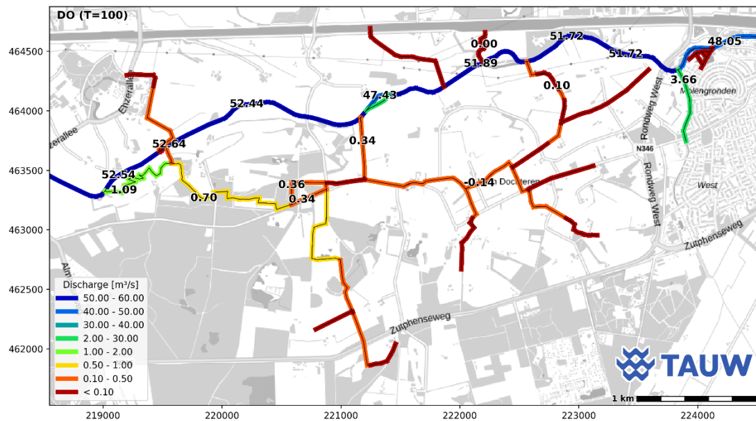
Figuur 5.17 Gemodelleerde debieten in de toekomstige situatie (T=100-situatie)
