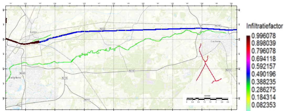
Figuur 2.10 Aangepaste Infiltratiefactor voor de Berkel tussen Lochem en Zutphen
