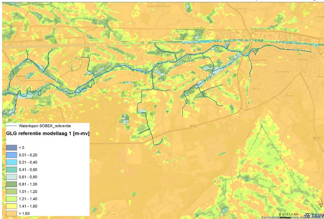
Figuur B3.21 GLG referentie (m-mv)
