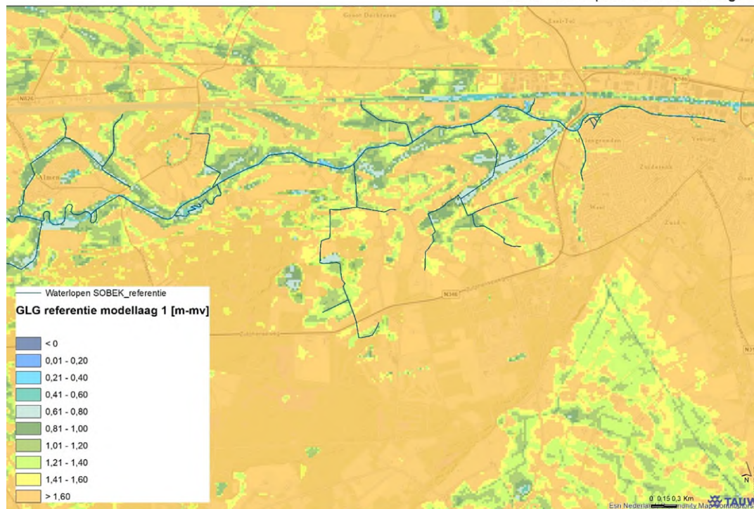
Figuur 3.18 GLG (m-mv) referentiesituatie
