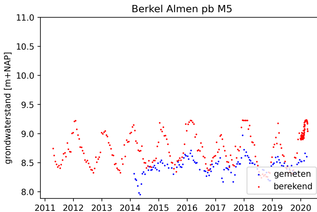
Figuur B2.2 Gemeten en berekende grondwaterstand ter hoogte van peilbuis 'Berkel Almen pb M5'
