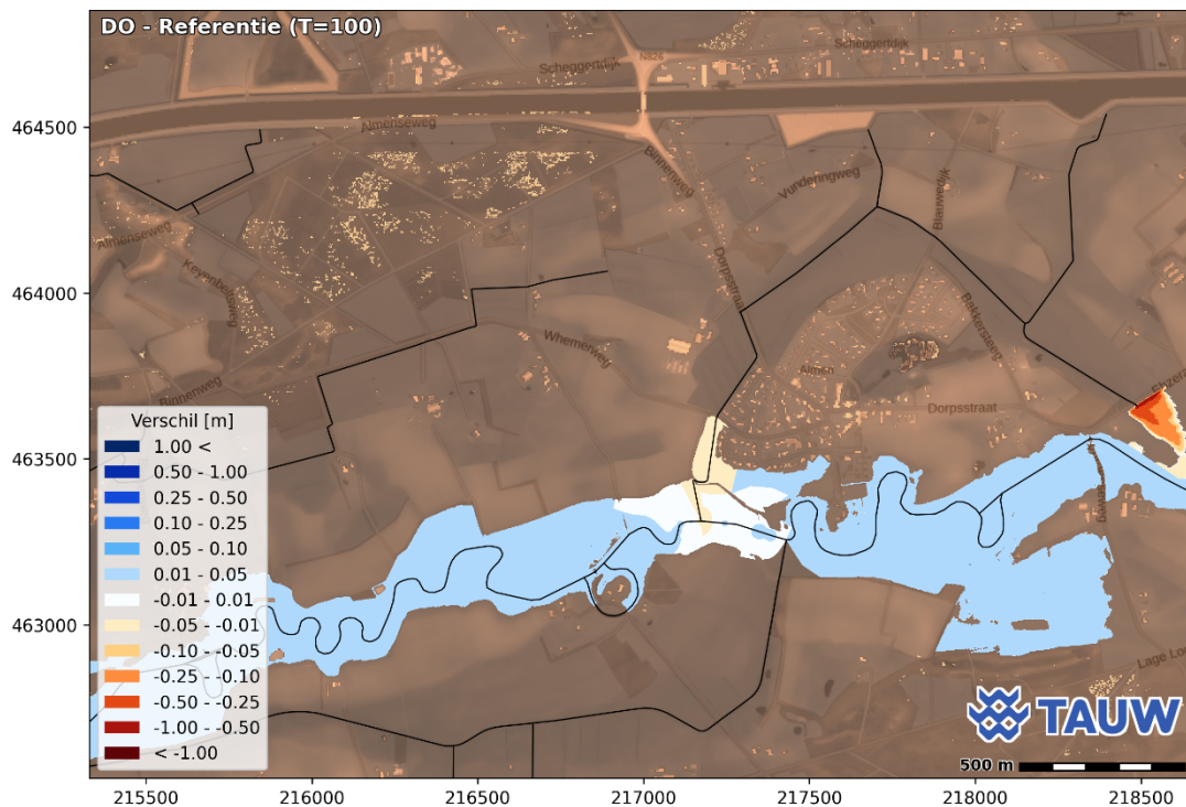
Figuur 5.40 Verschil in inundatiediepte in meters ten opzichte van de referentiesituatie (T=100-situatie)
