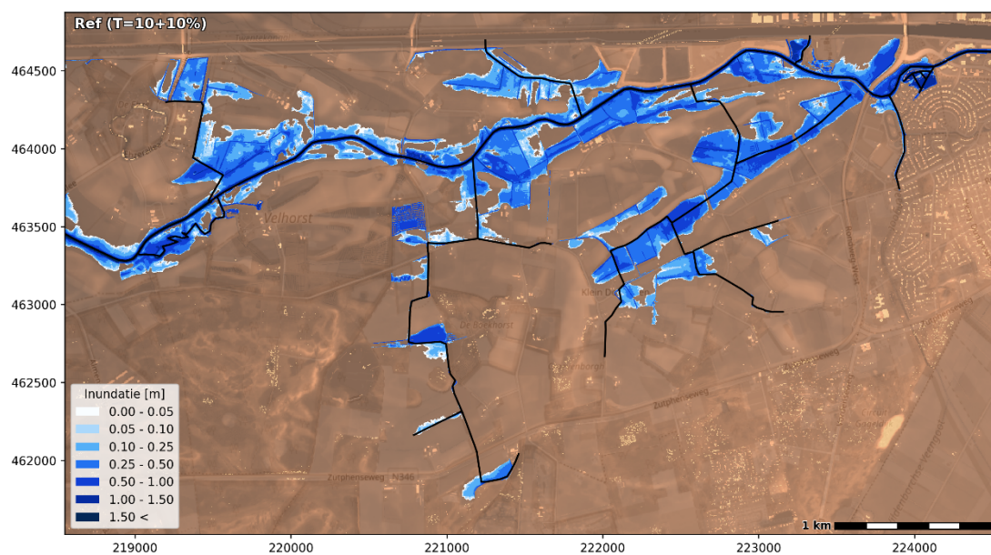
Figuur 3.15 Inundatiediepte in de T=10+10 %-situatie in meters ten opzichte van maaiveld
