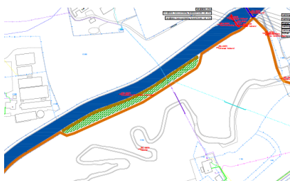
Figuur 5.2 Natuurvriendelijke oever punt 2
