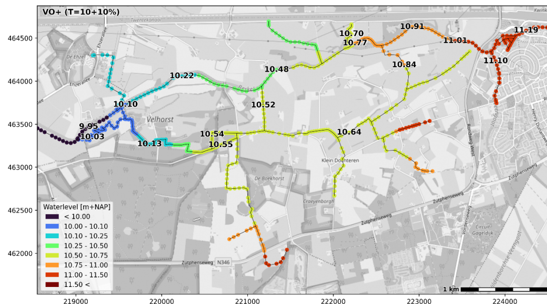
Figuur 4.16 Gemodelleerde waterstand in de toekomstige situatie in m + NAP (T=10+10 %-situatie)
