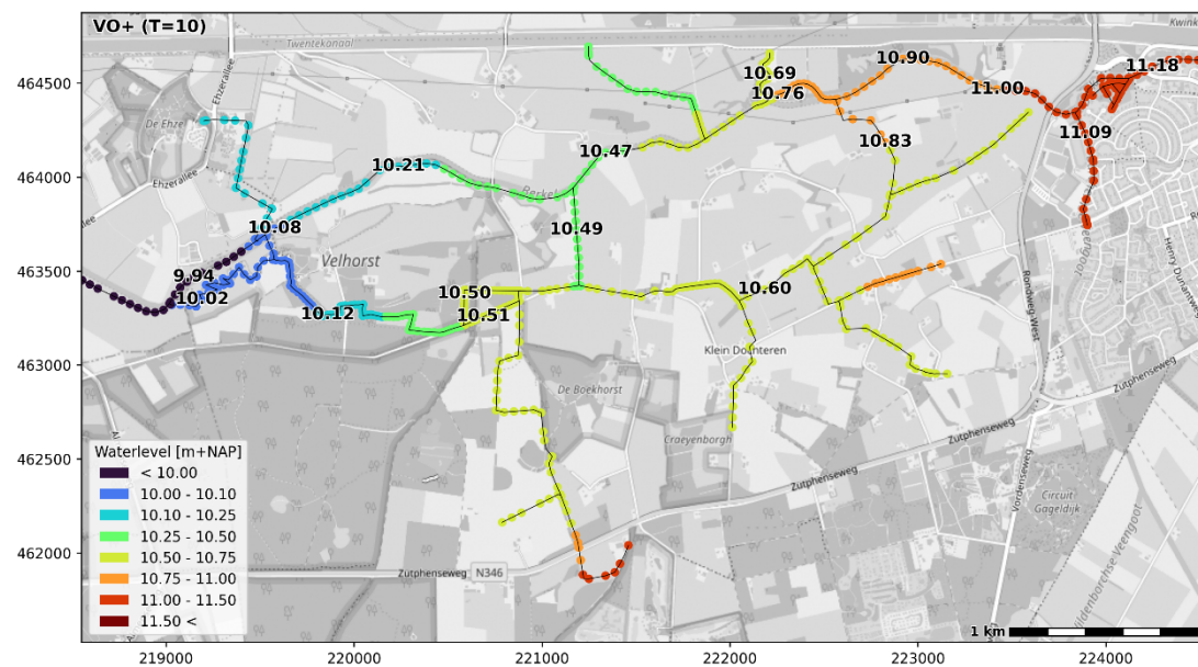
Figuur 4.15 Gemodelleerde waterstand in de toekomstige situatie in m + NAP (T=10-situatie)
