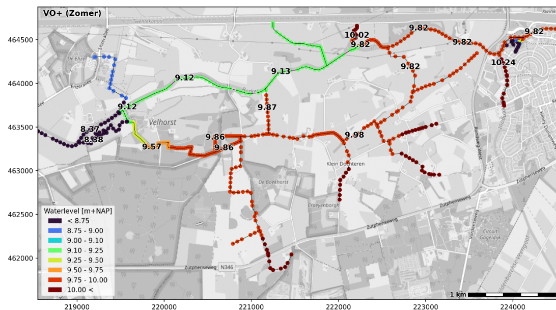
Figuur 4.13 Gemodelleerde waterstand in de toekomstige situatie in m + NAP (gemiddelde zomersituatie)
