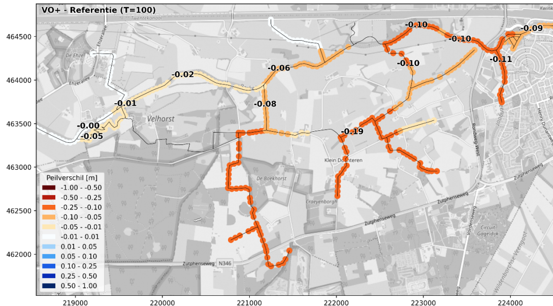
Figuur 4.22 Verschil in waterstanden (en tevens verschil in waterdiepte) ten opzichte van de referentiesituatie in meters (T=100-situatie)
