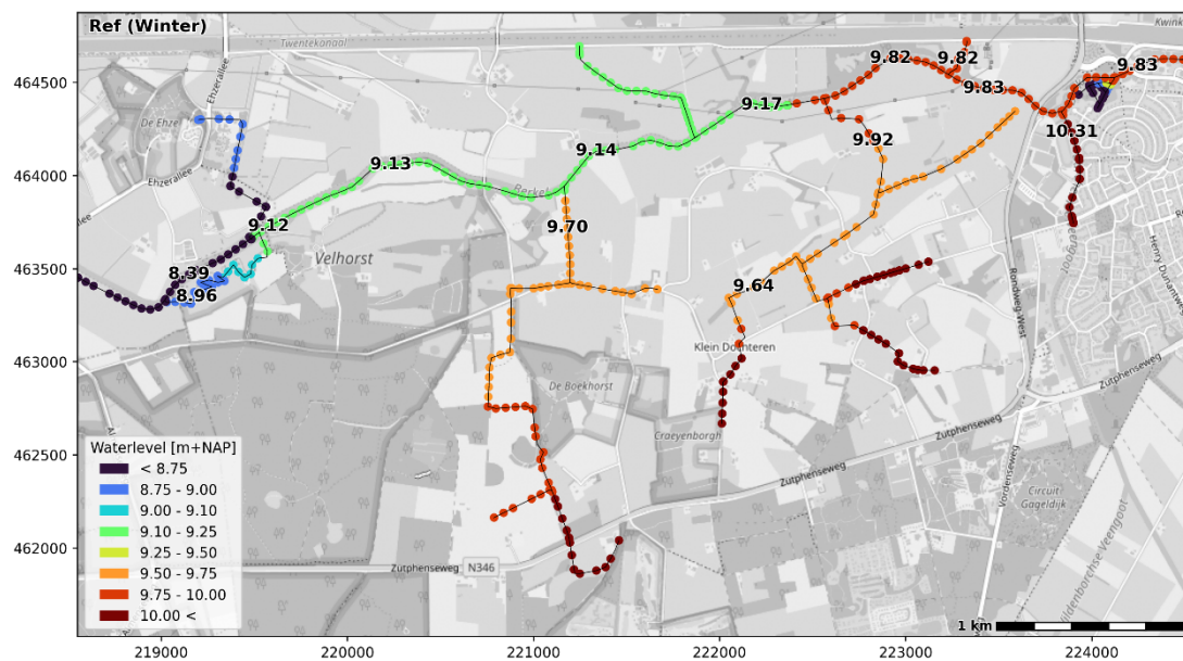
Figuur 3.7 Gemodelleerde waterstanden (m + NAP) in de huidige situatie (gemiddelde wintersituatie)
