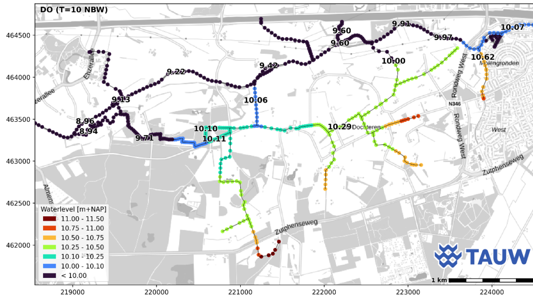
Figuur 5.21 Gemodelleerde waterstand in de toekomstige situatie in m + NAP (T=10+10 % NBW-situatie)
