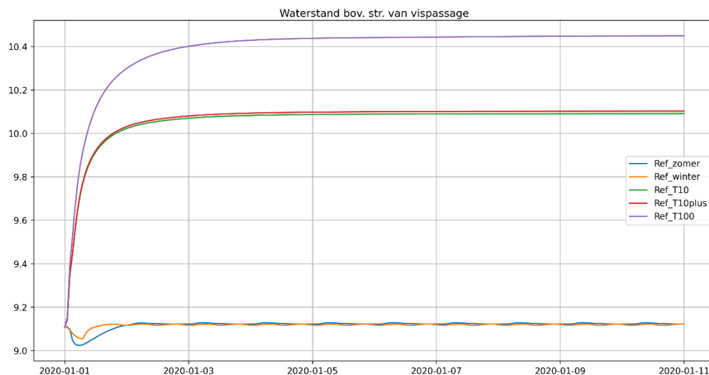
Figuur 2.3 Waterstand bovenstrooms van de vispassage voor alle afvoerscenario's. Hier is te zien dat er in alle scenario's een (quasi) steady state optreedt
