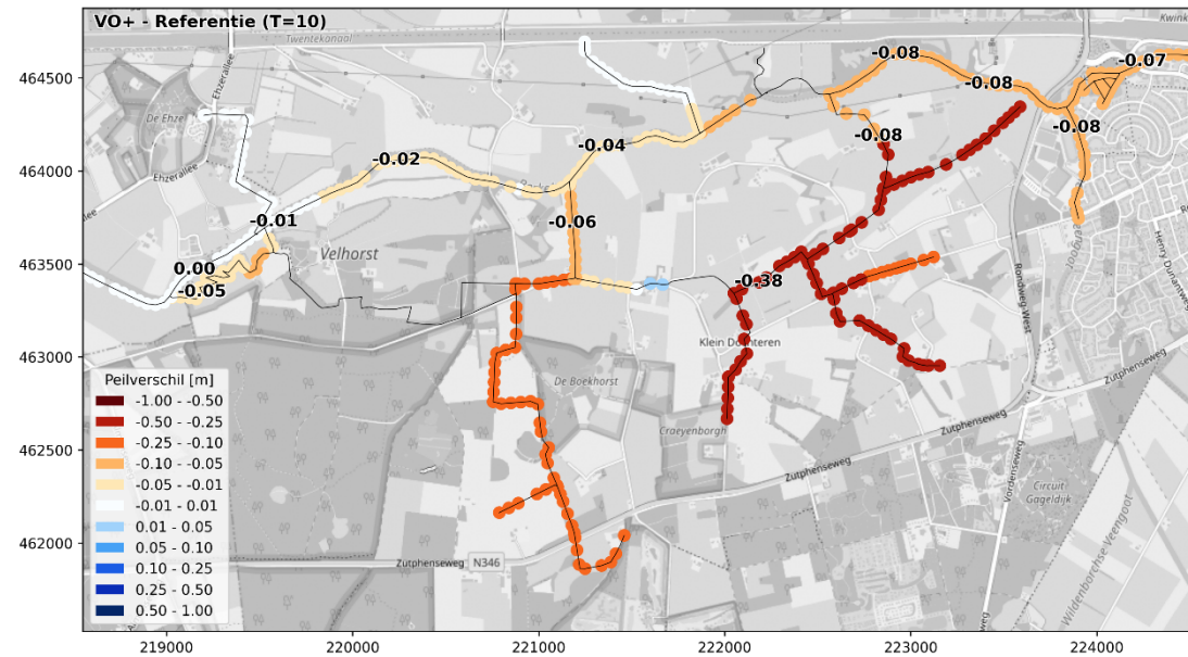
Figuur 4.20 Verschil in waterstanden (en tevens verschil in waterdiepte) ten opzichte van de referentiesituatie in meters (T=10-situatie)
