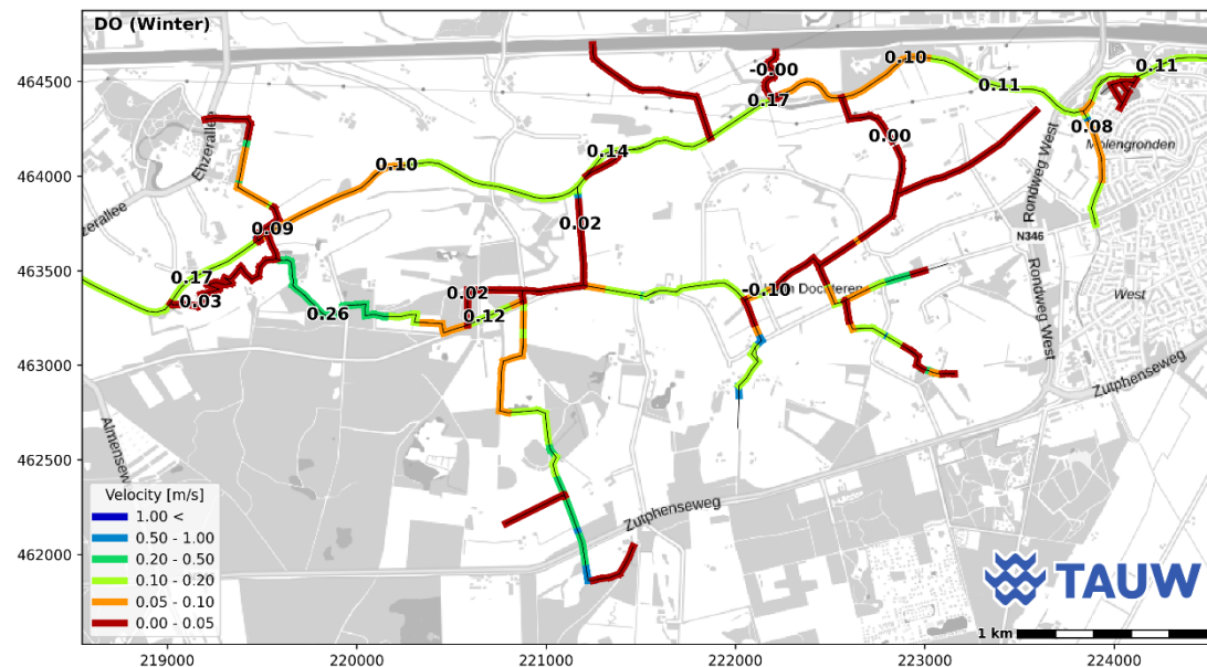
Figuur 5.31 Gemodelleerde stroomsnelheden in de toekomstige situatie (gemiddelde wintersituatie)
