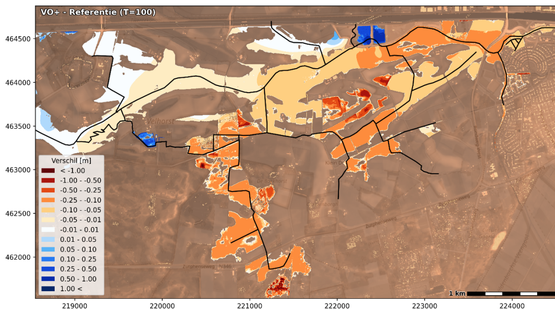
Figuur 4.33 Verschil in inundatiediepte in meters ten opzichte van de referentiesituatie (T=100-situatie)
