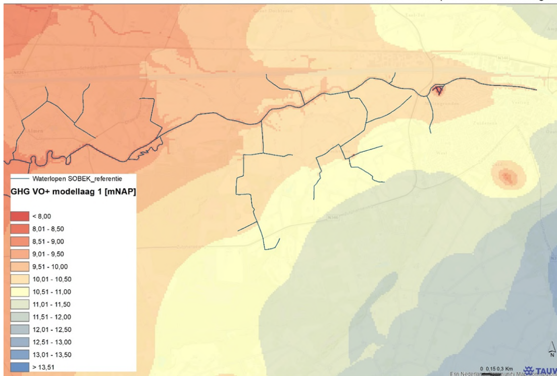
Figuur B3.11 GHG VO++ (mNAP)
