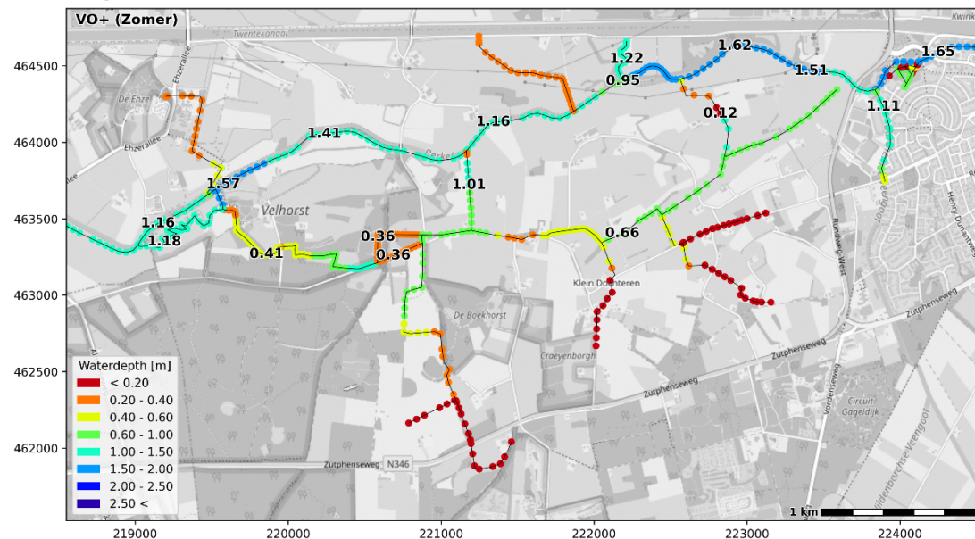
Figuur 4.23 Berekende waterdiepte in de toekomstige situatie (gemiddelde zomersituatie)
