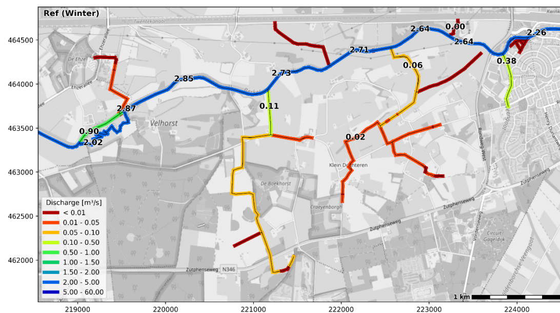
Figuur 3.2 Gemodelleerde debieten in de huidige situatie (gemiddelde wintersituatie)
