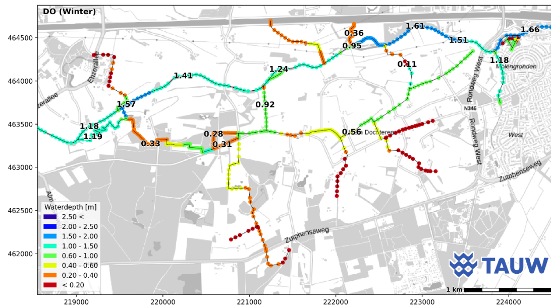
Figuur 5.29 Berekende waterdiepte in de toekomstige situatie (gemiddelde wintersituatie)
