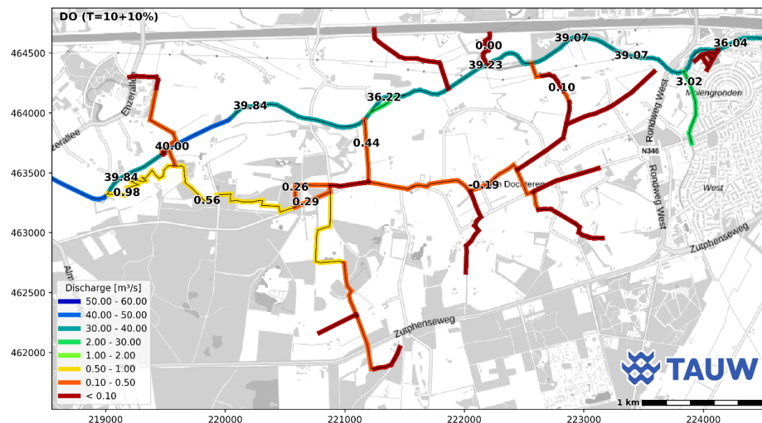
Figuur 5.15 Gemodelleerde debieten in de toekomstige situatie (T=10+10 %-situatie)
