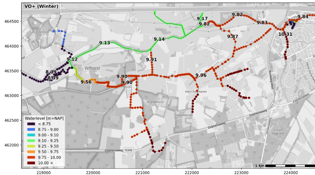
Figuur 4.14 Gemodelleerde waterstand in de toekomstige situatie in m + NAP (gemiddelde wintersituatie)
