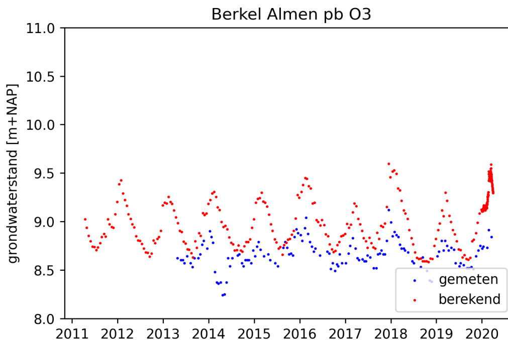
Figuur B2.4 Gemeten en berekende grondwaterstand ter hoogte van peilbuis 'Berkel Almen pb O3'
