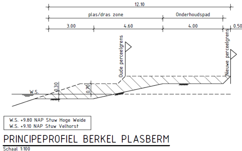
Figuur 4.2 Principe profiel natuurvriendelijke oever 'principe 1 Plasberm'
