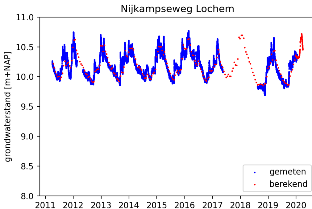
Figuur B2.6 Gemeten en berekende grondwaterstand ter hoogte van peilbuis 'Nijkampseweg Lochem'
