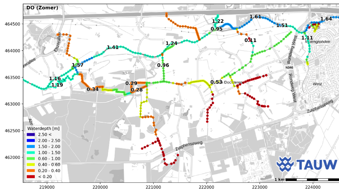
Figuur 5.28 Berekende waterdiepte in de toekomstige situatie (gemiddelde zomersituatie)
