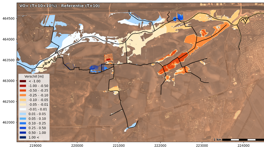
Figuur 4.31 Verschil in inundatiediepte in het VO (T=10+10 %-situatie) ten opzichte van de referentiesituatie (T=10-situatie) in meters. Blauw duidt op toename en rood duidt op afname van inundatiediepte
