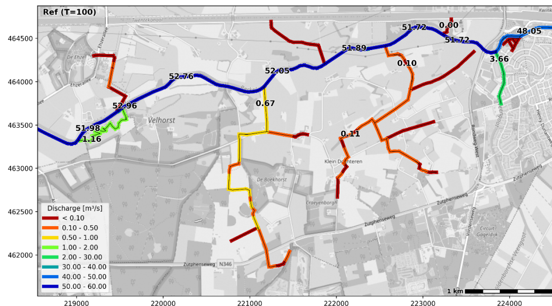
Figuur 3.5 Gemodelleerde debieten in de huidige situatie (T=100-situatie)
