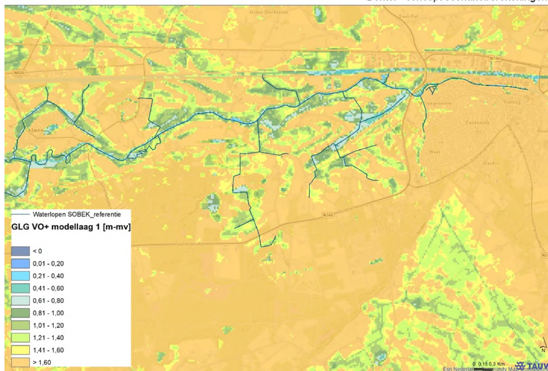
Figuur B3.7 GLG VO++ (m-mv)
