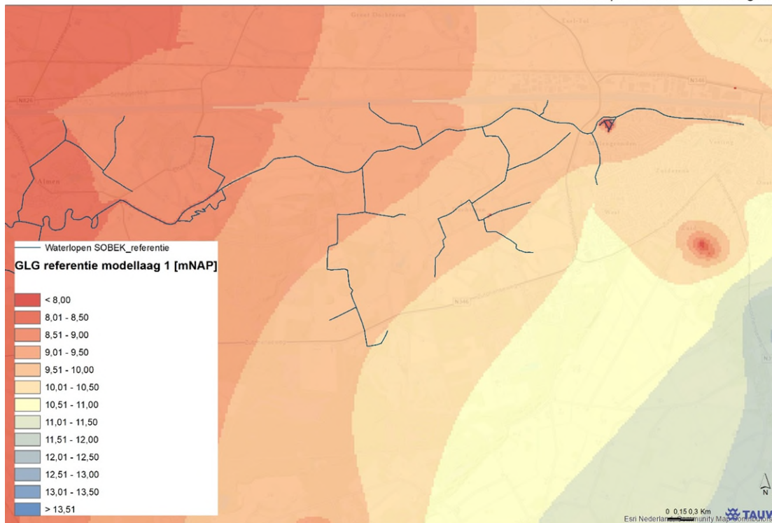
Figuur B3.12 GLG referentie (mNAP)
