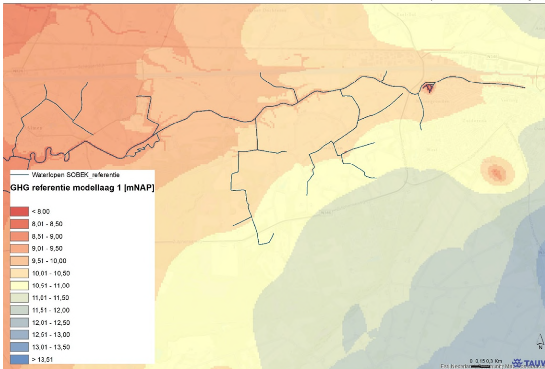
Figuur B3.10 GHG-referentie (mNAP)
