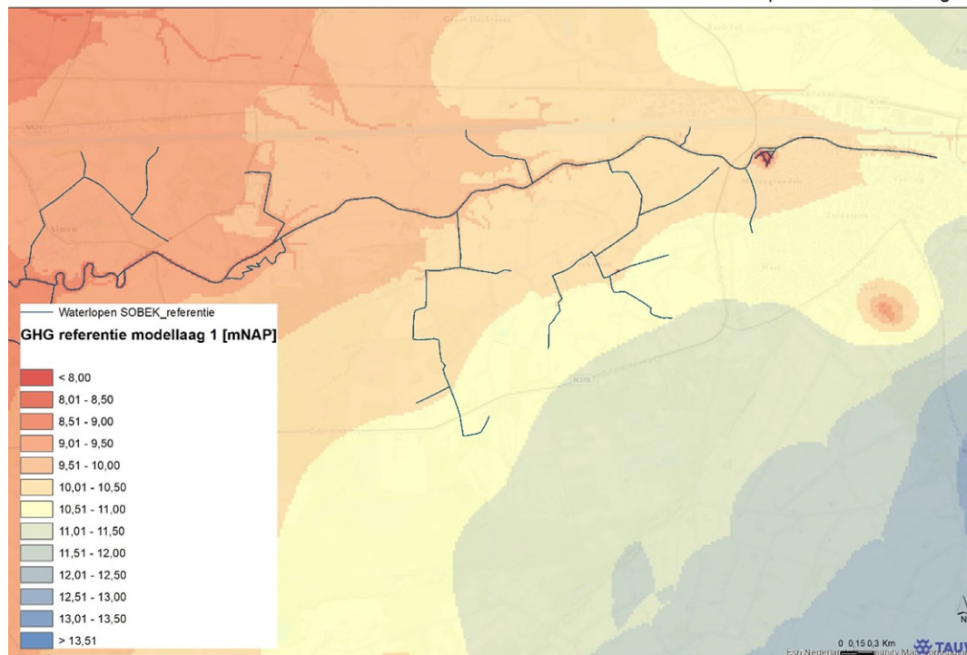
Figuur 3.20 GHG (mNAP) referentiesituatie
