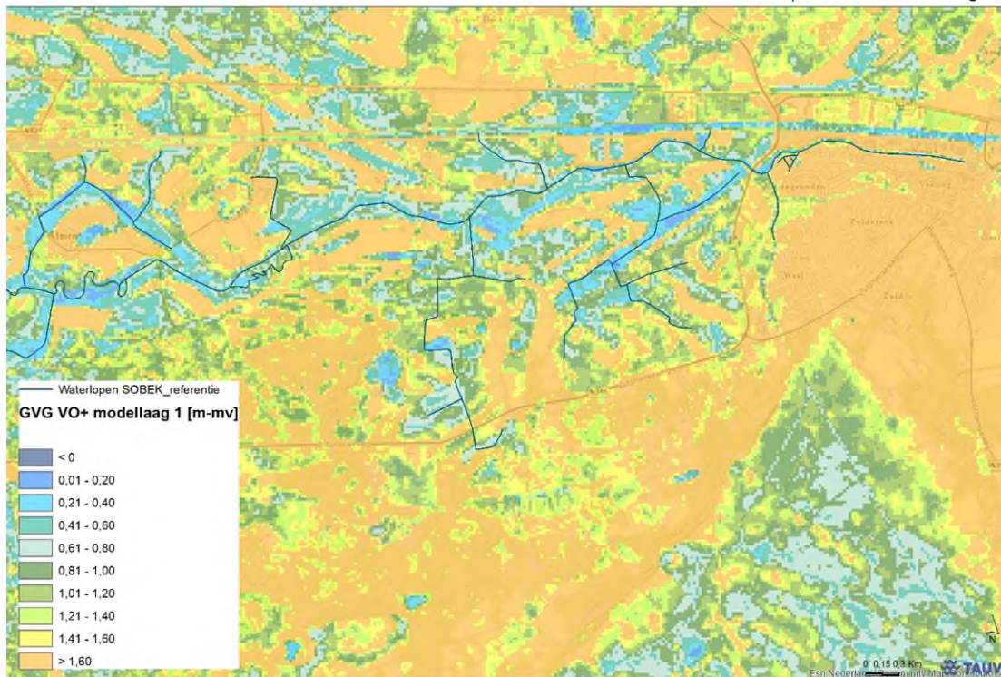
Figuur B3.9 GVG VO++ (m-mv)
