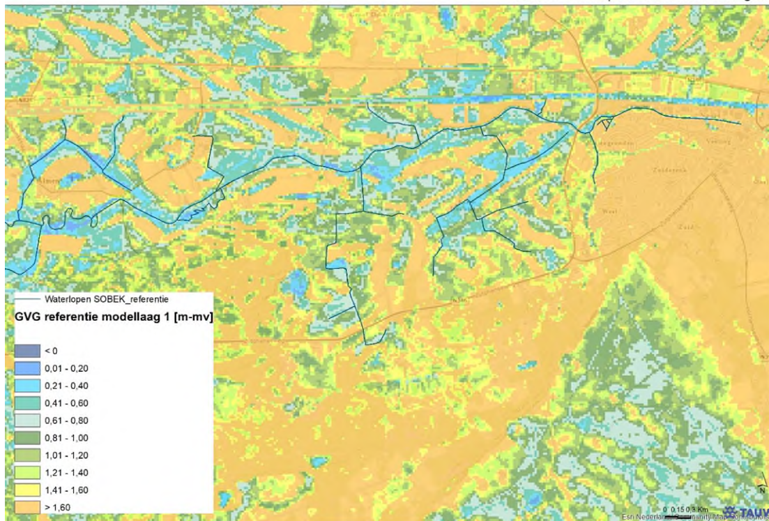
Figuur B3.8 GVG-referentie (m-mv)
