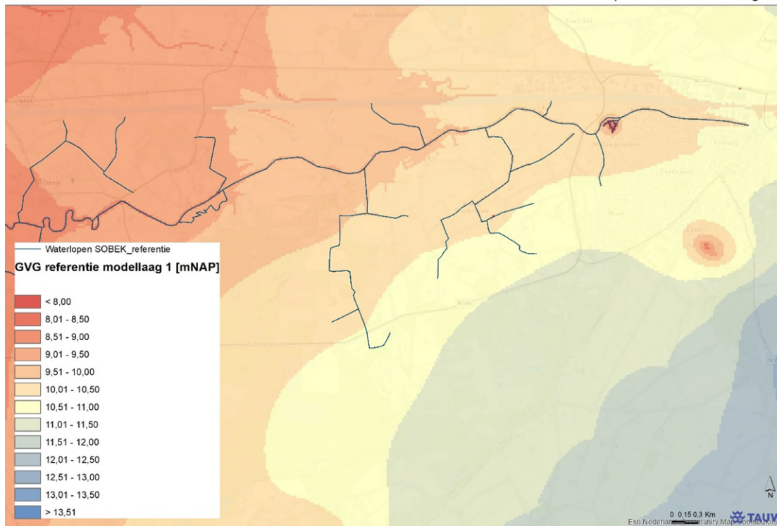
Figuur B3.14 GVG-referentie (mNAP)
