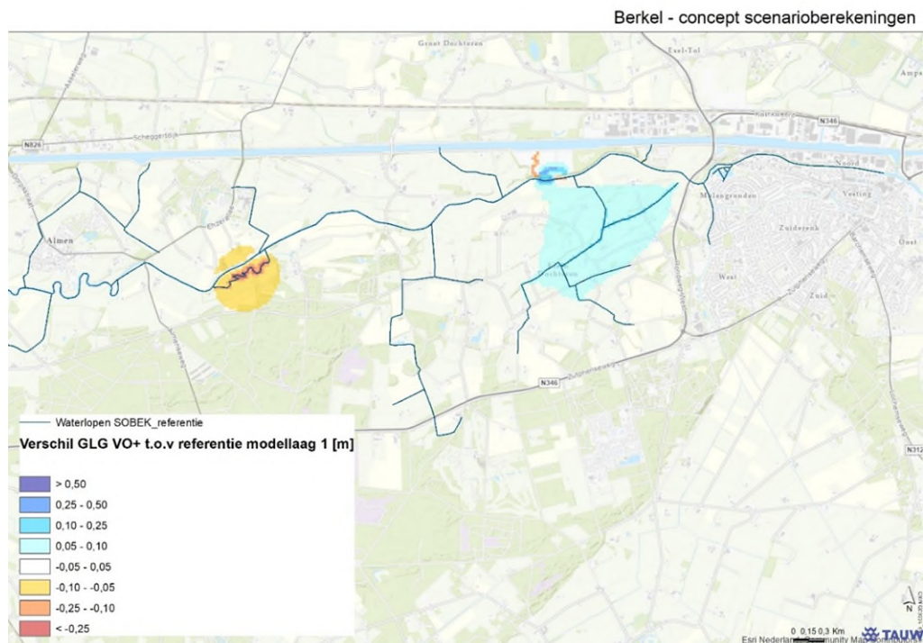
Figuur 4.36 Vershil GLG (VO++ minus referentie)
