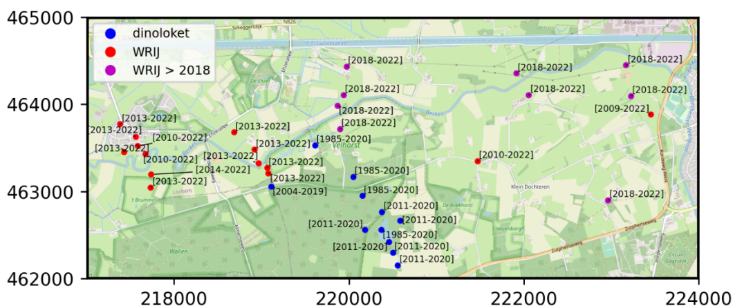
Figuur 2.14 Peilbuislocaties validatieset met meetperiode
