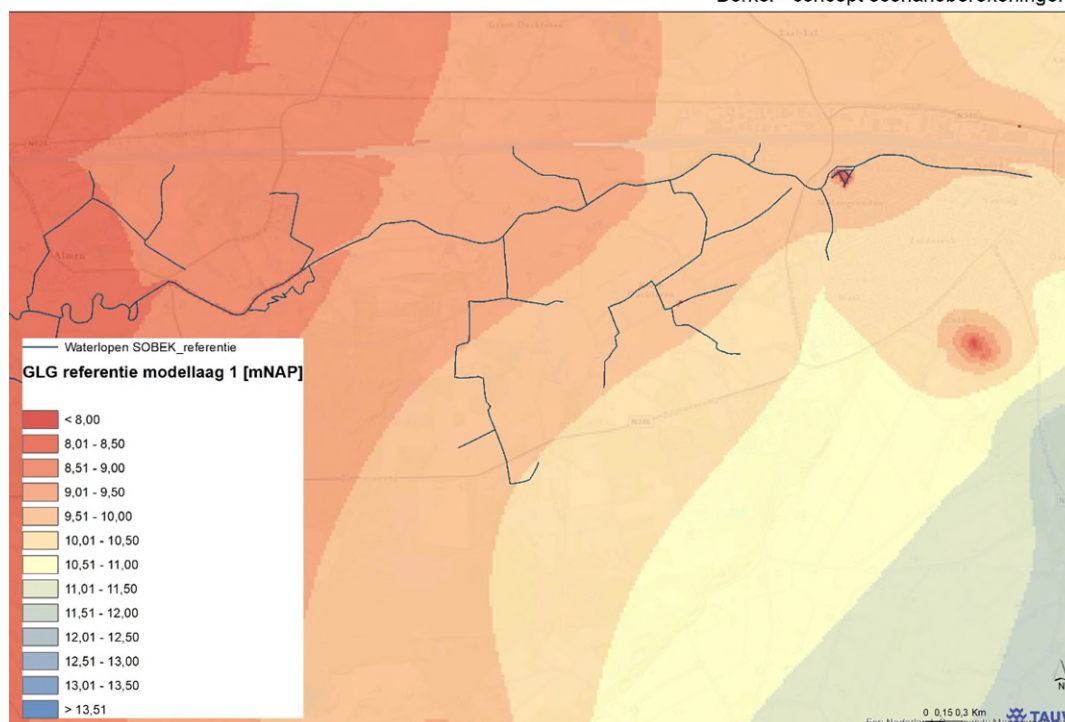
Figuur 3.21 GLG (mNAP) referentiesituatie
