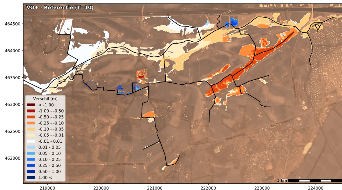
Figuur 4.28 Verskil in inundatiediepte in het VO ten opzichte van de referentiesituatie in de T=10-situatie (in meters). Blauw duidt op toename en rood duidt op afname van inundatiediepte
