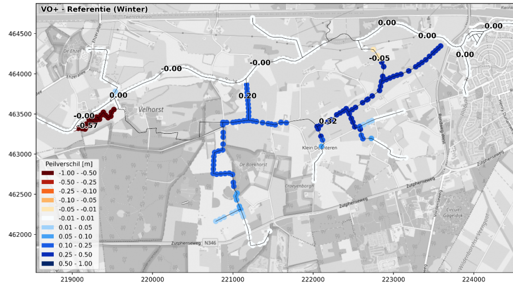
Figuur 4.19 Verschil in waterstanden (en tevens verschil in waterdiepte) ten opzichte van de referentiesituatie in meters (gemiddelde wintersituatie)
