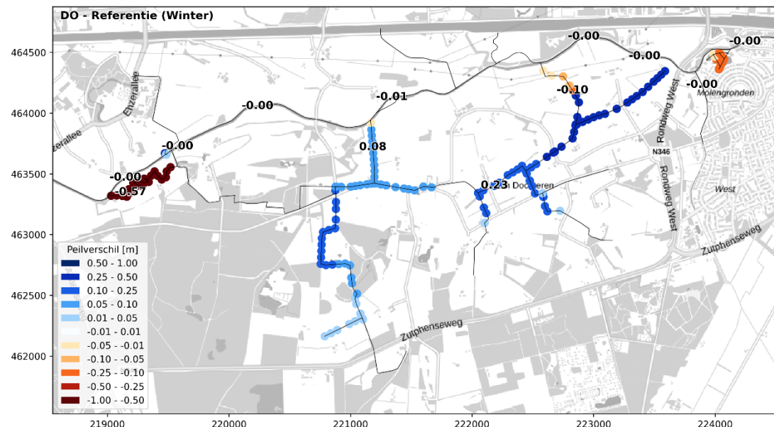
Figuur 5.24 Verschil in waterstanden (en tevens verschil in waterdiepte) ten opzichte van de referentiesituatie in meters (gemiddelde wintersituatie)
