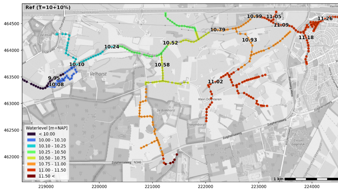
Figuur 3.9 Gemodelleerde waterstanden (m + NAP) in de huidige situatie (T=10+10 %-situatie)
