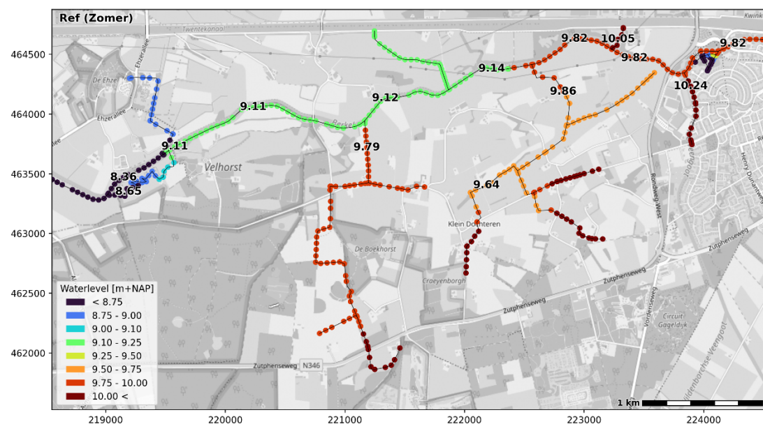
Figuur 3.6 Gemodelleerde waterstanden (m + NAP) in de huidige situatie (gemiddelde zomersituatie)
