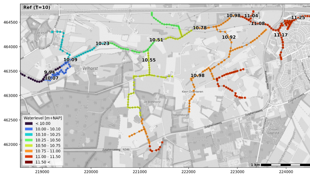
Figuur 3.8 Gemodelleerde waterstanden (m + NAP) in de huidige situatie (T=10-situatie)
