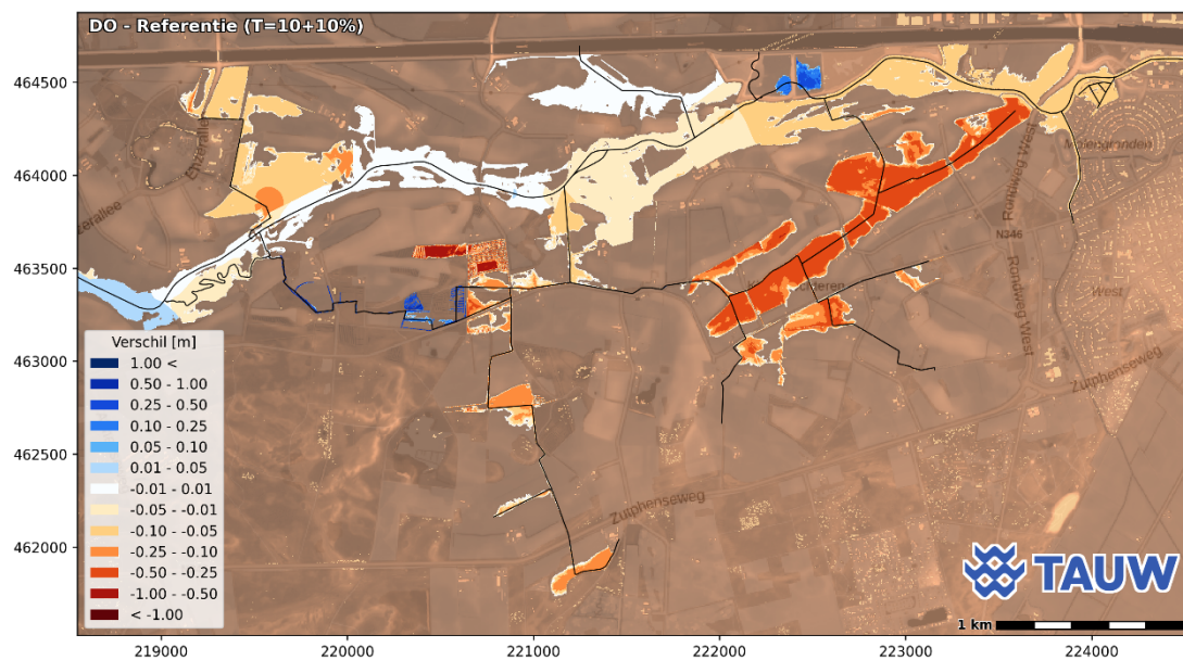
Figuur 5.33 Verschil in inundatiediepte in het VO ten opzichte van de referentiesituatie in de T=10-situatie (in meters). Blauw duidt op toename en rood duidt op afname van inundatiediepte
