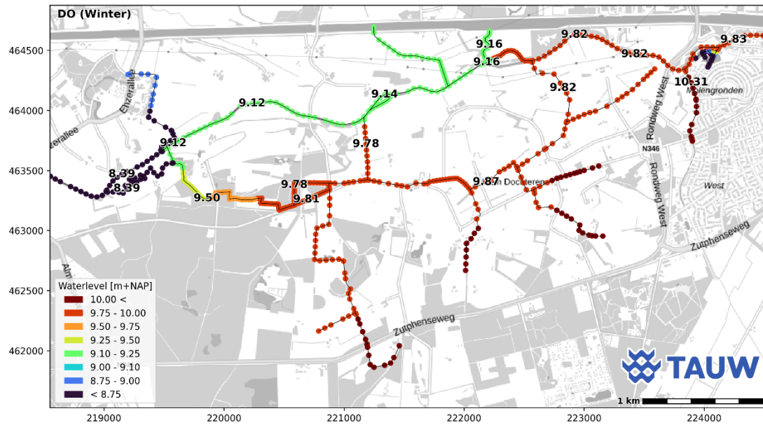
Figuur 5.19 Gemodelleerde waterstand in de toekomstige situatie in m + NAP (gemiddelde wintersituatie)
