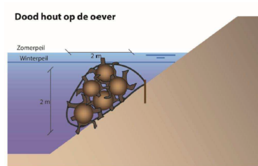
Figuur 5.11 Principe van toepassing van dood hout in de Berkel (Bron: hydrologische onderbouwing DO's Karshoek Stegeren en Rheezermaten, Vechtstromen 2019)
