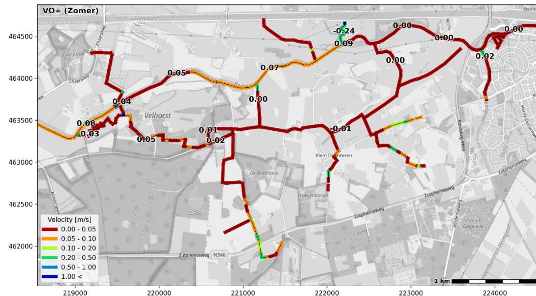
Figuur 4.25 Gemodelleerde stroomsnelheden in de toekomstige situatie (gemiddelde zomersituatie)
