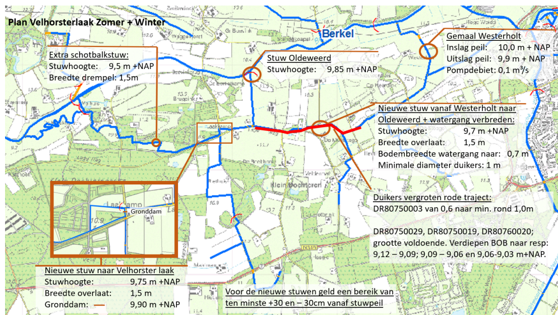
Figuur 4.6 Modelaanpassing #4. Aantakken Velhorsterlaak. In bruin de locatie van de kunstwerken. In rood de locatie van de te verbreden watergang (niet overgenomen in VO++) en te vergroten duikers (wel meegenomen in VO++)
