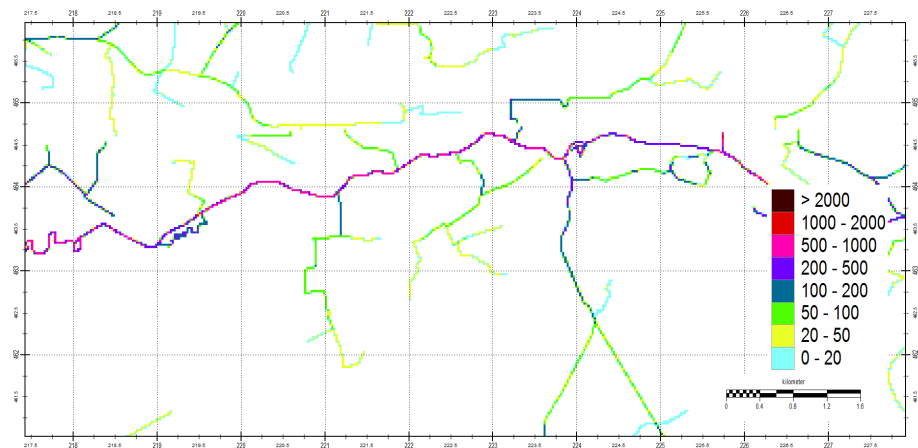
Figuur B4.4 Conductance referentie
