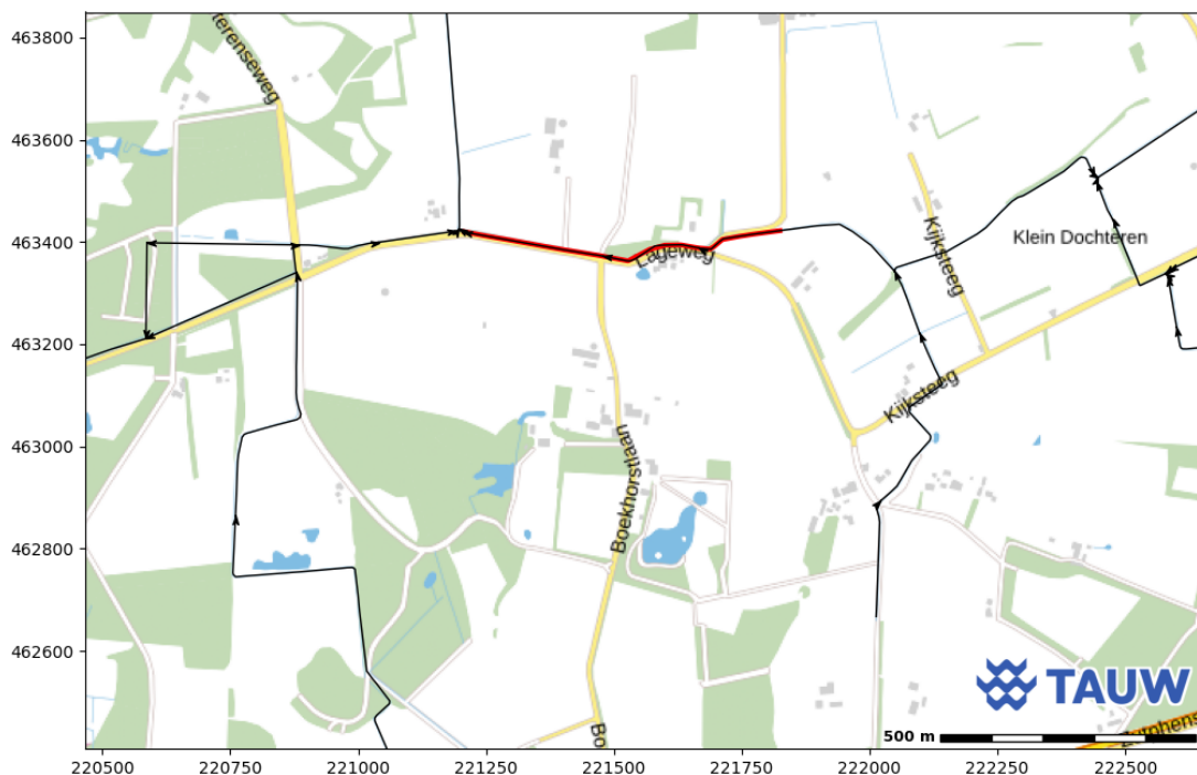
Figuur 5.7 Traject waarover verdieping is opgenomen in DO-modelling
