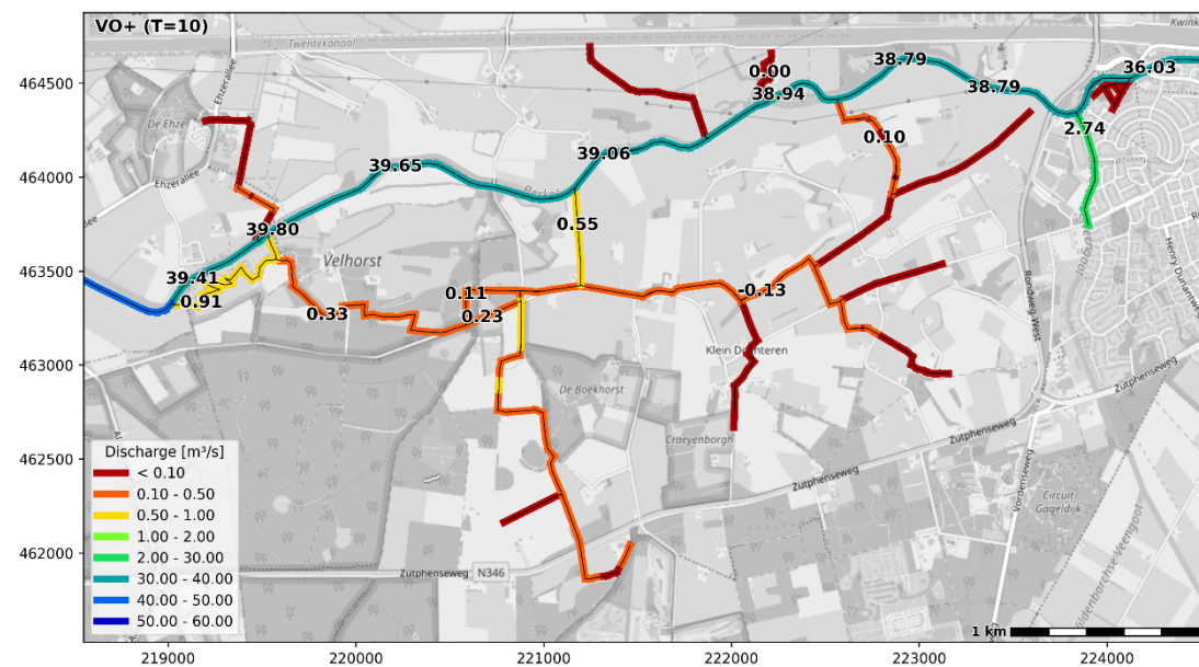
Figuur 4.10 Gemodelleerde debieten in de toekomstige situatie (T=10-situatie)
