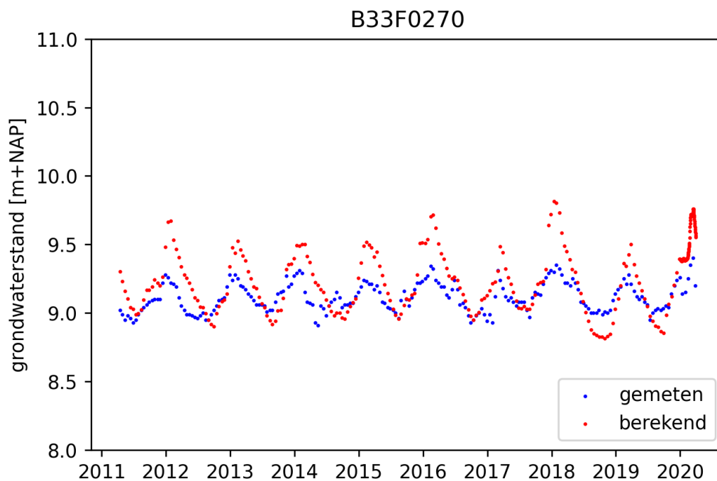
Figuur B2.5 Gemeten en berekende grondwaterstand ter hoogte van peilbuis 'B33F0270'
