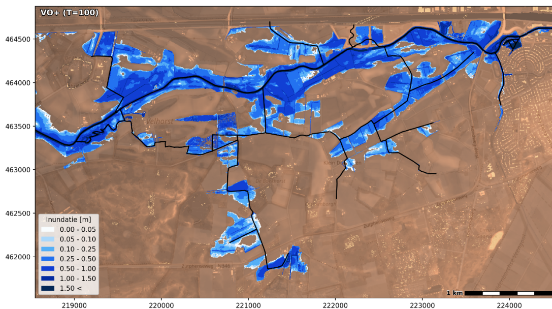
Figuur 4.32 Berekende inundatiediepte in meters ten opzichte van het maaiveld in de T=100-situatie
