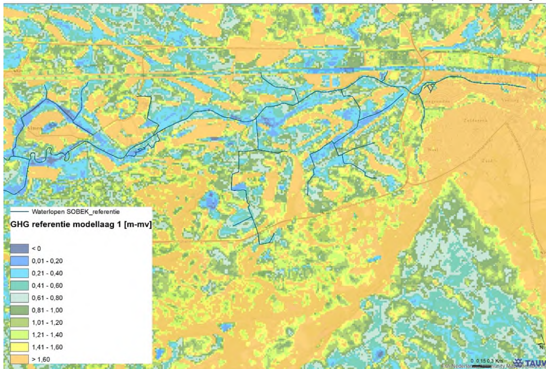
Figuur B3.4 GHG-referentie (m-mv)
