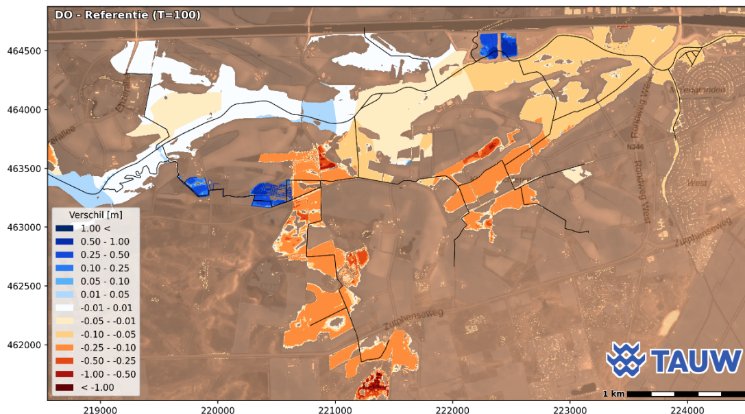
Figuur 5.37 Verschil in inundatiediepte in meters ten opzichte van de referentiesituatie (T=100-situatie)
