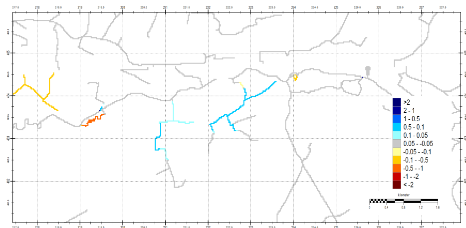
Figuur B4.27 Verschil winterpeil (DO minus referentie)
