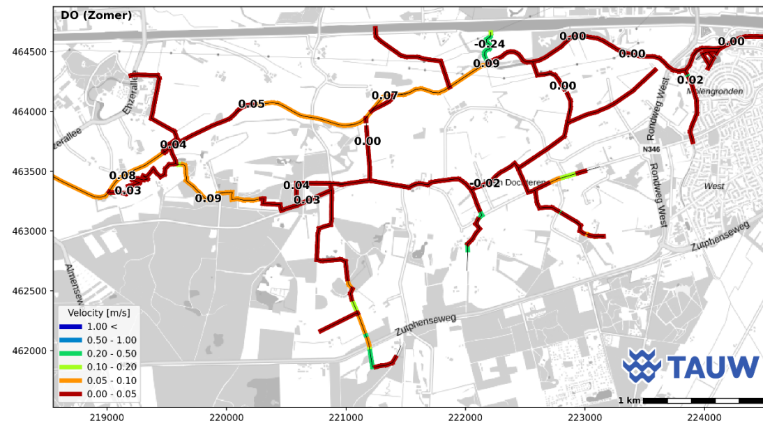
Figuur 5.30 Gemodelleerde stroomsnelheden in de toekomstige situatie (gemiddelde zomersituatie)
