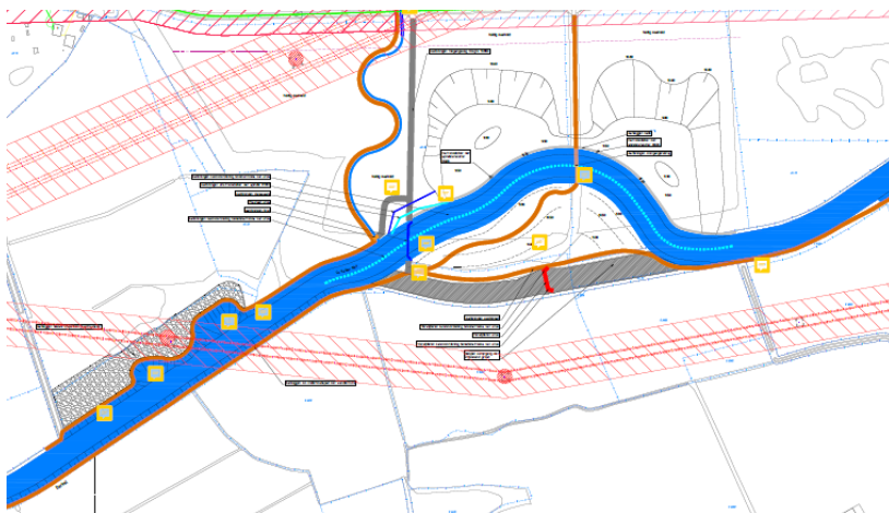
Figuur 4.5 Modelaanpassing #2 Verplaatsen hoofdloop en stuw Hoge Weide
