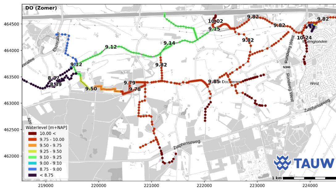
Figuur 5.18 Gemodelleerde waterstand in de toekomstige situatie in m + NAP (gemiddelde zomersituatie)
