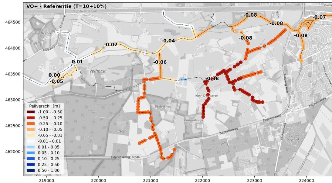
Figuur 4.21 Verschil in waterstanden (en tevens verschil in waterdiepte) ten opzichte van de referentiesituatie in meters (T=10+10 %-situatie)
