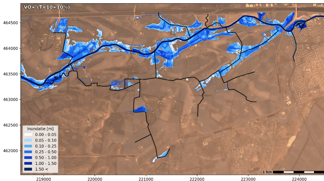
Figuur 4.29 Berekende inundatiediepte in meters ten opzichte van het maaiveld in de T=10+10 %-situatie
