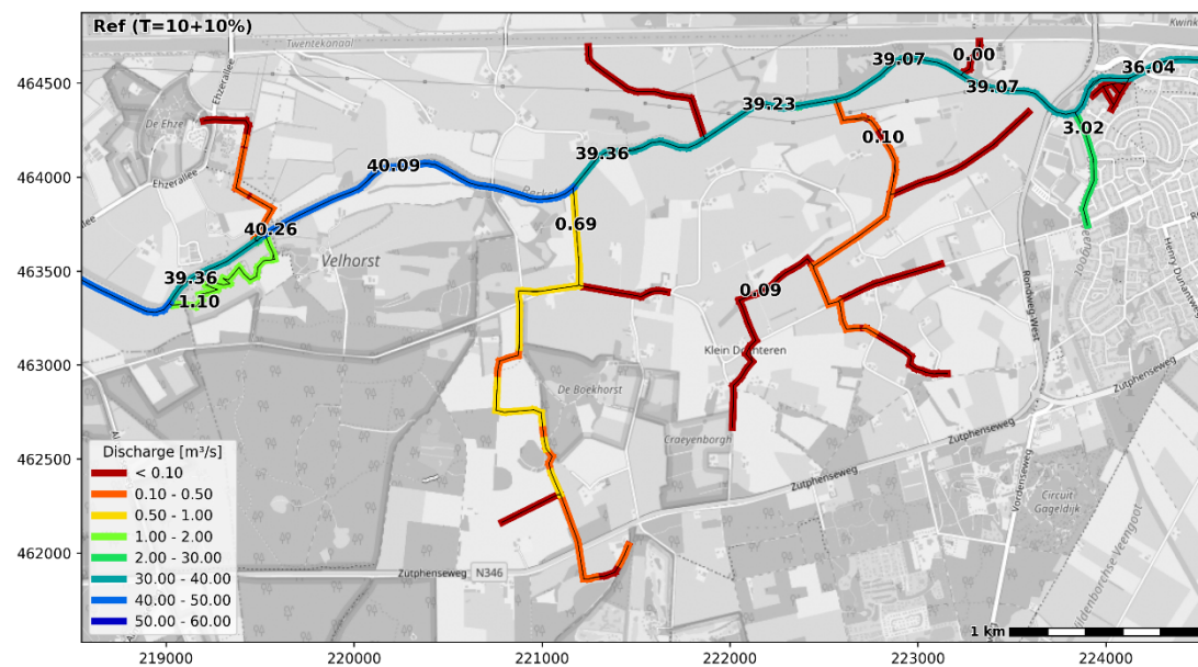
Figuur 3.4 Gemodelleerde debieten in de huidige situatie (T=10+10 %-situatie)
