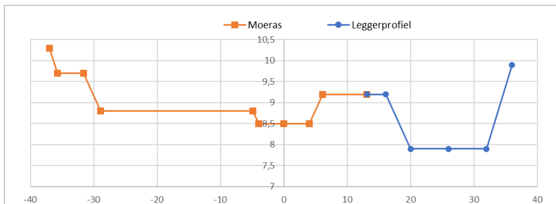
Figuur 5.4 Principeprofiel Staringkoepel
