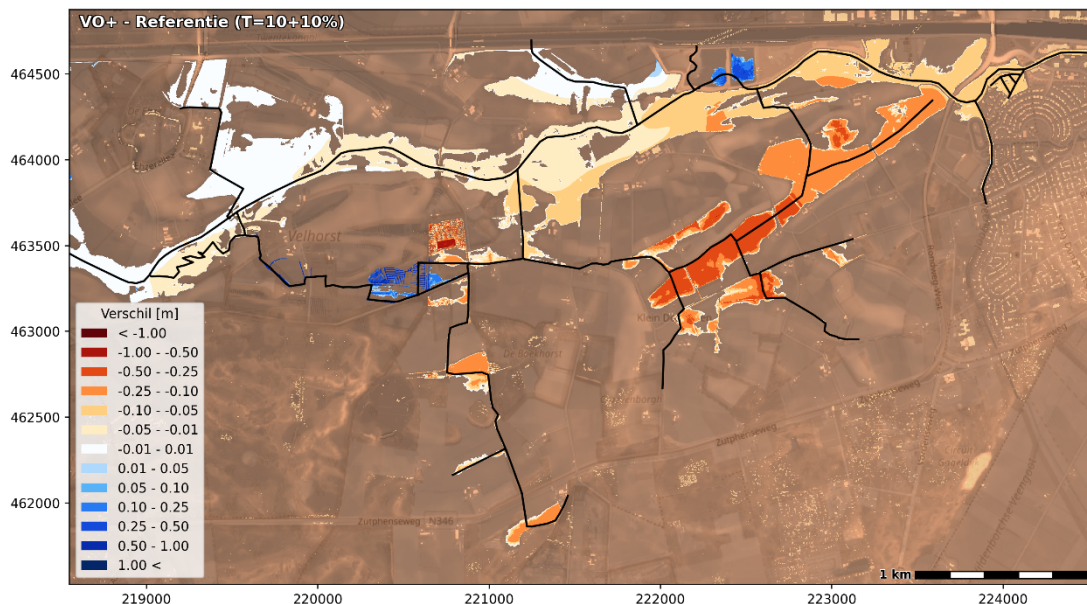
Figuur 4.30 Verschil in inundatiediepte in meters ten opzichte van de referentiesituatie (T=10+10 %-situatie)
