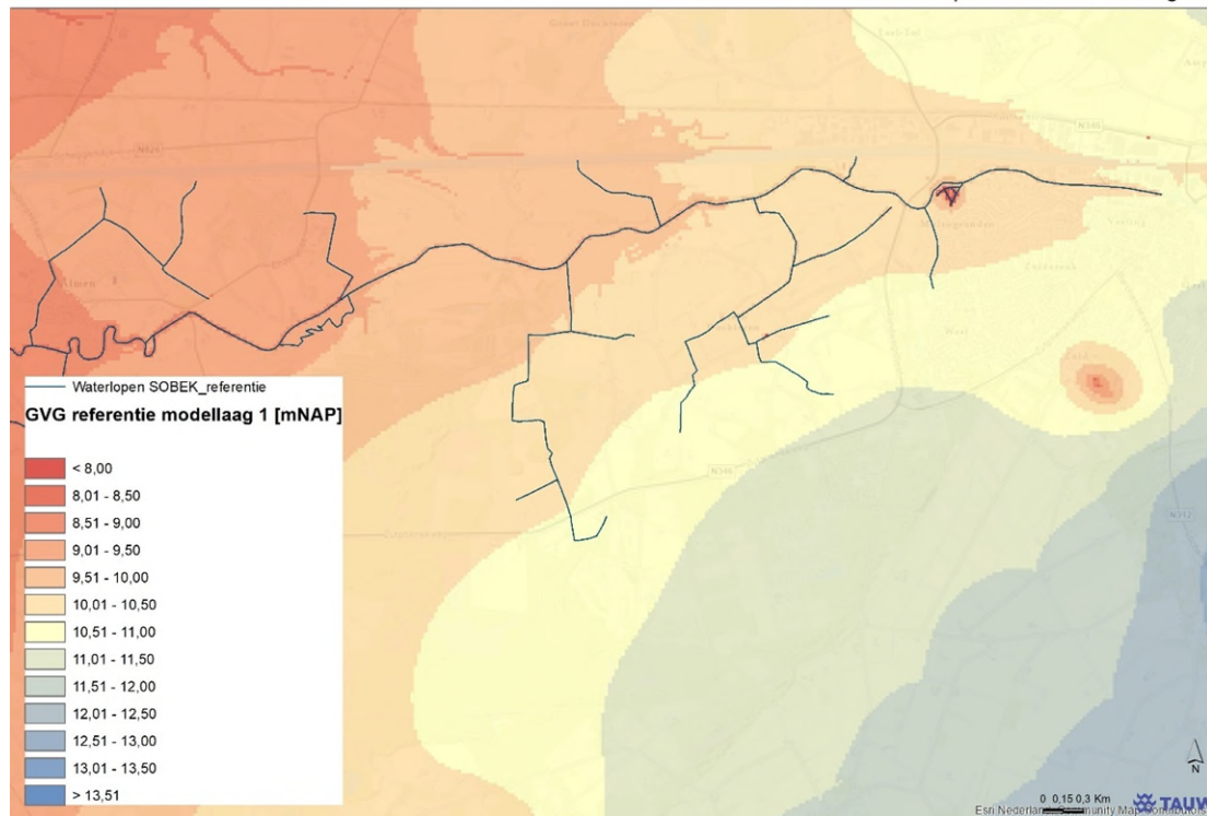
Figuur B3.29 GVG-referentie (mNAP)
