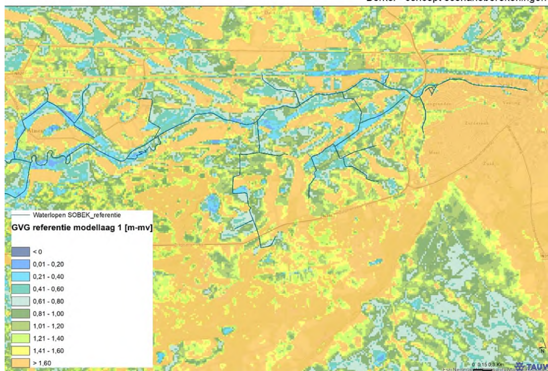
Figuur 3.19 GVG (m-mv) referentiesituatie
