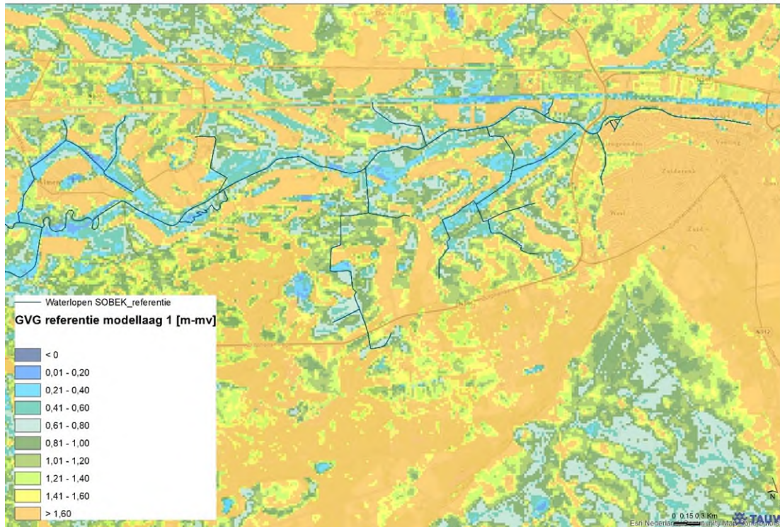
Figuur B3.23 GVG-referentie (m-mv)
