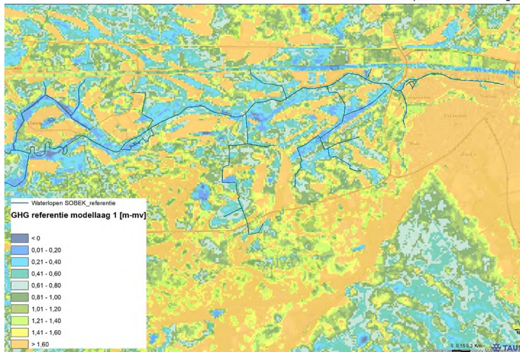
Figuur 3.17 GHG (m-mv) referentiesituatie
