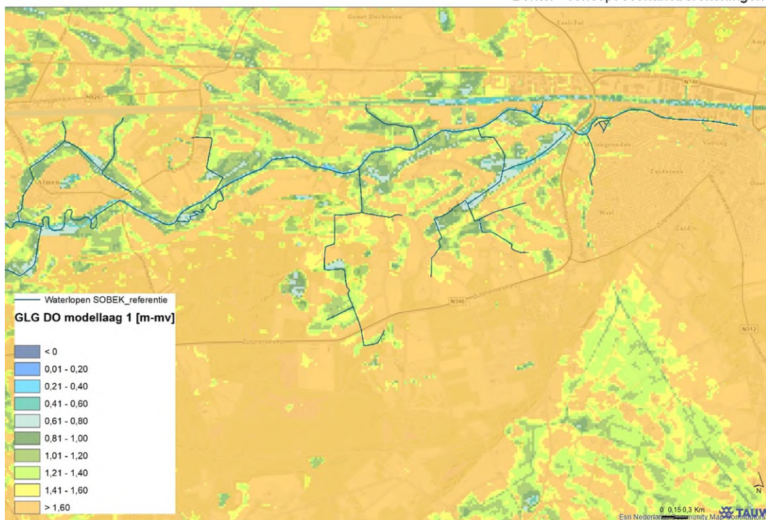
Figuur B3.22 GLG DO (m-mv)
