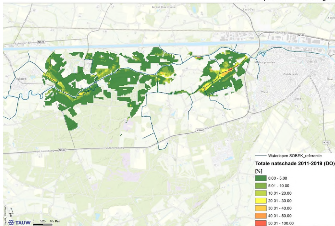
Figuur B5.14 Totale natschade DO in % over periode 2011-2019
