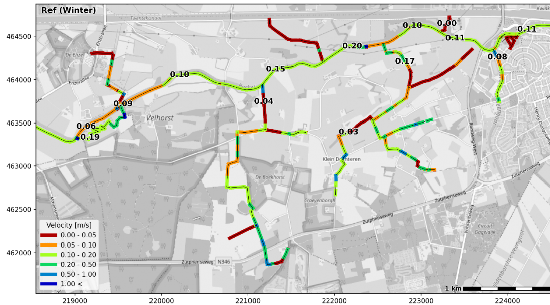
Figuur 3.13 Gemodelleerde stroomsnelheden in de huidige situatie in m/s (gemiddelde wintersituatie)
