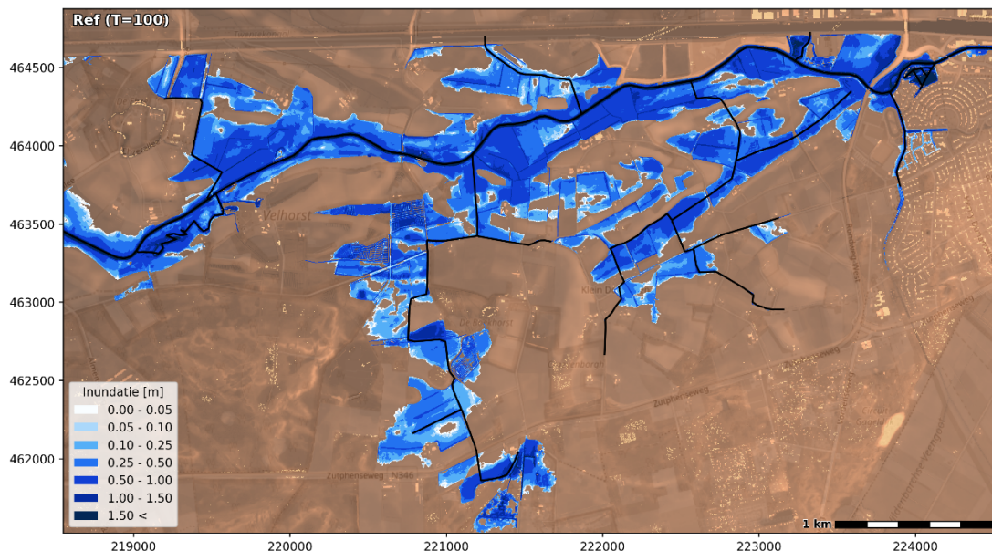
Figuur 3.16 Inundatiediepte in de T=100-situatie in meters ten opzichte van maaiveld
