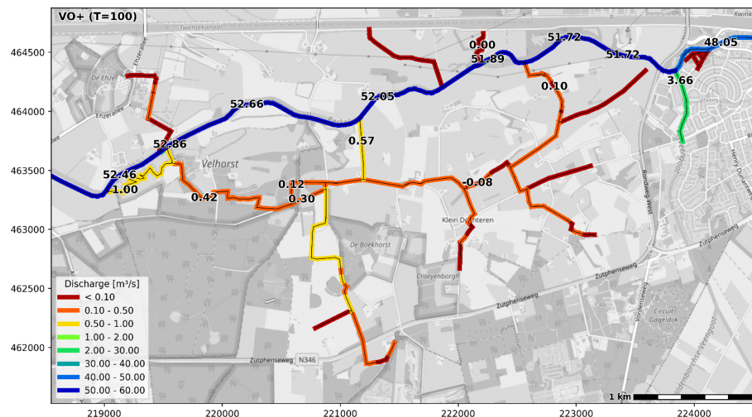
Figuur 4.12 Gemodelleerde debieten in de toekomstige situatie (T=100-situatie)
