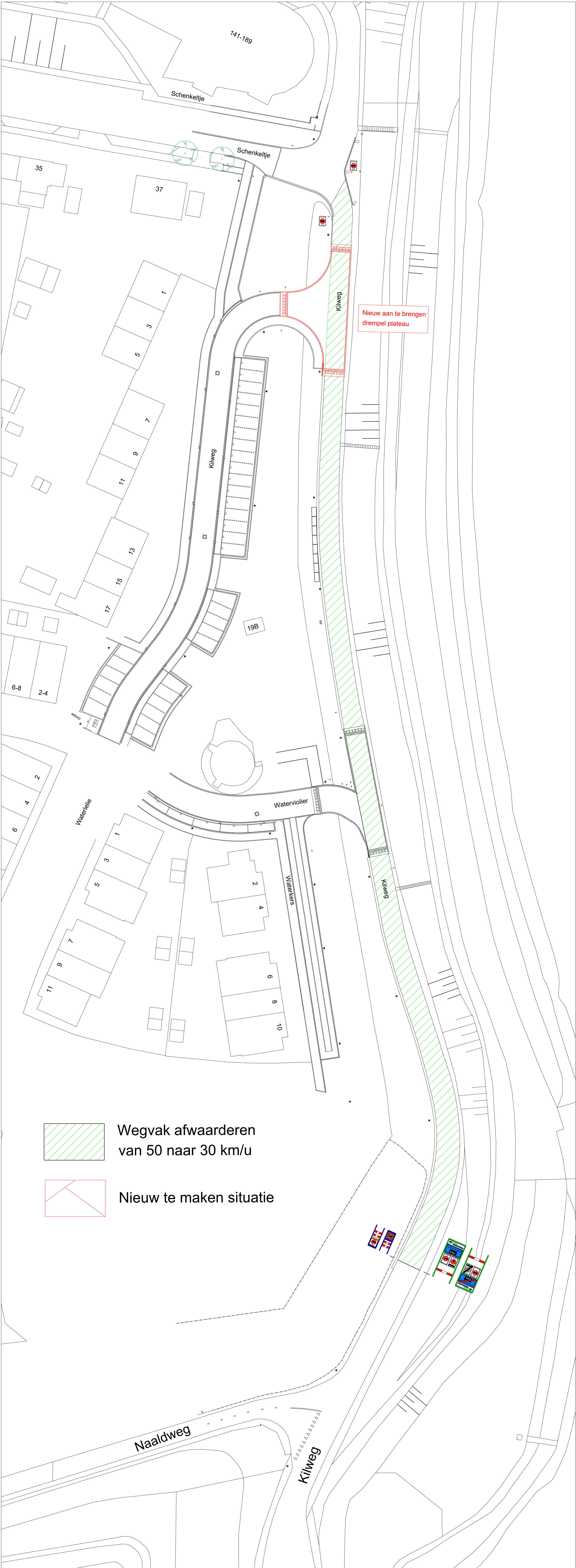
Nieuwe situatie Kilweg (tussen Schenkeltje en Naaldweg)
