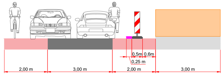
Dwarsdoorsnede A-A
