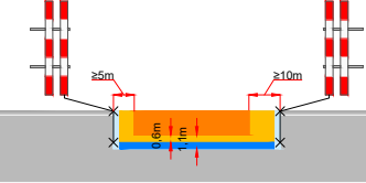
Werkvakindeling ETW
