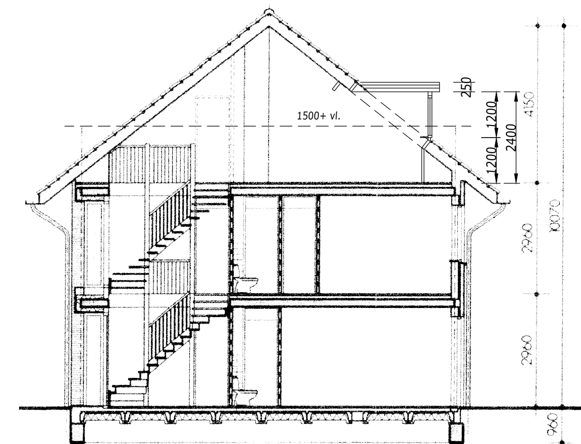
DOORSNEDE GEWIJZIGD
