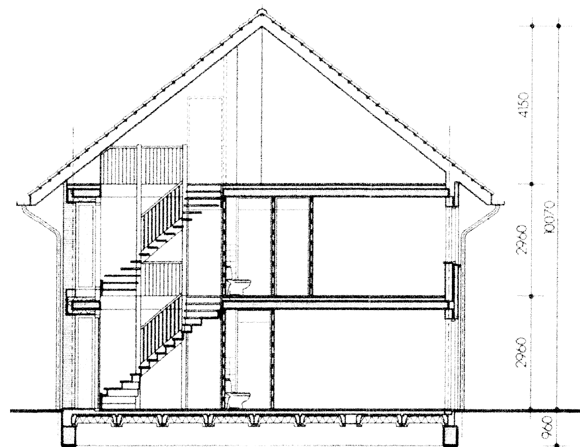
DOORSNEDE BESTAAND
