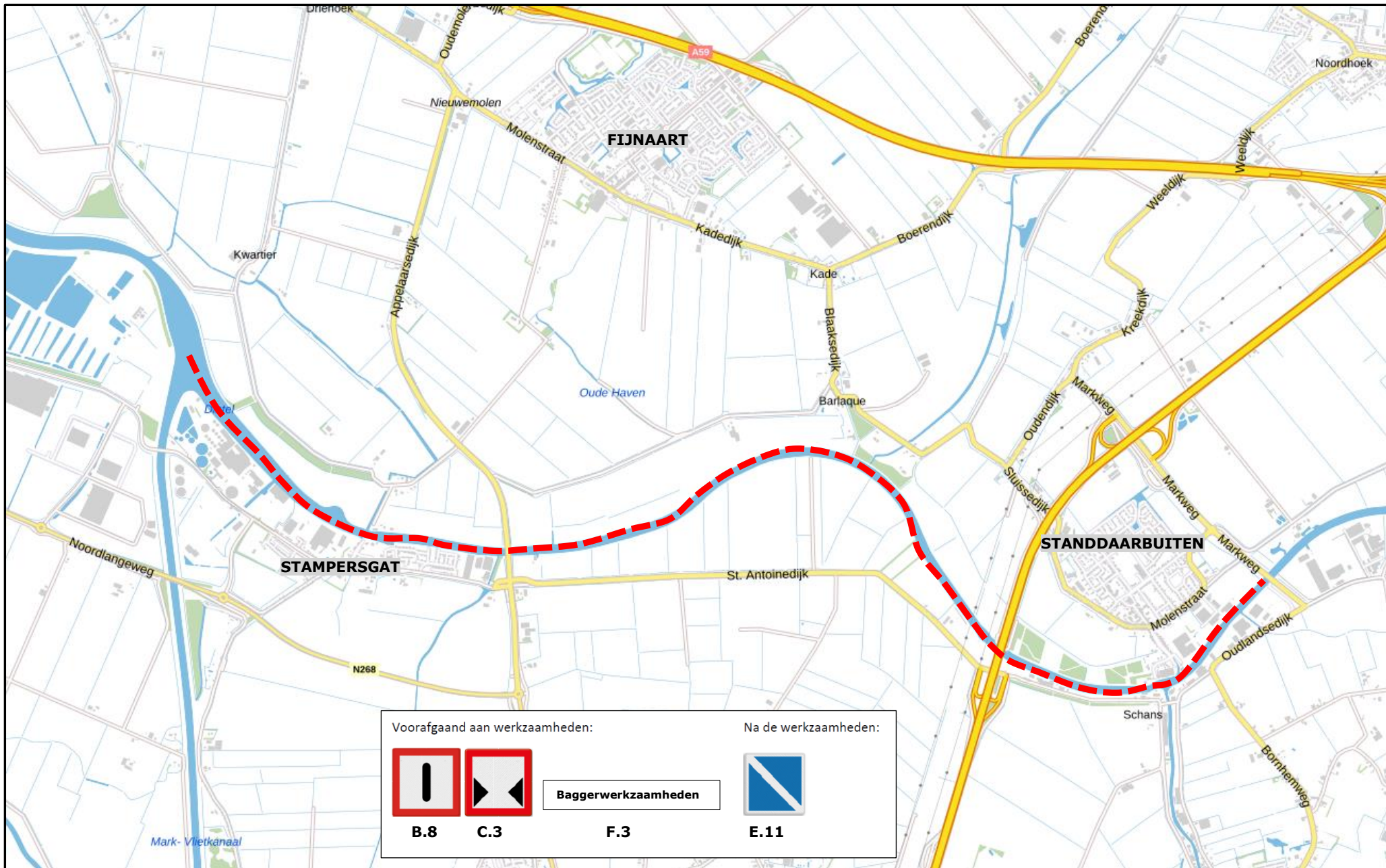
715057-B overzichtstekening bagger traject C – aanbrengen scheepvaarttekens
