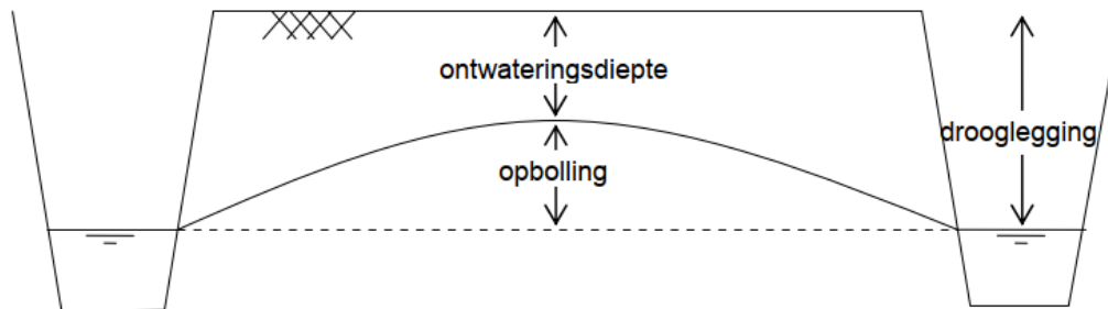
Figuur 13 Ontwateringsdiepte
