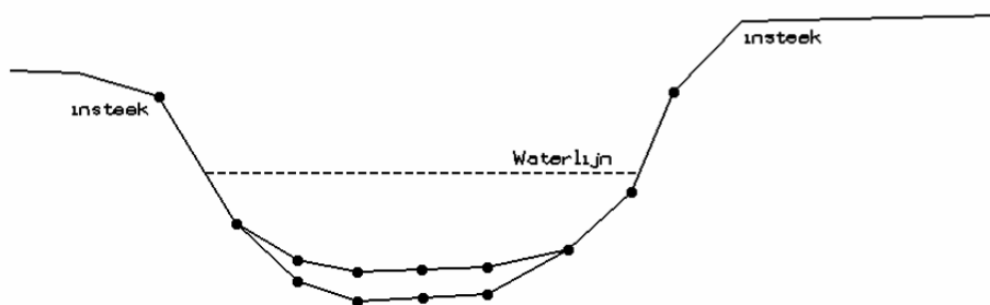
Figuur : Meting bovenkant losse bodem (modder) en vaste bodem
