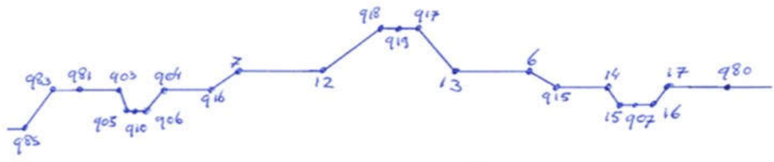
Klei profiel met voor- en achterlandverbetering + Zandontlasting achterland
