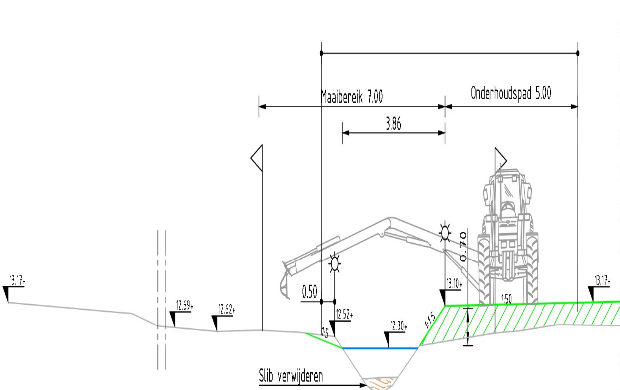
10.00-NAP Dwarsprofiel Q-Q SCHAAL 1:100
