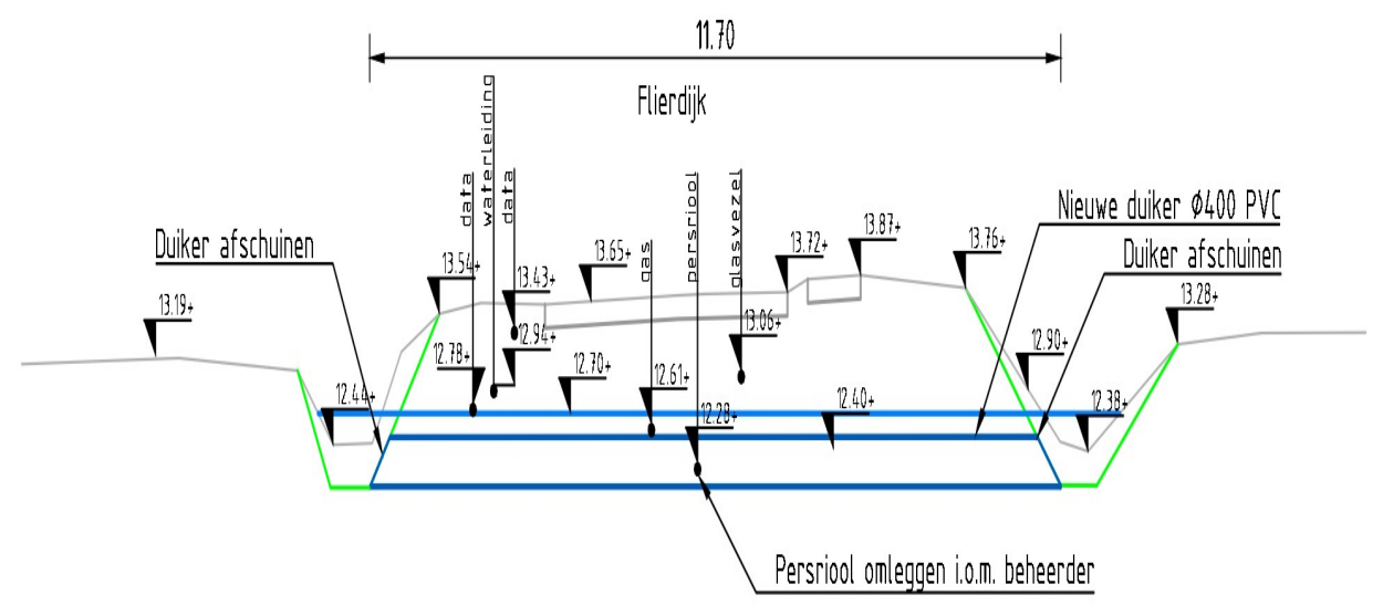
Dwarsprofiel duiker 16 SCHAAL 1 : 100
