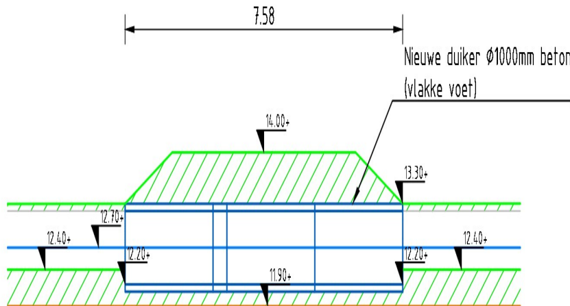
Dwarsprofiel duiker 13 SCHAAL 1 : 100
