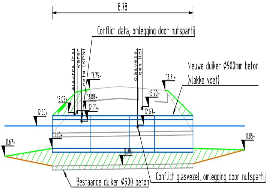
Dwarsprofiel duiker 1 SCHAAL 1 : 100
