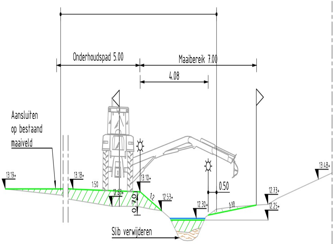
10.00-NAP Dwarsprofiel 0-0 SCHAAL 1:100
