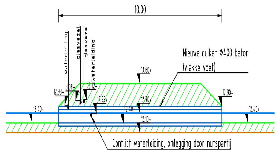
Dwarsprofiel duiker 15 SCHAAL 1 : 100
