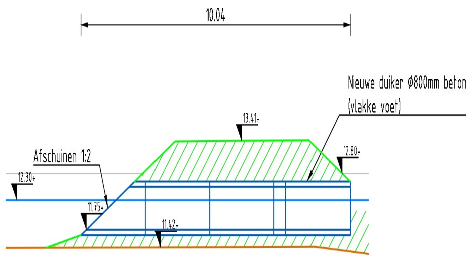
Dwarsprofiel duiker 12 SCHAAL 1 : 100
