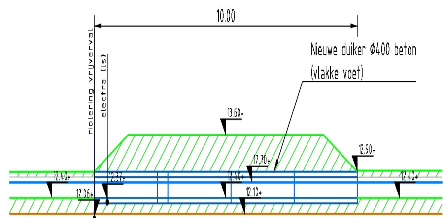
Dwarsprofiel duiker 17 SCHAAL 1 : 100
