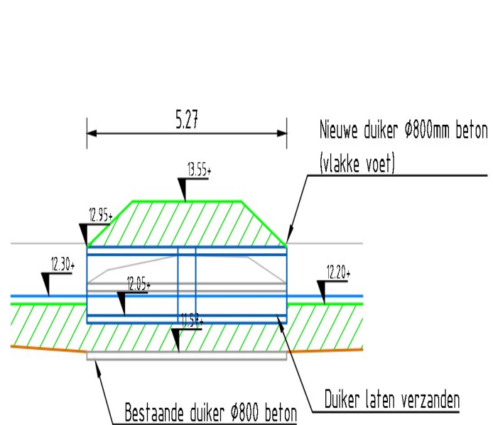
Dwarsprofiel duiker 6 SCHAAL 1 : 100
