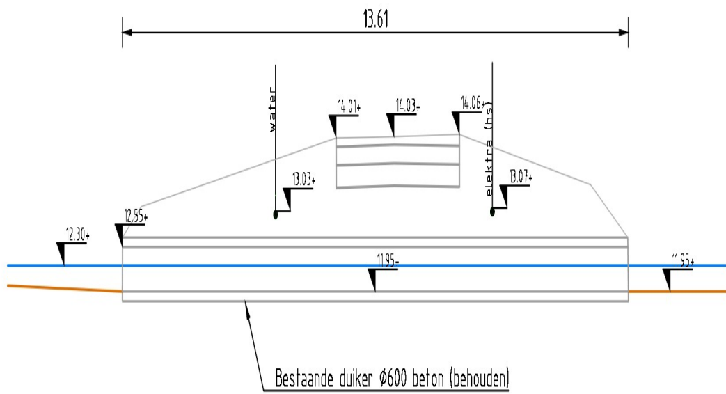
Dwarsprofiel duiker 10 SCHAAL 1 : 100
