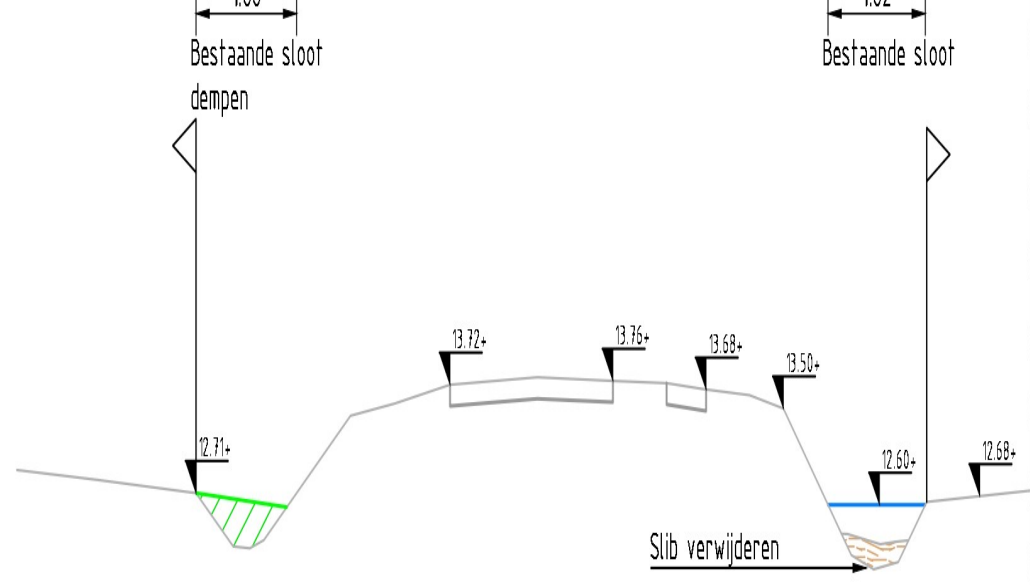
Dwarsprofiel: S-S SCHAAL 1:100
