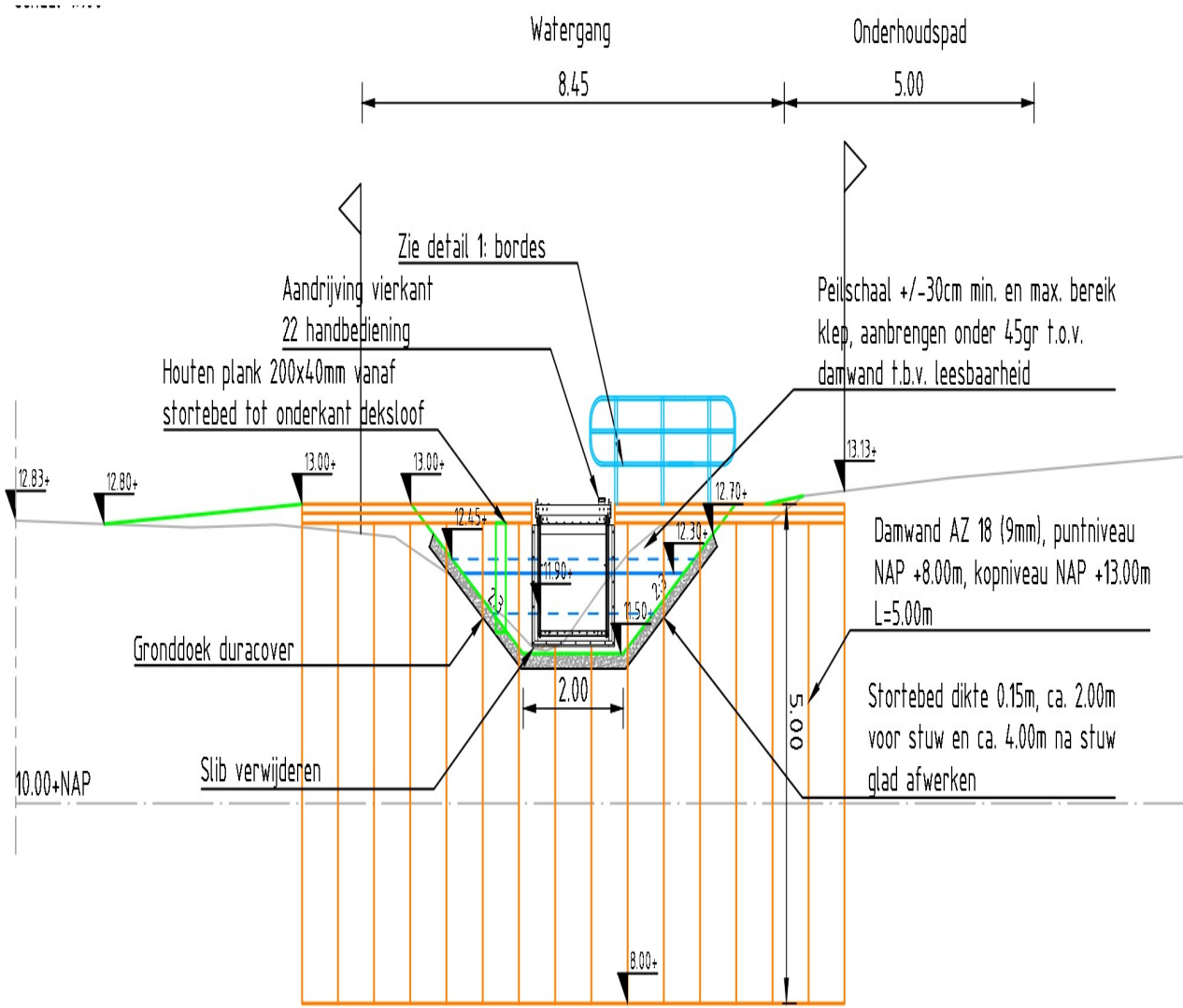
Dwarsprofiel: S-S SCHAAL 1:100
