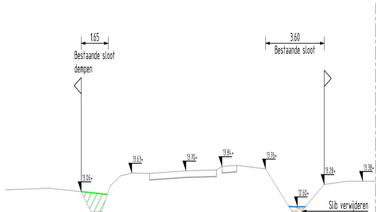
10.00-NAP Dwarsprofiel T-T SCHAAL 1:100
