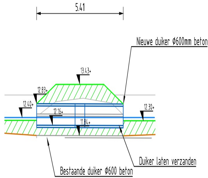
Dwarsprofiel duiker 4 SCHAAL 1 : 100
