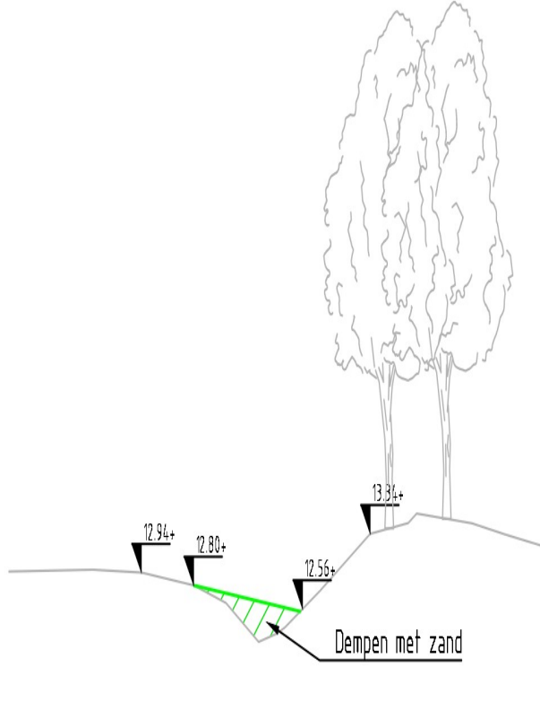
10.00-NAP Dwarsprofiel V-V SCHAAL 1:100
