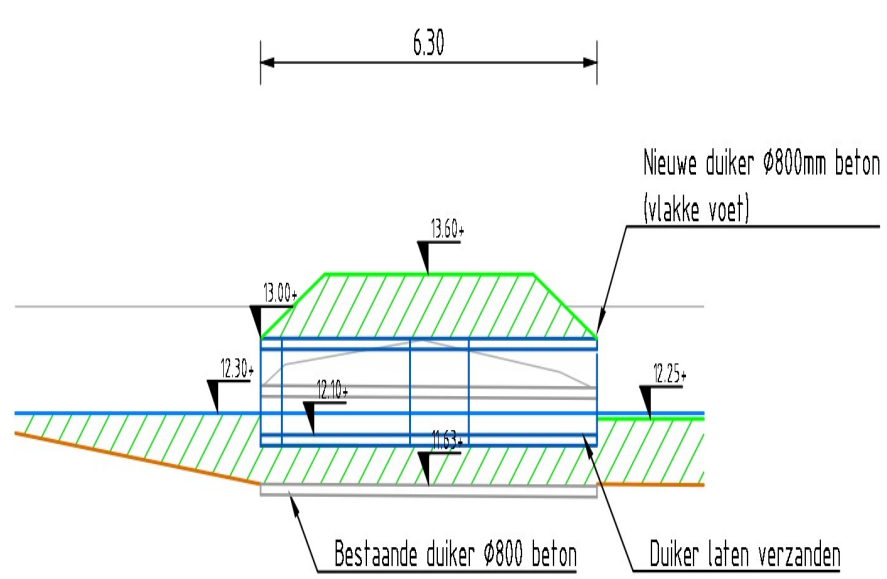
Dwarsprofiel duiker 5 SCHAAL 1 : 100
