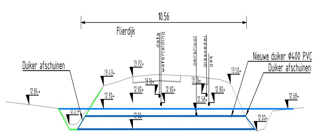
Dwarsprofiel duiker 18 SCHAAL 1 : 100
