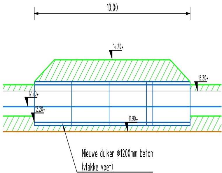
Dwarsprofiel duiker 12 SCHAAL 1 : 100
