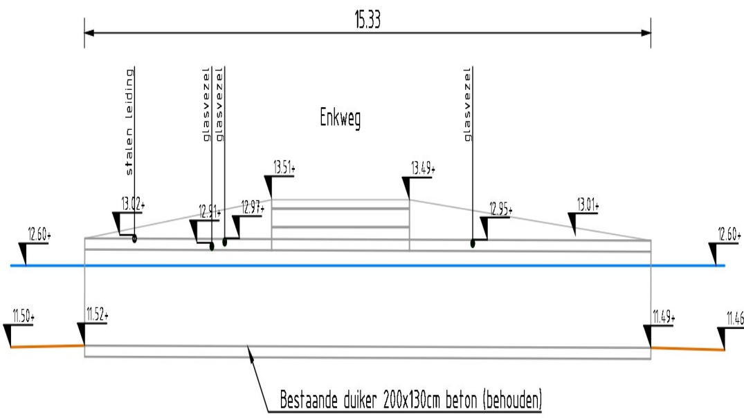
Dwarsprofiel duiker 3 SCHAAL 1 : 100 *Kabels & Leidingen zijn indicatief ingetekend in dit profiel
