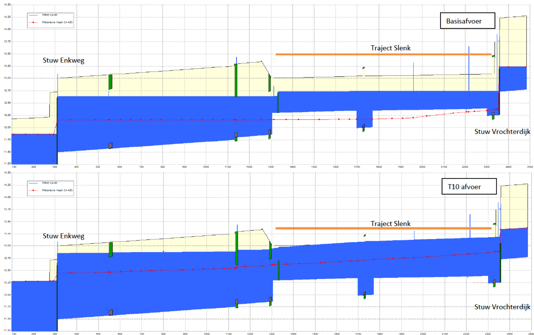
Figuur 12: Lengteprofiel van de Barchemse Veengoot bij basisafvoer (boven) en T10 afvoer (onder). Van Stuw Vrochterdijk rechts t/m stuw Enkweg links. In rood de huidige waterstand te zien in blauw de waterstand na inrichting.
