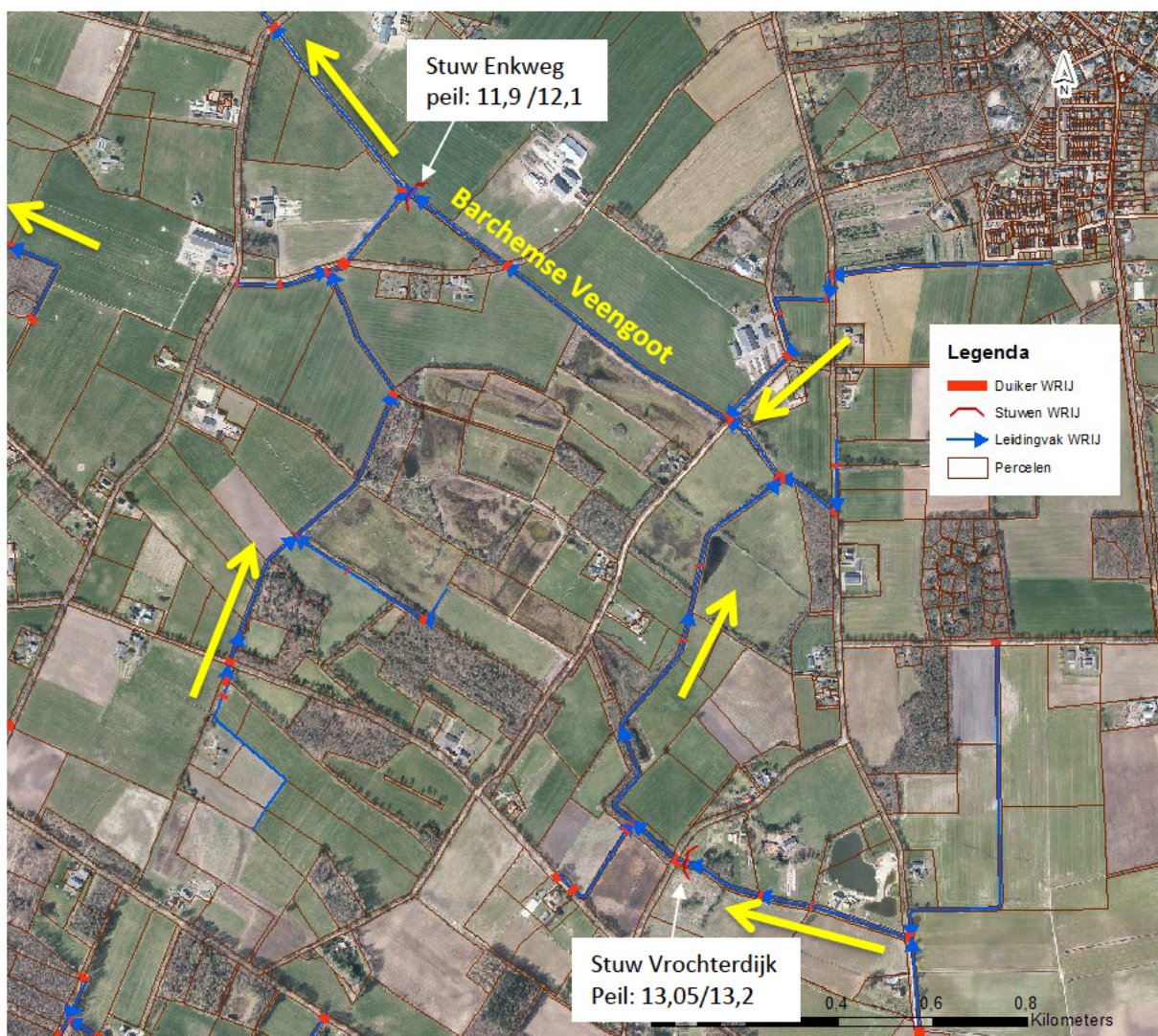
Figuur 4: Afwateringsrichting.
