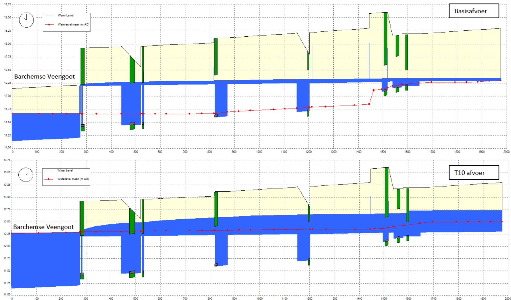
Figuur 11: Lengteprofiel van de westelijke leggerwatergang bij basisafvoer (boven) en T10 afvoer (onder). Van de start van de leggerwatergang, rechts, tot waar de zijtak de Barchemse Veengoot instroomt benedenstrooms van stuw Enkweg. In rood de huidige waterstand te zien in blauw de waterstand na inrichting.
