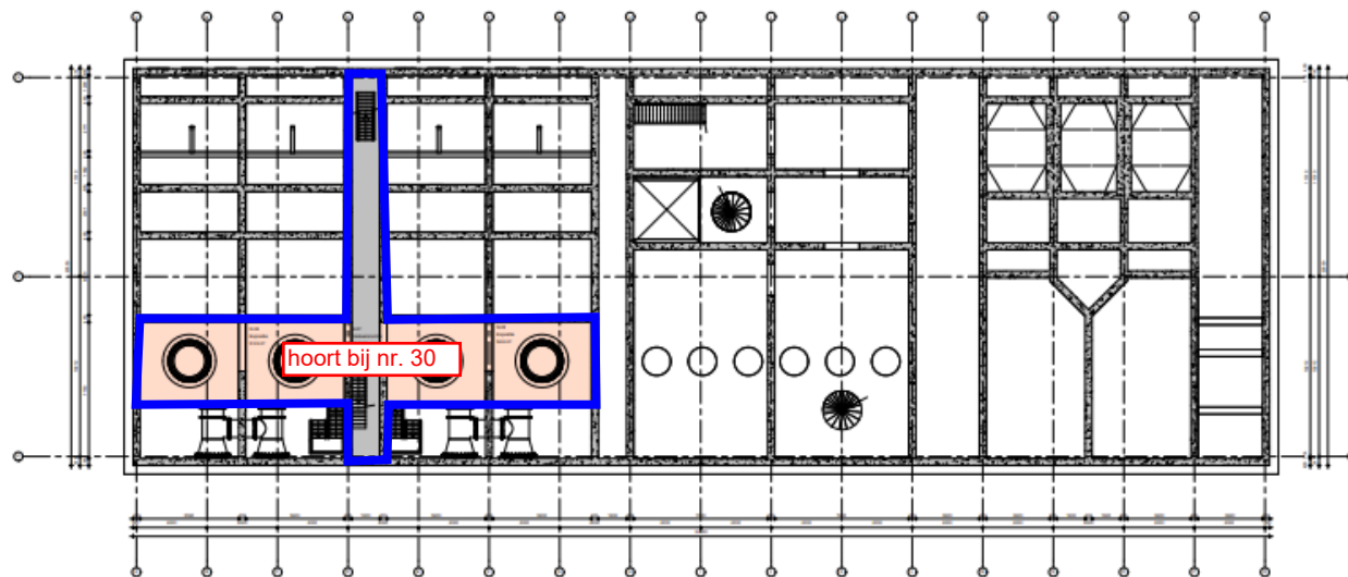
Plattegrond level -2 nieuw
