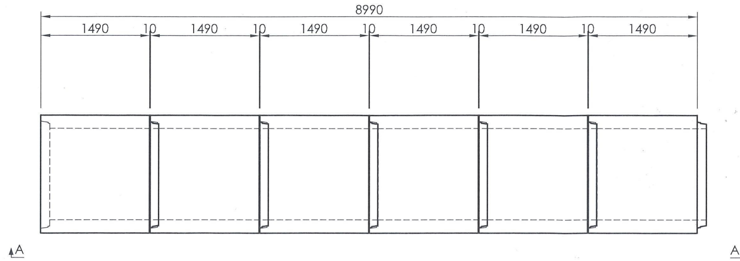
BOVENAANZICHT
