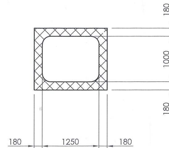
DOORSNEDE B-B
