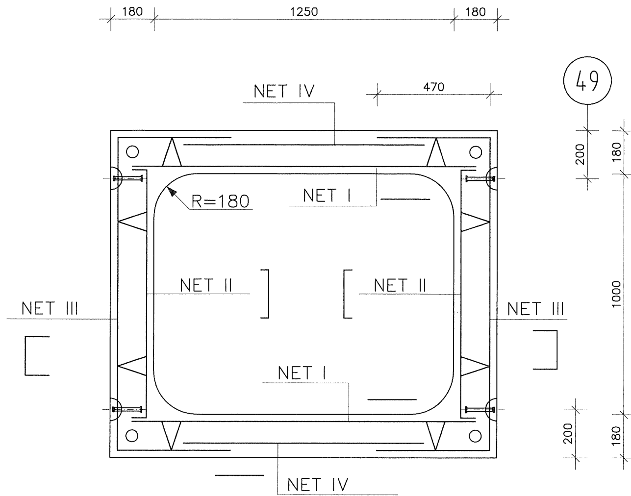
LANGSDOORSNEDE
