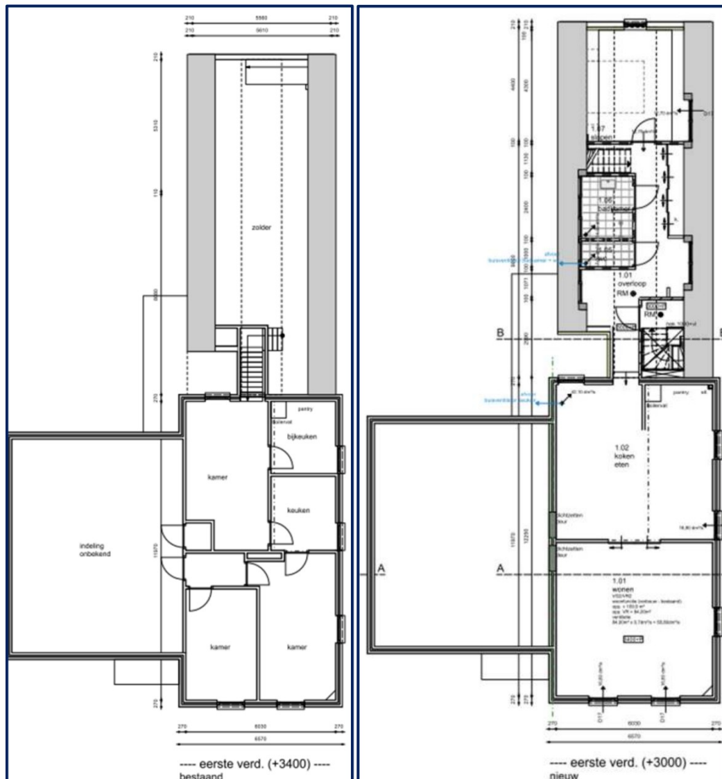
Figuur 4: bestaande en beoogde indeling verdieping bestaand gebouw (bron: Architom Architecten)
