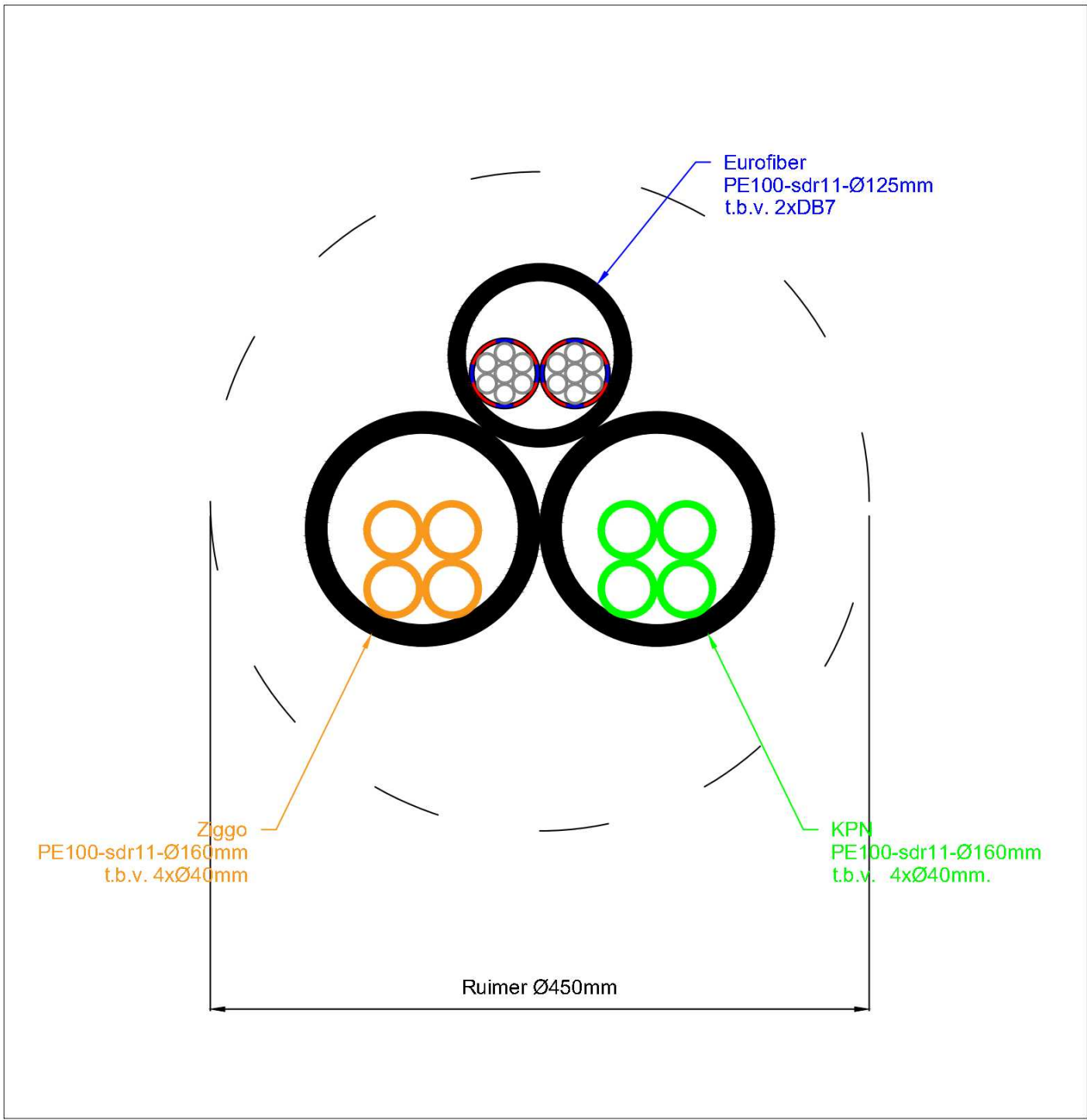
Dwarsdoorsnede buis (schaal 1:4)
