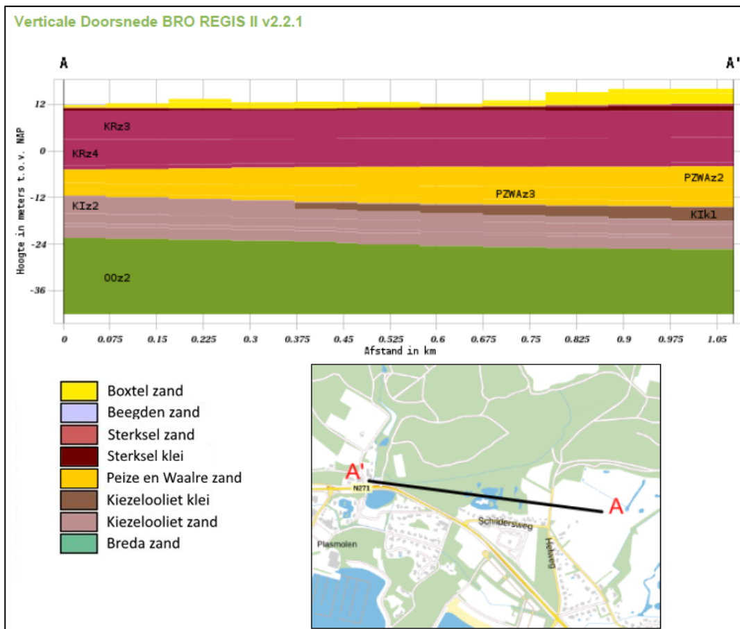
Figuur 2-2: Doorsnede REGIS van de Geuldert tot de zwembijver
