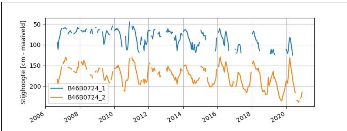
Figuur 2-5: Meetreeks peilbuis B46B0724
