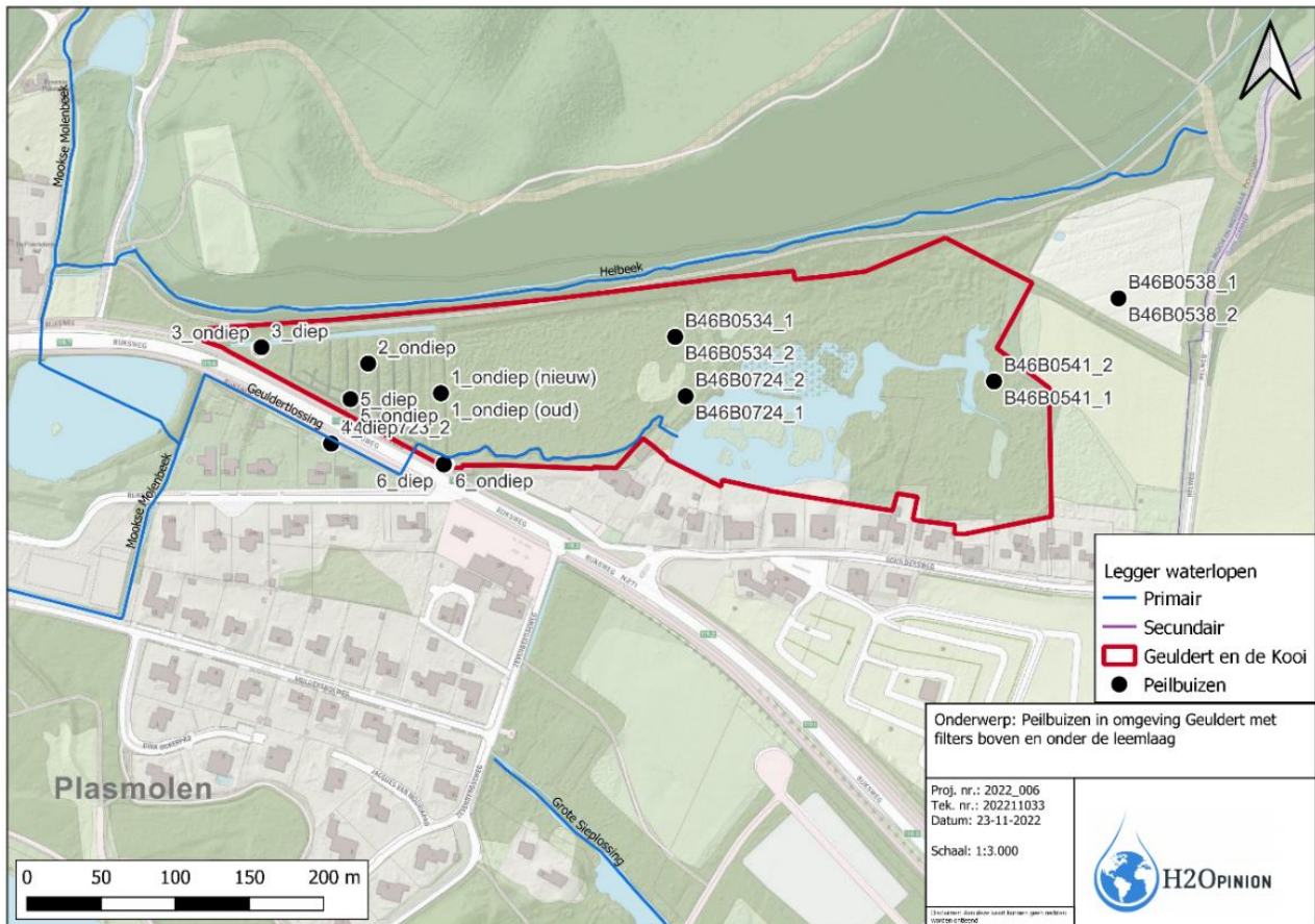
Figuur 2-4: Overzicht locaties peilbuizen in de omgeving
