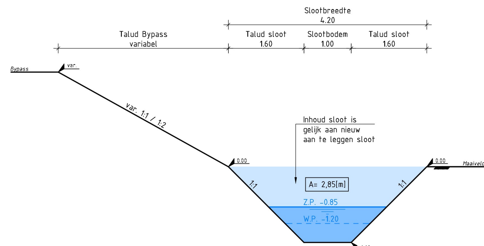
PRINCIPEDOORSNEDE TIJDELIJKE SLOOT SCHAAL 1:50
