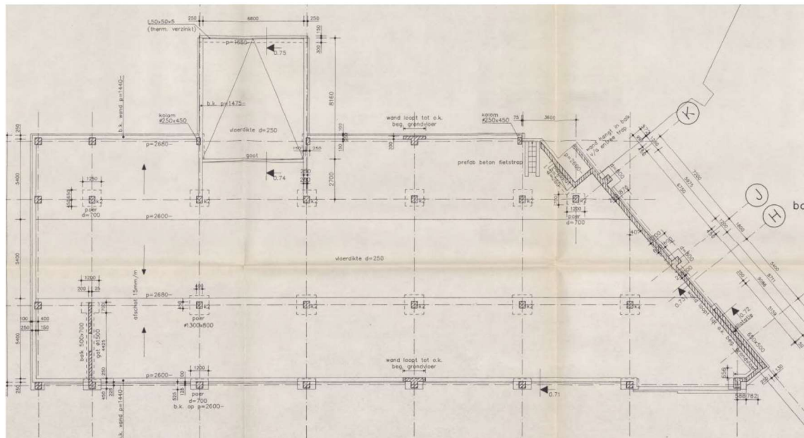
Figuur 10. Overzichtstekening van het souterrain. Het westen is boven. Bron: bouwarchief gemeente Leidschendam-Voorburg.
