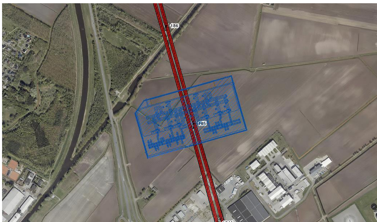
Figuur 8 Luchtfoto met station Musselkanaal 380/110 kV.
