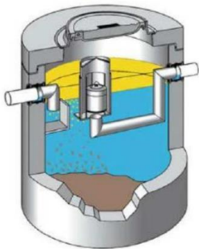
Figuur 17 Olie waterafscheider
