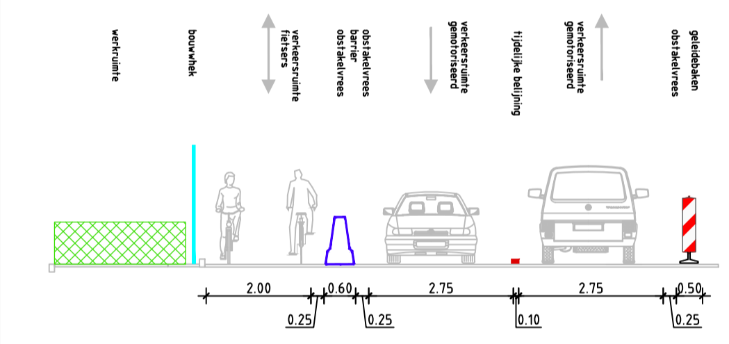
Dwarsprofiel A-A
