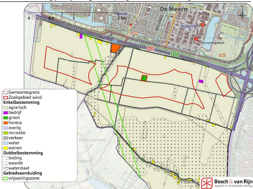
Figuur 17 Bestemmingsplan Rijnenburg, Utrecht (zoekgebied windturbines rood gemarkeerd)
