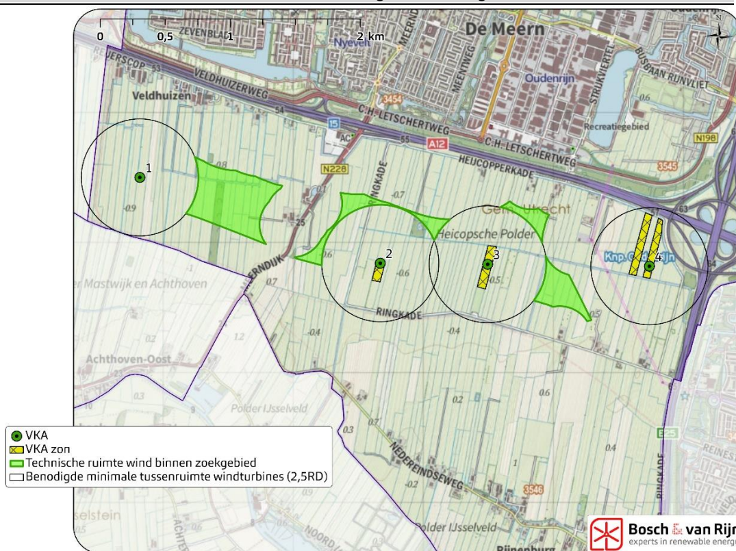
Figuur 108 Technische ruimte windturbines binnen zoekgebied rekening houdend met VKA
