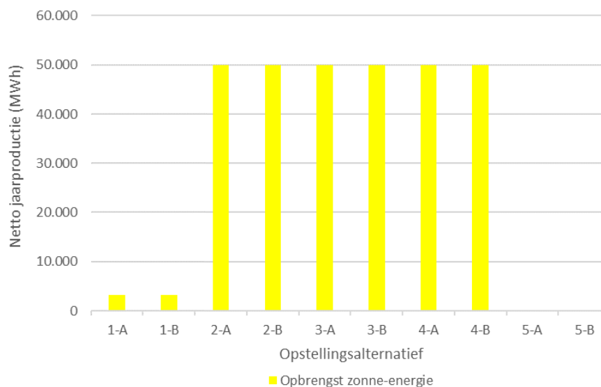
Figuur 88 Nettoproductie van de onderzochte alternatieven zon.
