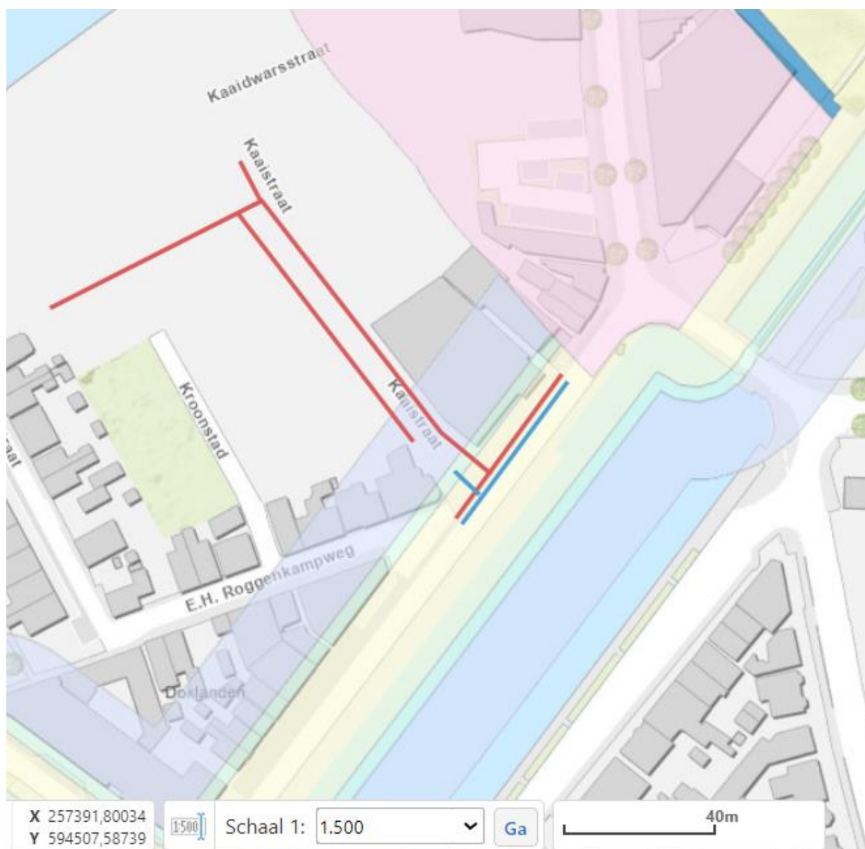
Figuur 1: De rode lijn geeft globaal de locatie weer van de aan te leggen leiding. De blauwe lijn geeft globaal de locatie weer van de te verwijderen leiding. De gele, groene en paarse vlakken geven beperkingengebied I, II en III weer van een regionale waterkering.
