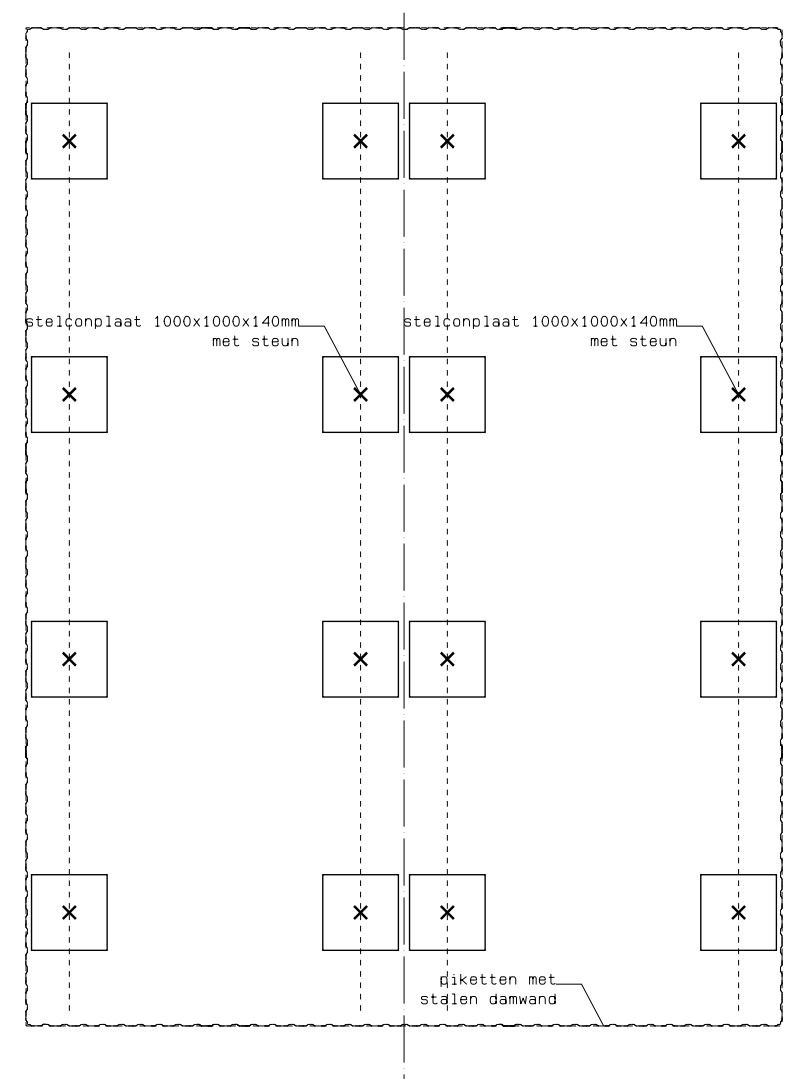
principe fundering
