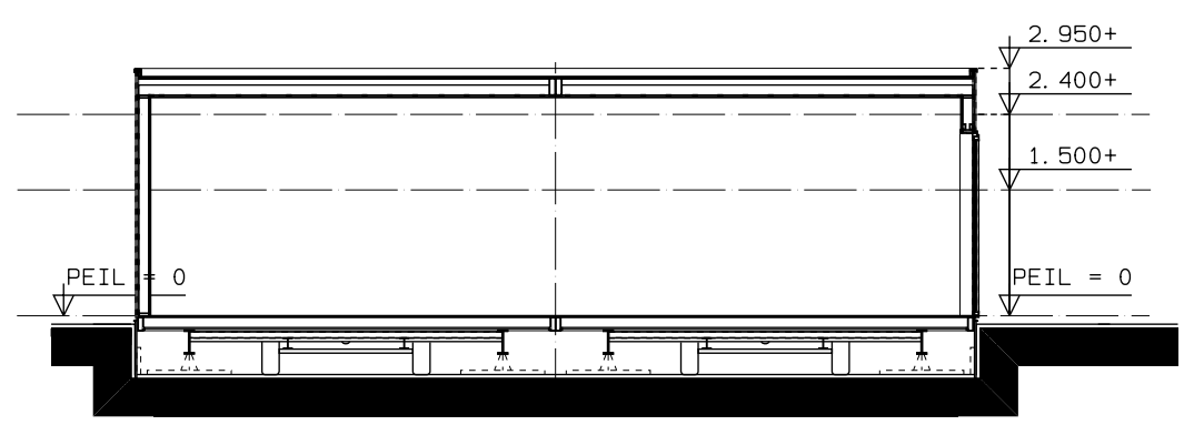
doorsnede A-A
