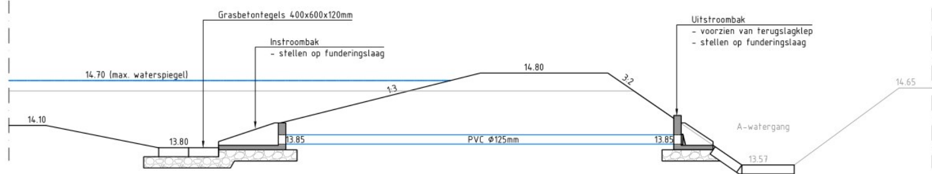
Detail vertraagde afvoer retentievoorziening - A-watergang Schaal 150
