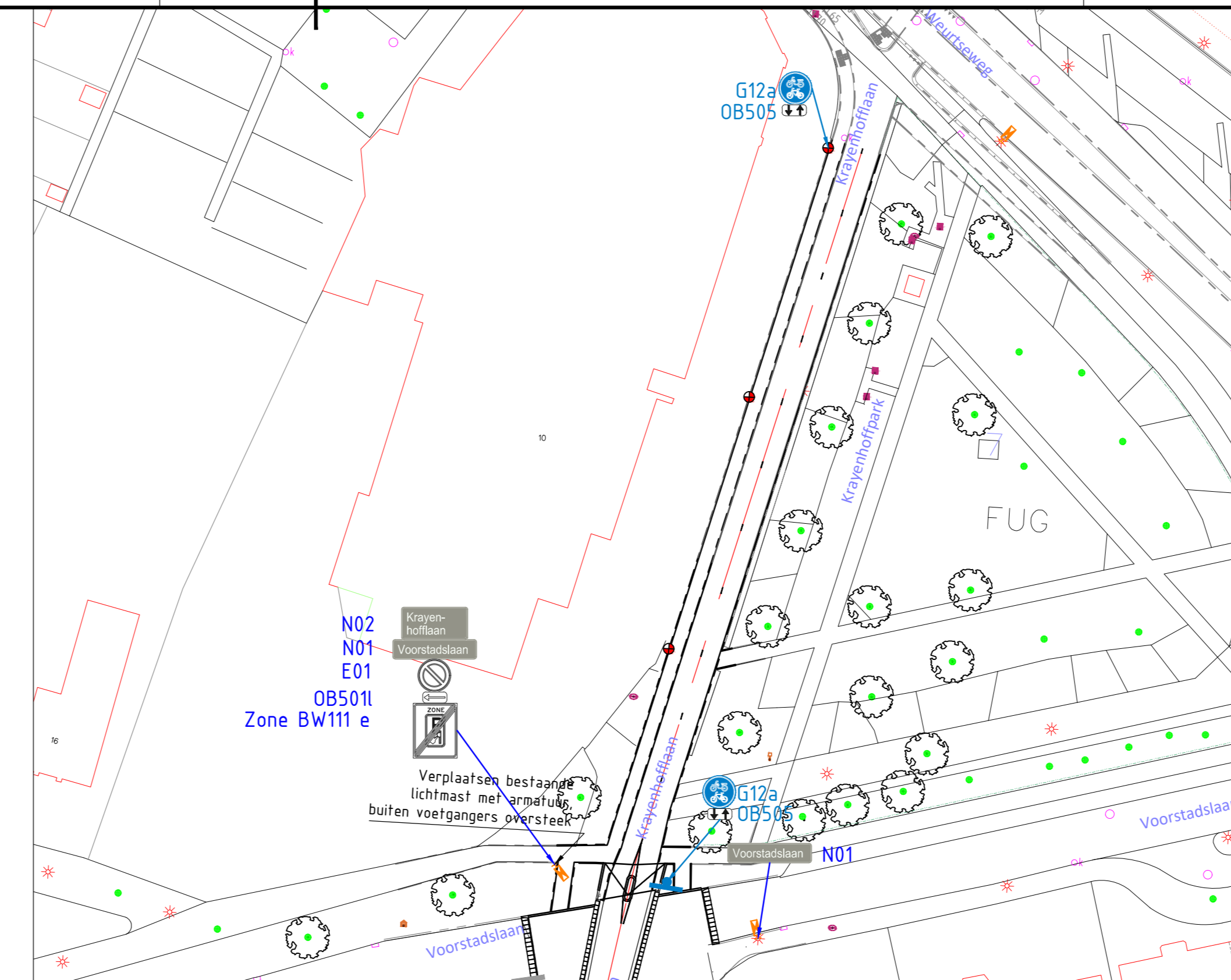
Situatie Krayenhofflaan fietspad Schaal 1:500
