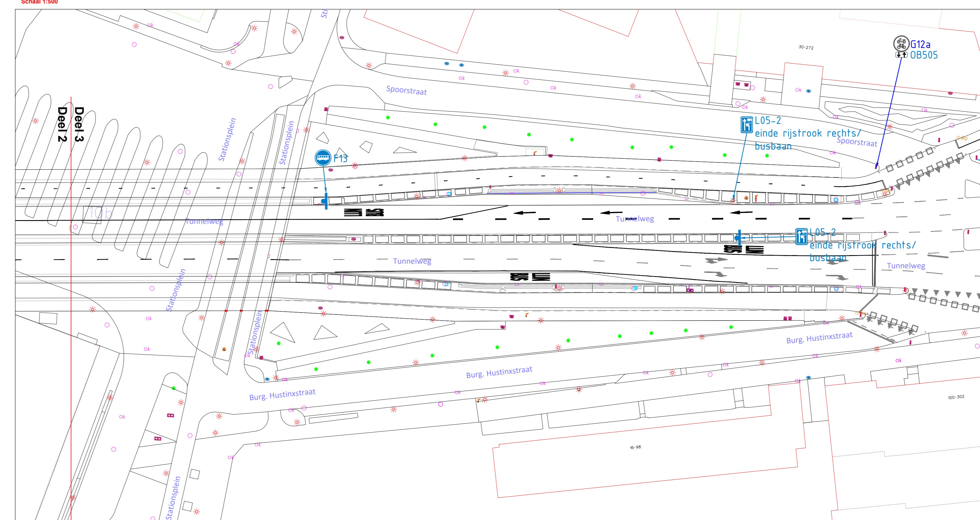
Situatie deel 3 Schaal 1:500
