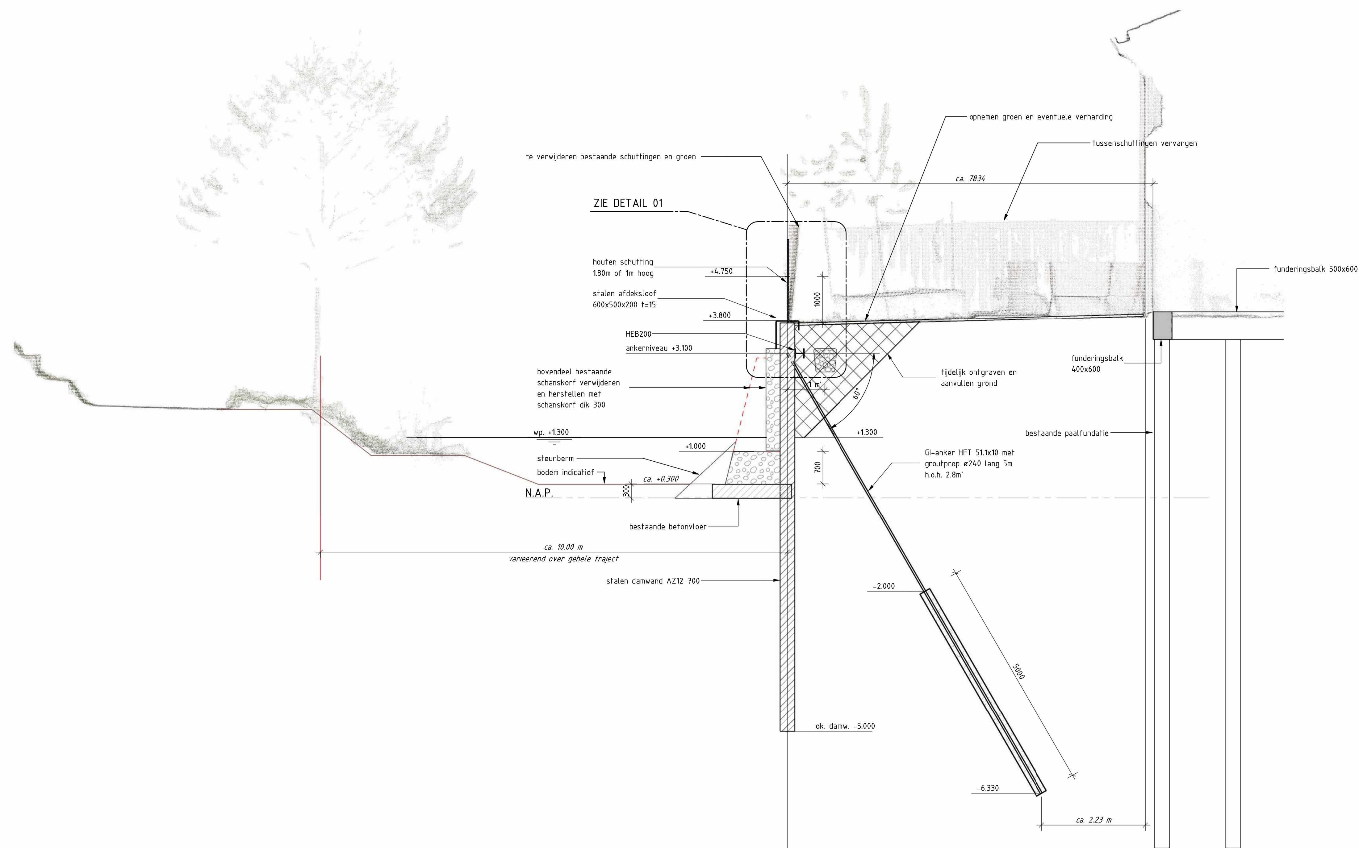
DOORSNEDE A-A SCHAAL: 1 : 50
