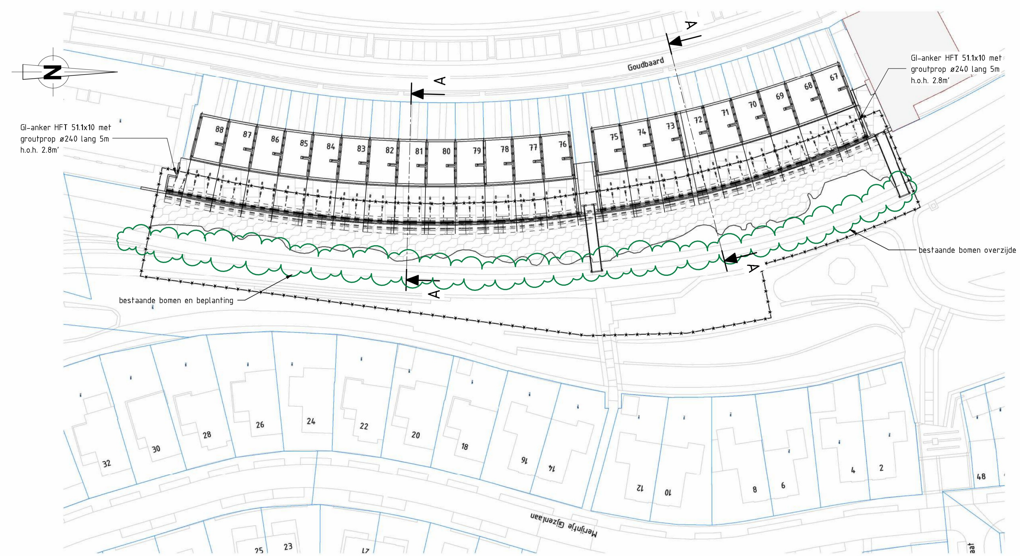
BOVENAANZICHT SCHAAL: 1 : 500
