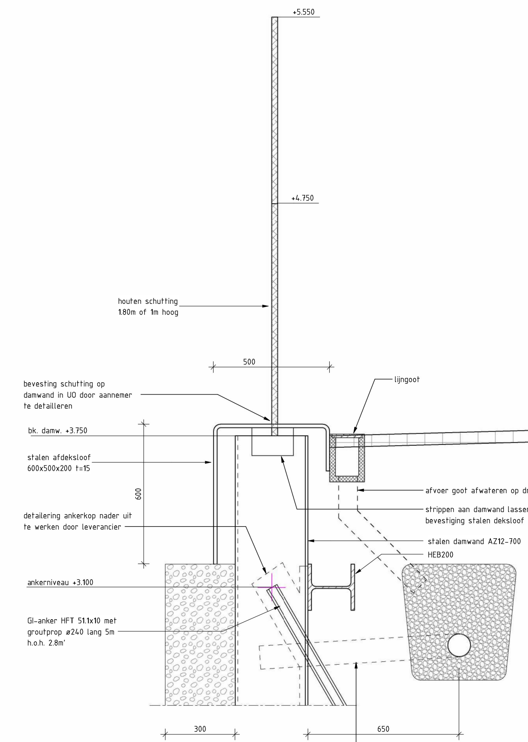
DETAIL 01 SCHAAL: 1 : 10
