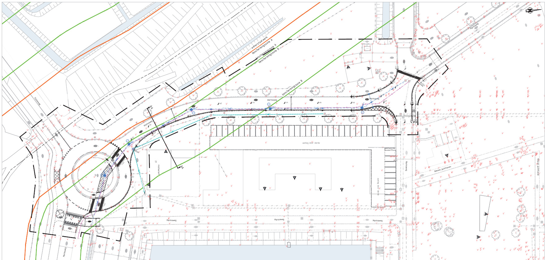
Bovenaanzicht
