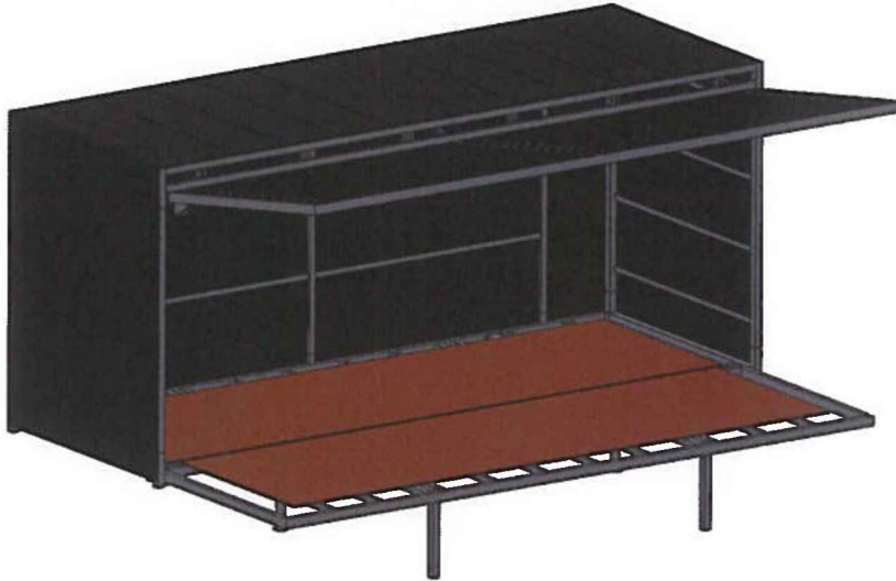
Figuur 14: Vereenvoudigd rekenmodel van de podiumwagen
