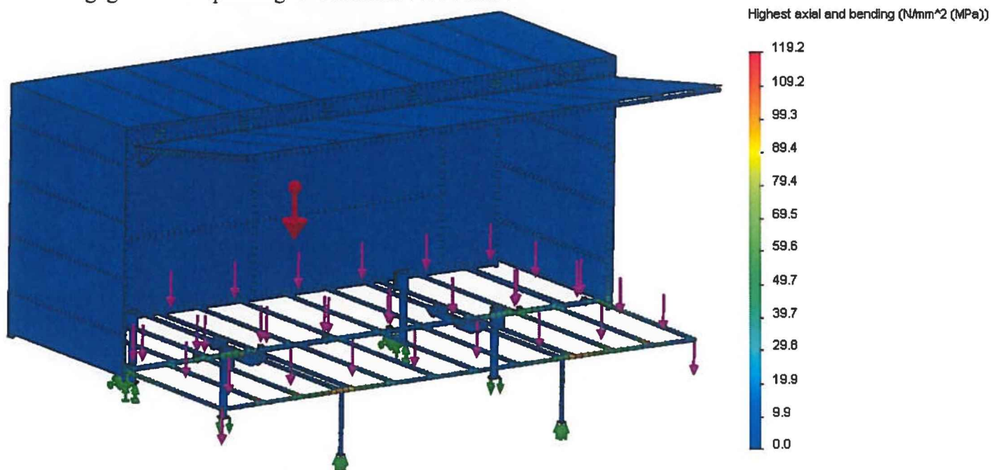
Figuur 21: Optredende spanning in de profielen van de podiumwagen bij de vloerbelasting
