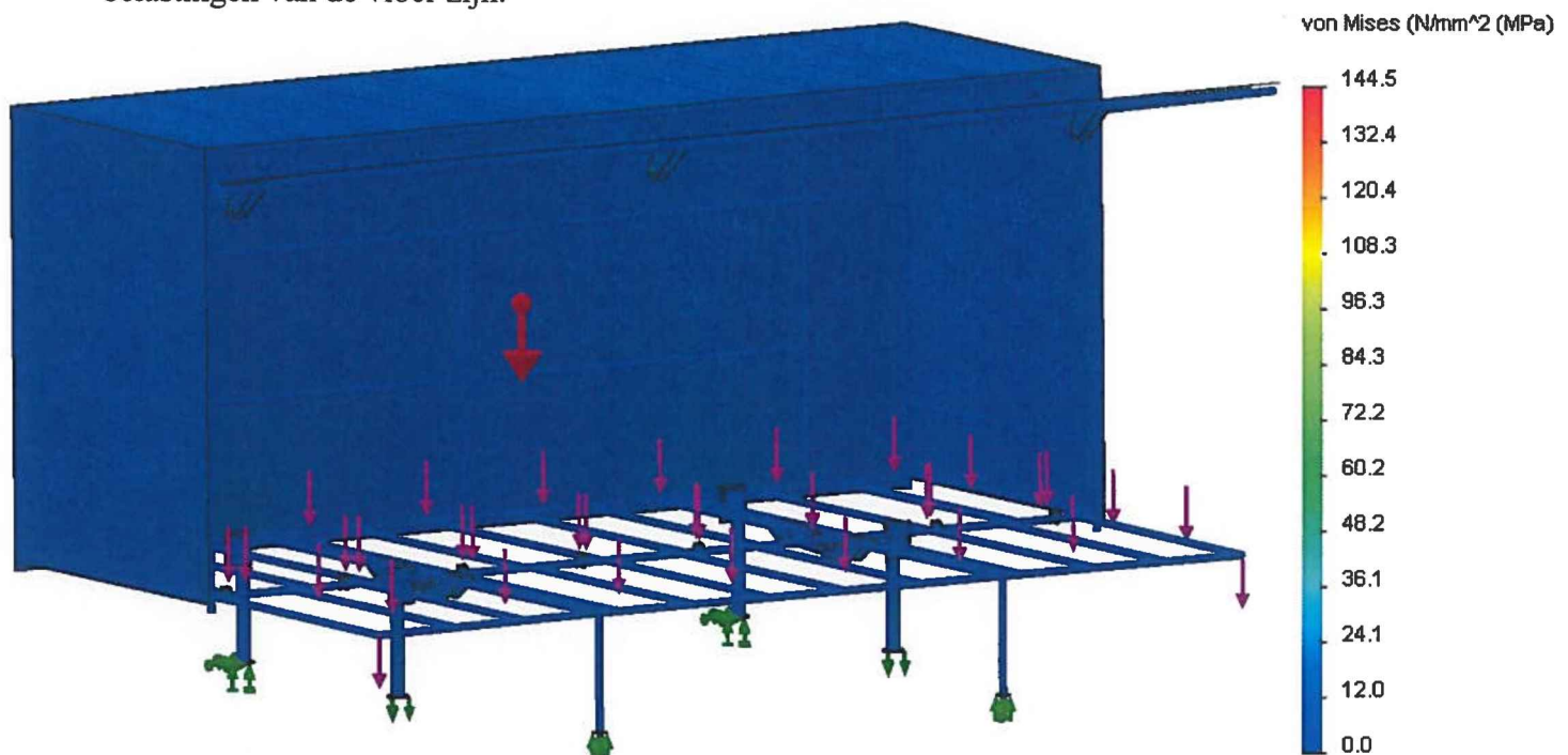
Figuur 19: Spanningen van de plaatdelen bij de vloerbelasting
