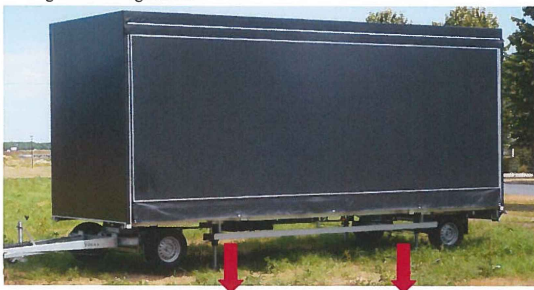
Figuur 6: Knop 2 afstandbediening is podiumwagen afstempelen
