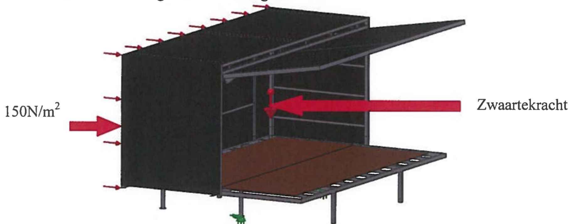
Figuur 16: Stabiliteit berekening podiumwagen
