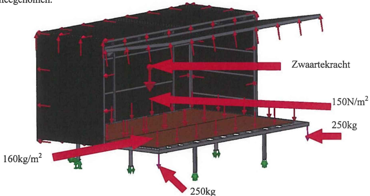
Figuur 22: Belasting voor sterkte berekening van de constructie van de podiumwagen
