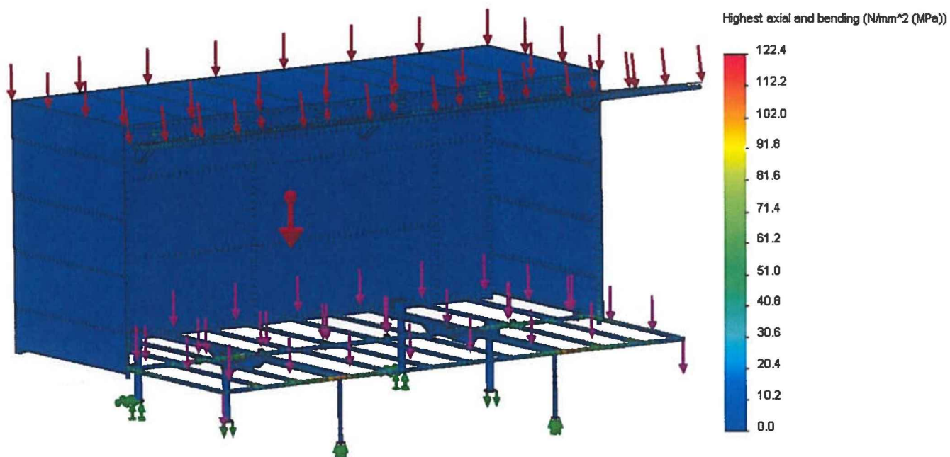
Figuur 27: Optredende spanning in de profielen van de podiumwagen bij sneeuw en vloerbelasting
