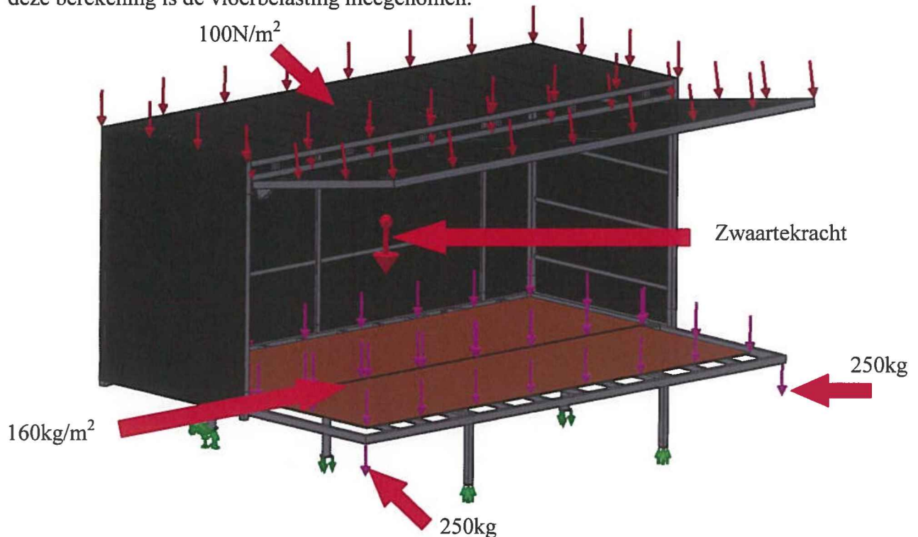
Figuur 25: Belasting voor sterkte berekening van de constructie van de podiumwagen
