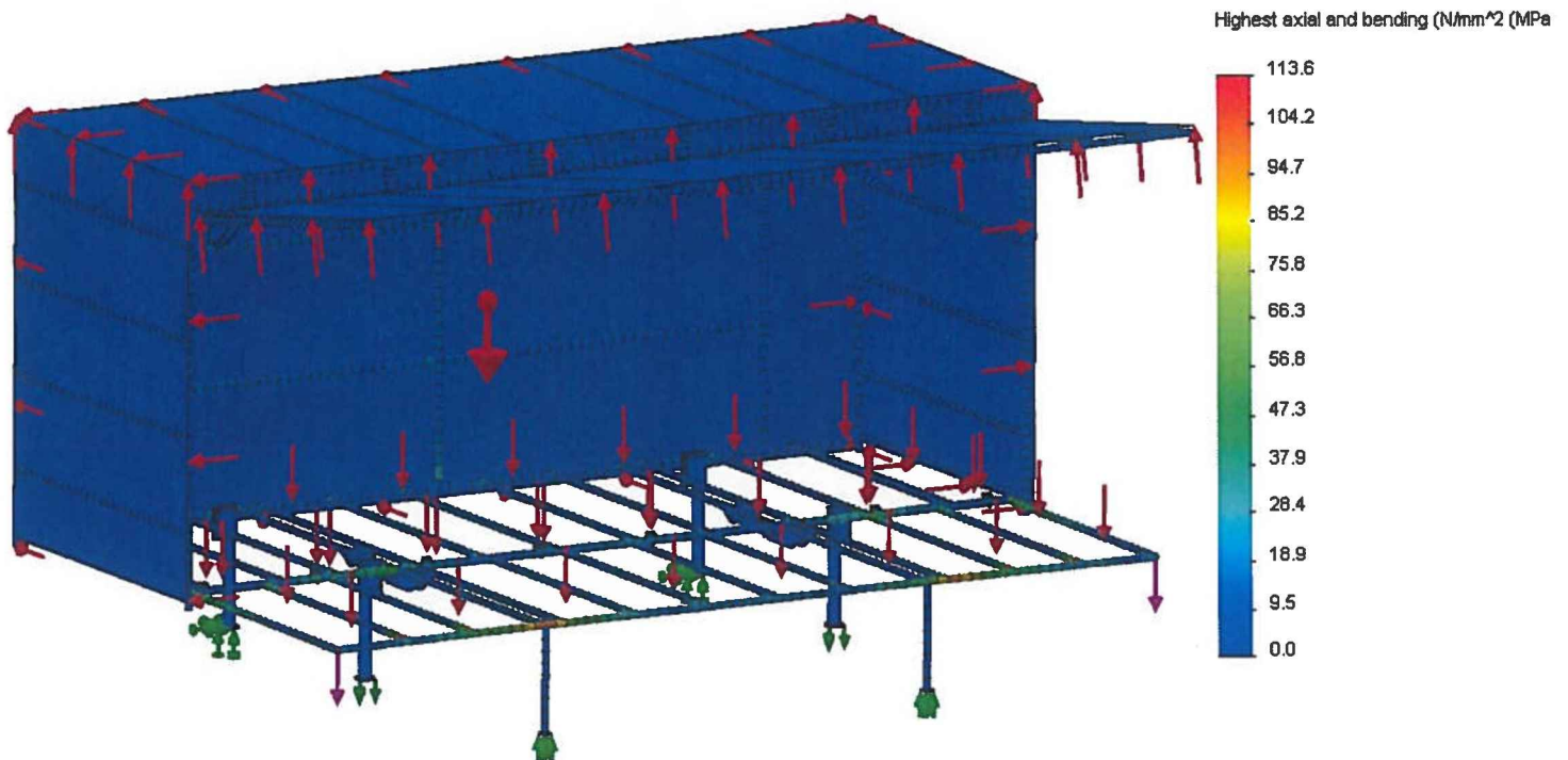
Figuur 24: Optredende spanning in de profielen van de podiumwagen bij deze belasting
