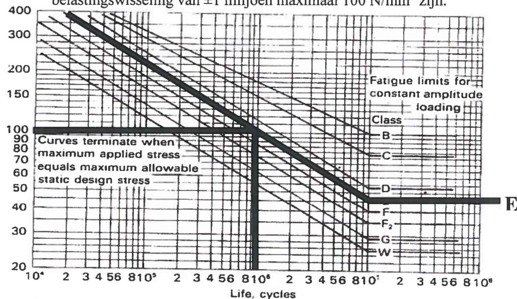
Figuur 15: Wöhlercurve voor maximaal toelaatbare lasspanning
