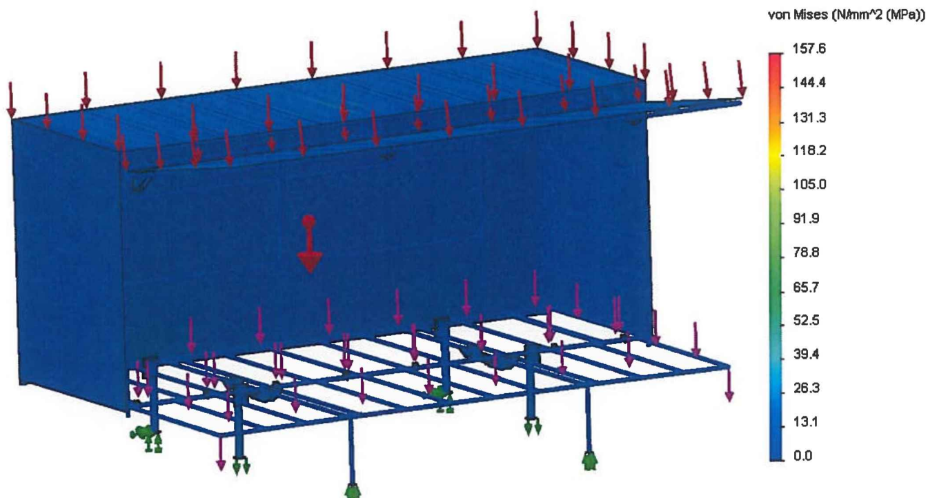
Figuur 26: Spanningen in de plaatdelen van de constructie bij sneeuw en vloerbelasting
