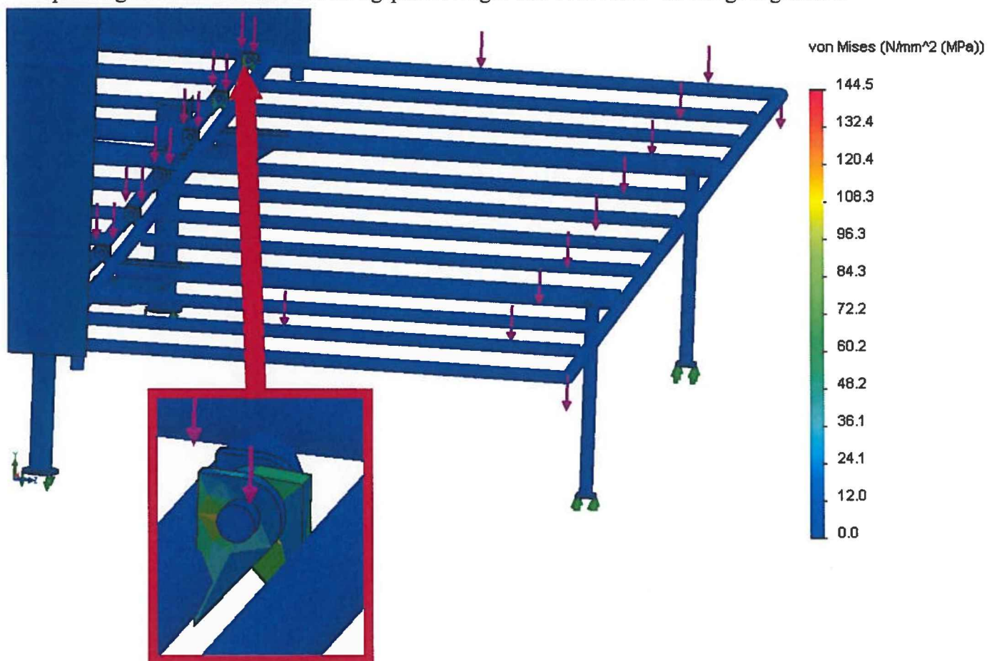
Figuur 20: Detail spanning van de verbinding tussen de vloeren
