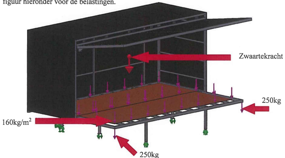
Figuur 18: Belasting voor sterkte berekening van de vloer van de podiumwagen
