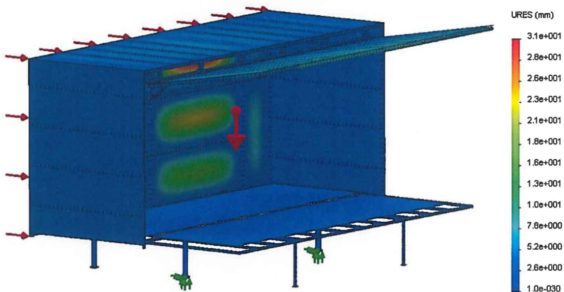
Figuur 17: Verplaatsing podiumwagen bij stabiliteit berekening
