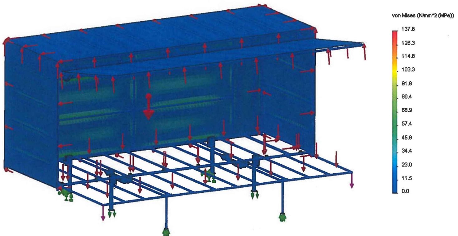
Figuur 23: Spanningen in de plaatdelen van de constructie bij deze wind en vloerbelasting
