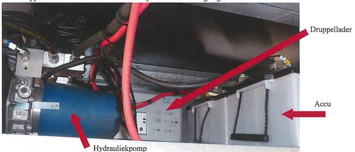
Figuur 2: Onderdelen voor aansturing hydraulisch systeem
