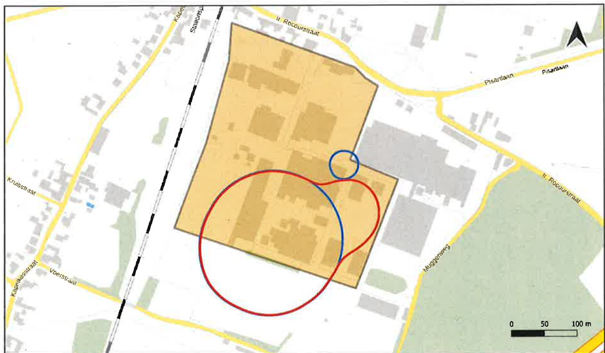
Figuur 1 Plaatsgebonden risico (PR 10-6) PQ Silicas B.V. Eijsden
